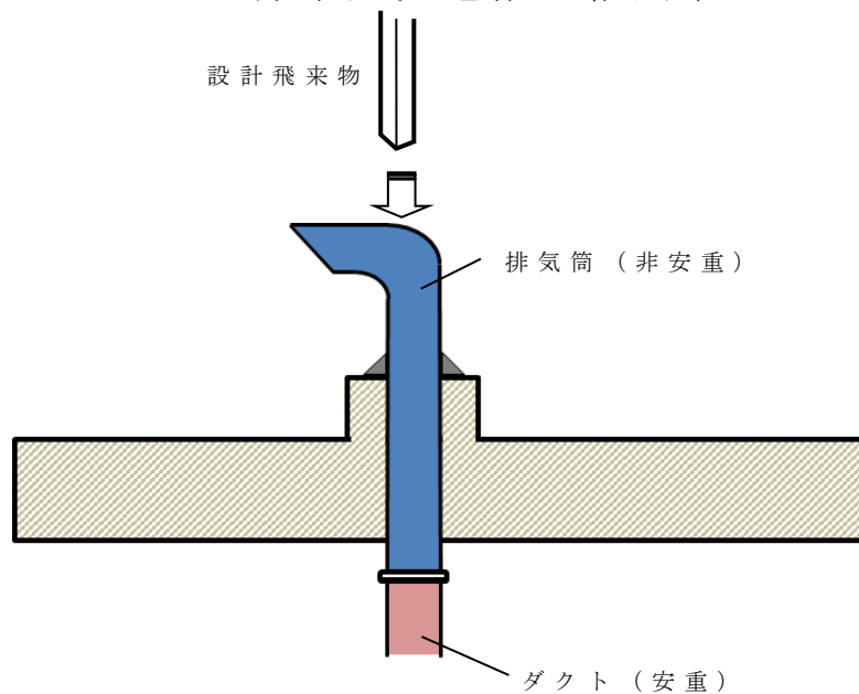
b . 非常用発電機の排気系
