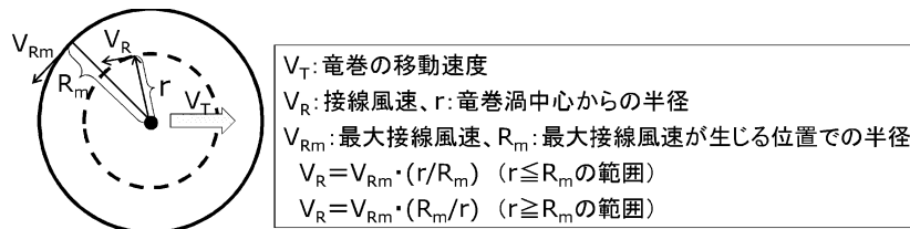
解説図 3.5 ランキン渦モデルの概要
