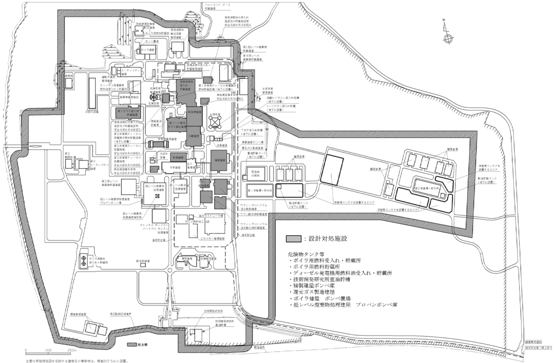
第 1.7.11-1 防火帯，設計対処施設等の配置図
