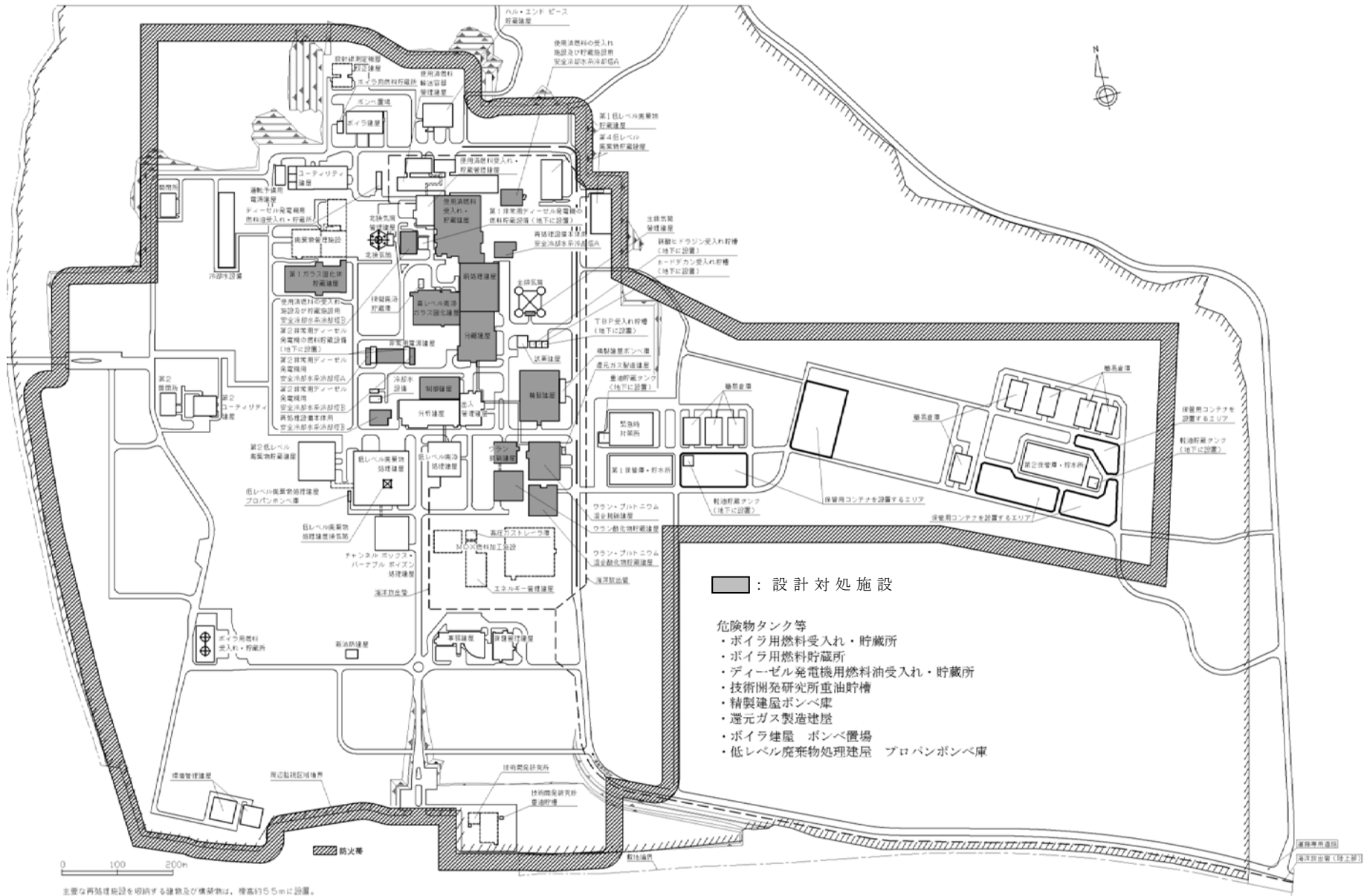
第 3 図 設計対処施設の配置図
