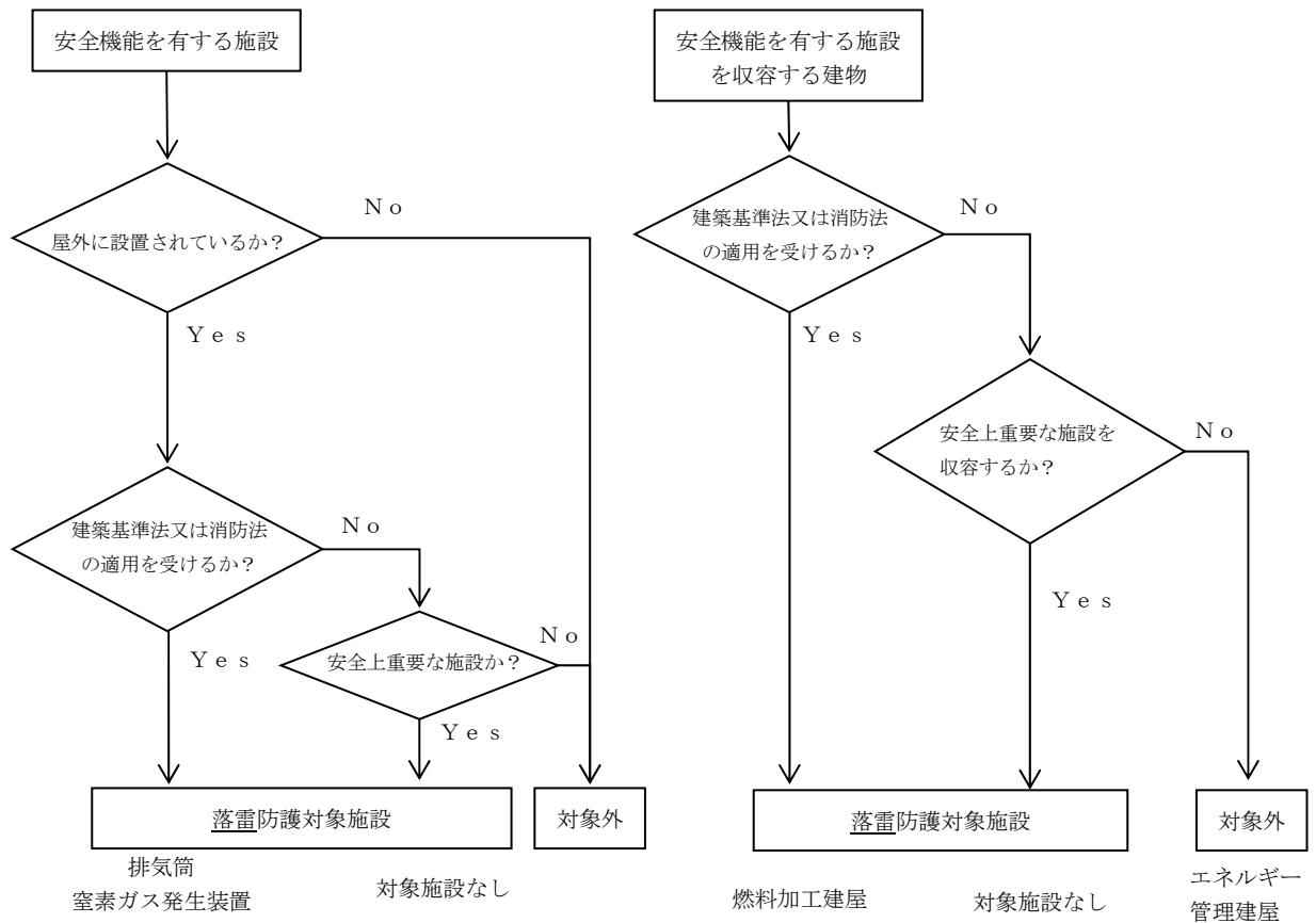
第4-1図 直撃雷に対する落雷防護対象施設の選定フロー
