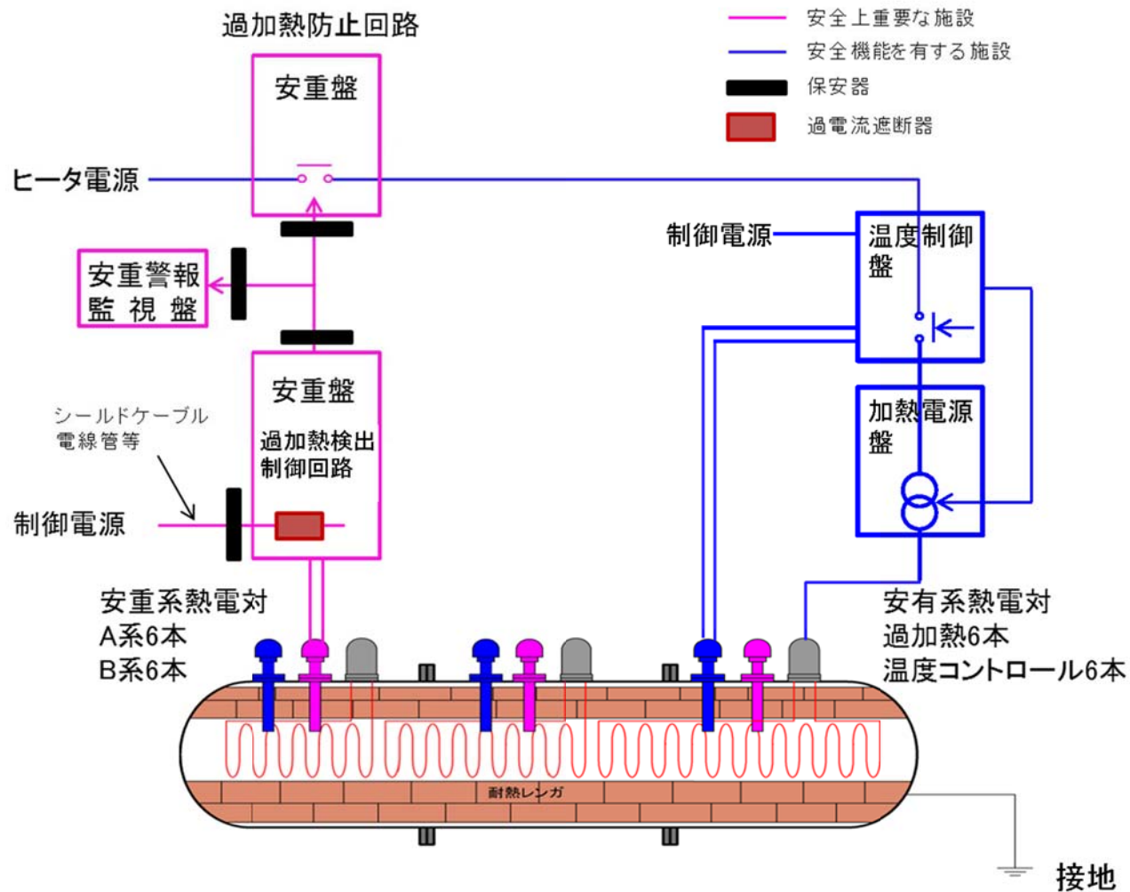
第 4 - 2 - 1 図 過加熱防止回路の対策イメージ
