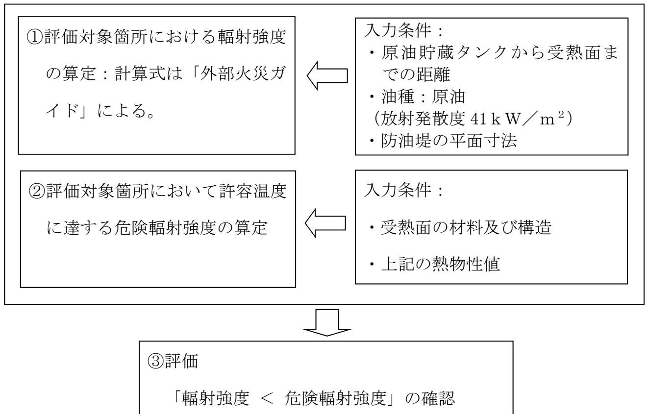
第1図 外部火災防護対象設備を収納する建屋に関する検討手順
