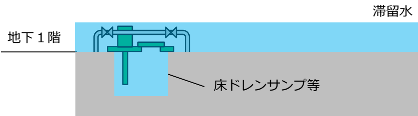
穿孔【断面図】
