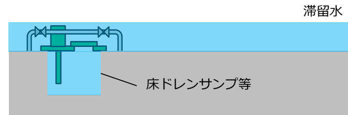
穿孔後【断面図】
