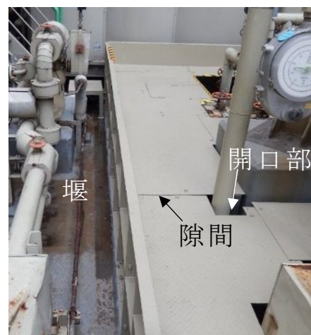
図1 高浜発電所 4号炉 タンク堰への覆い設置状況
