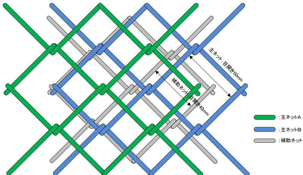
第1図 ネットの重ね合わせイメージ
