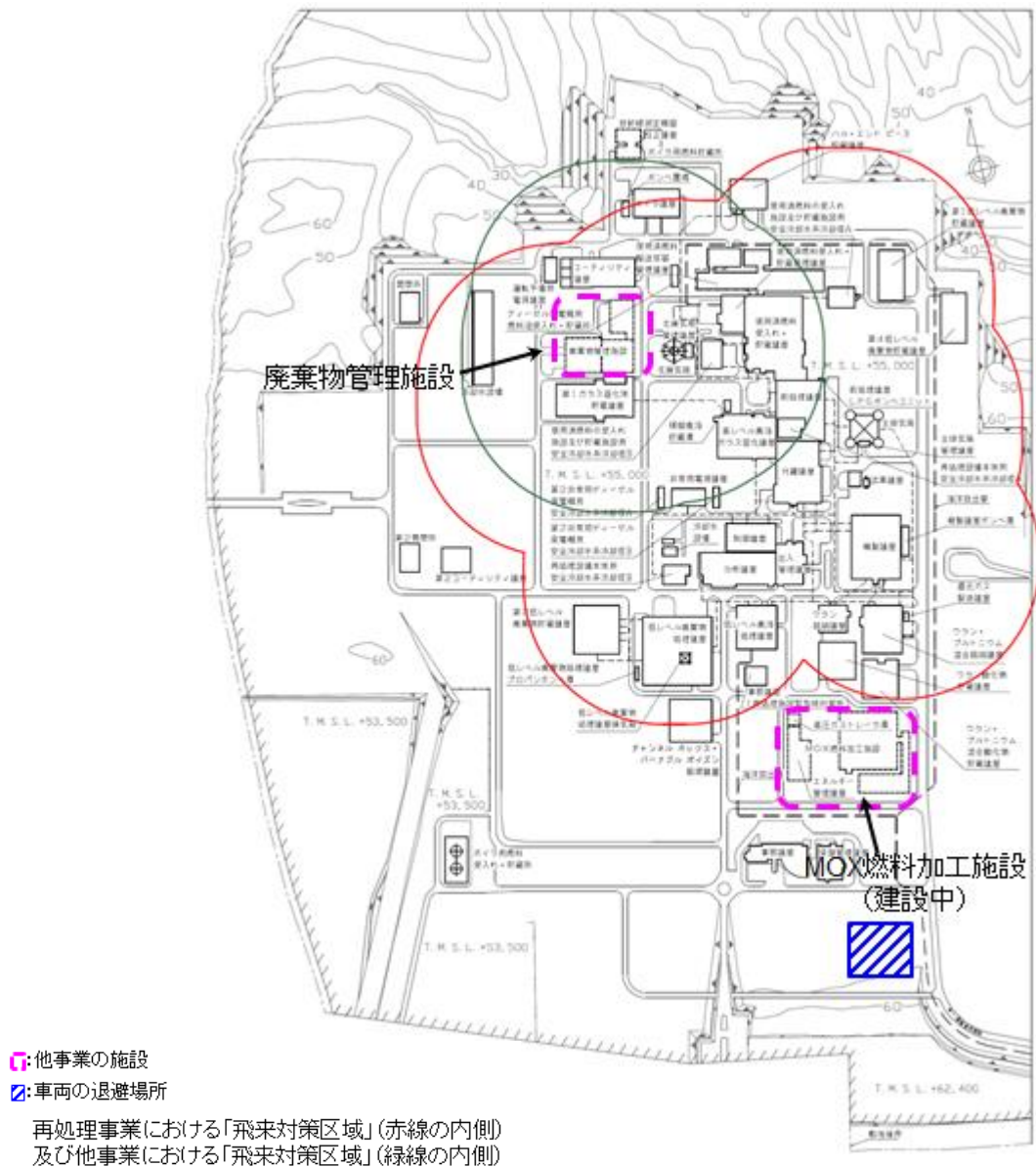
第10図 再処理事業及び他事業における飛来対策区域
