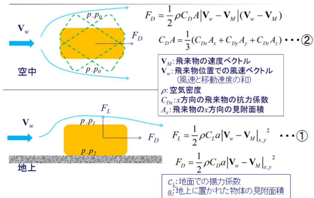
第5図 飛来物に作用する流体力 (3)
