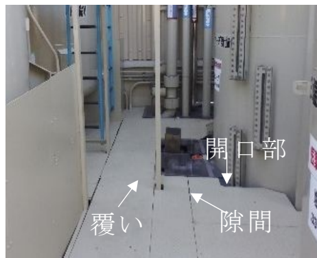
図 1 大飯発電所 4号炉 タンク堰への覆い設置状況
