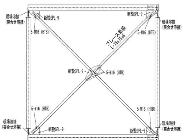
B部平面図 (当初設計)
