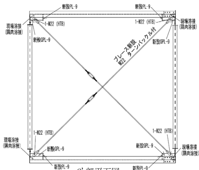
C'部平面図 (当初設計)
