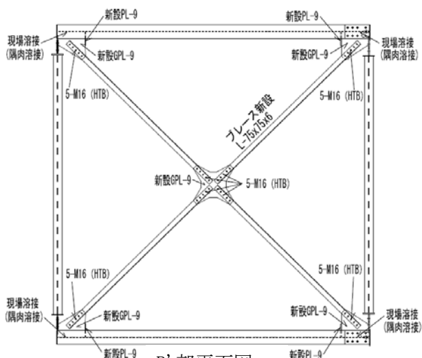
B'部平面図 (変更後)
