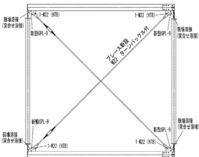
C部平面図 (当初設計)
