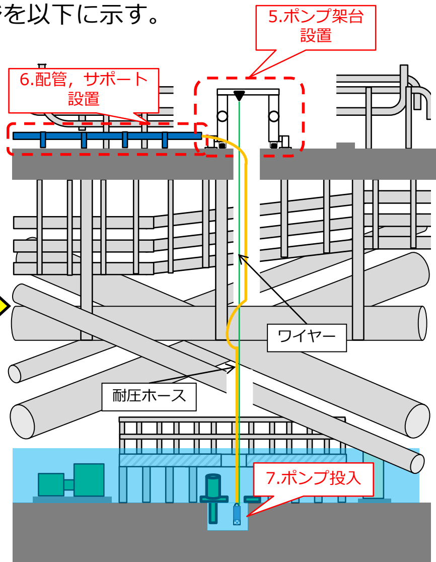
装置設置【断面図】
