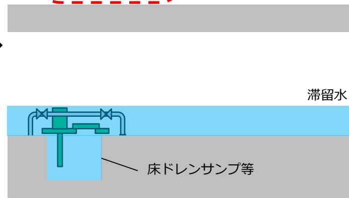
干渉物撤去後【断面図】
