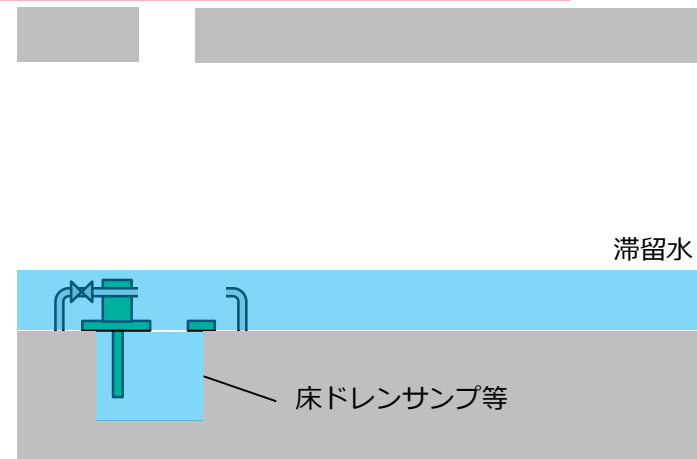
点検用マンホール撤去後【断面図】
