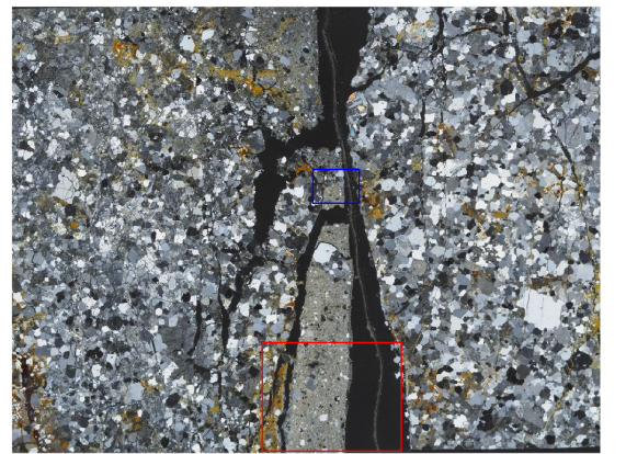
直交ニコル
