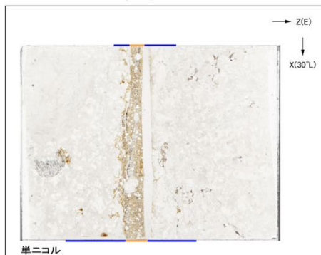
断層面の条線観察結果
