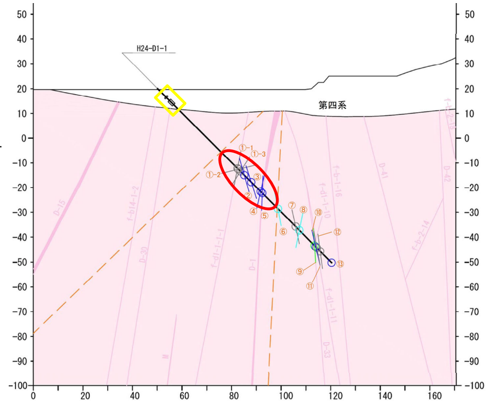
H24-D1-1孔沿いの断面図 赤枠は鉱物脈法の対象とした破碎部を示す。
