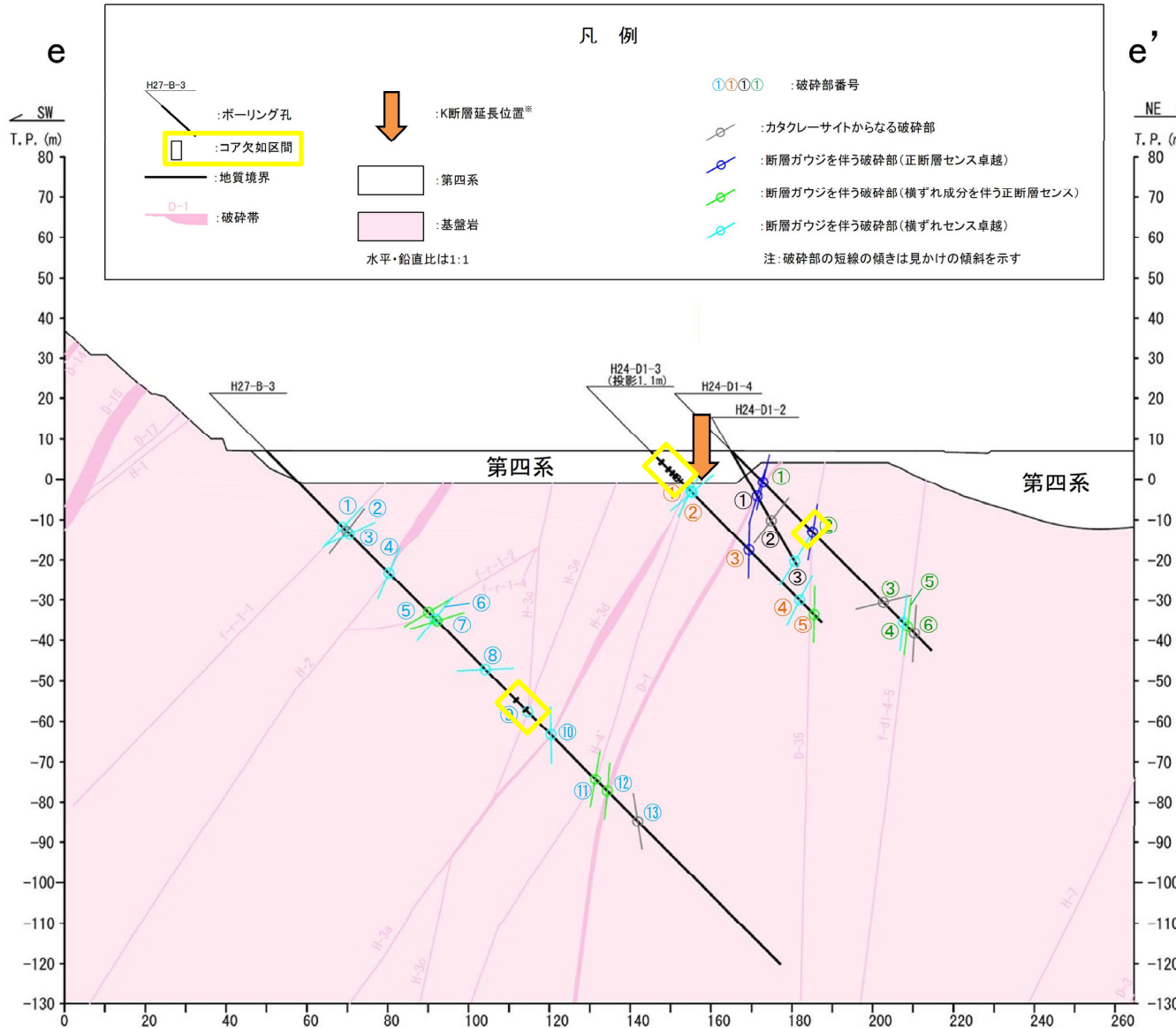
H27-B-3孔, H24-D1-3孔, H24-D1-2孔及びH24-D1-4孔沿いの地質断面図(e-e' 断面)
