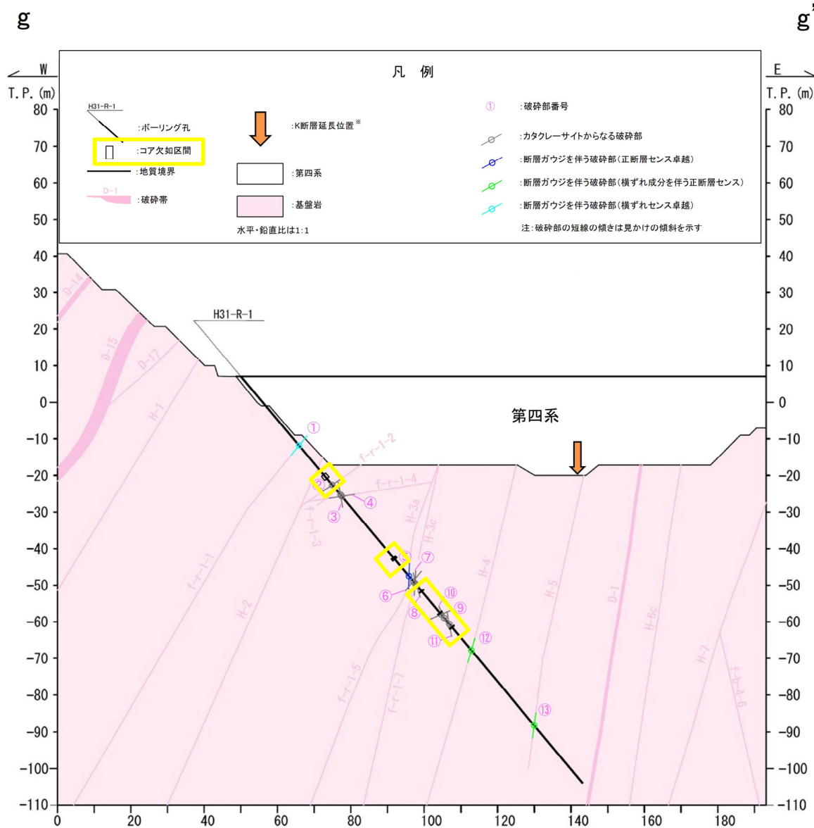
H31-R-1孔沿いの地質断面図(g-g'断面)
