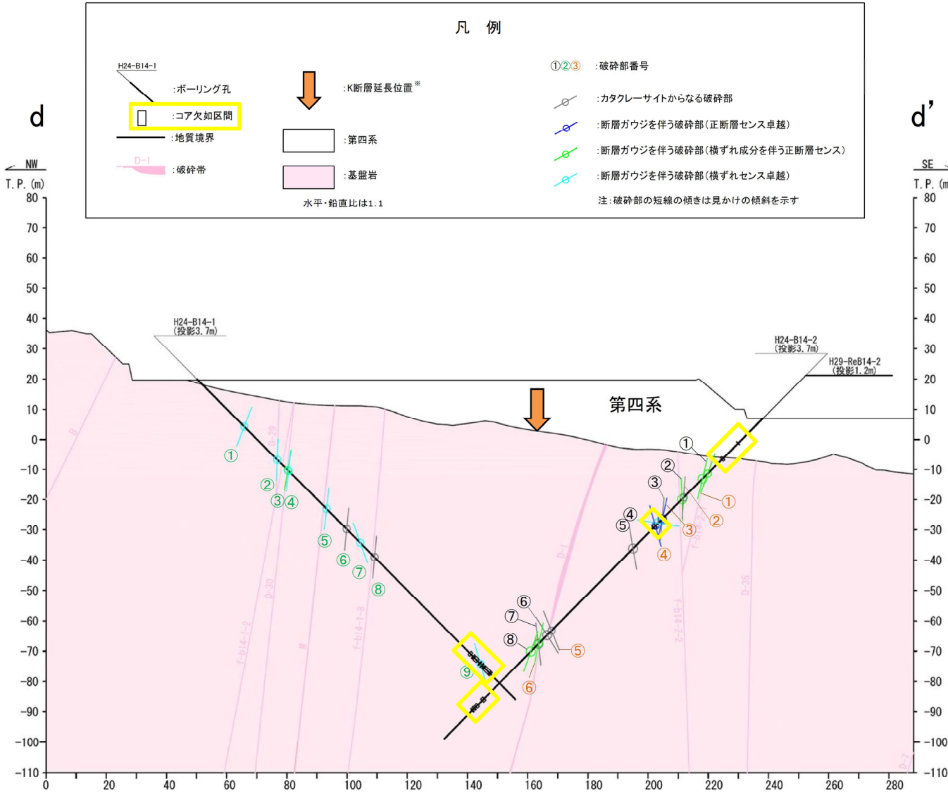
H24-B14-1孔, H24-B14-2孔, H29-ReB14-2孔沿いの地質断面図(d-d'断面)
