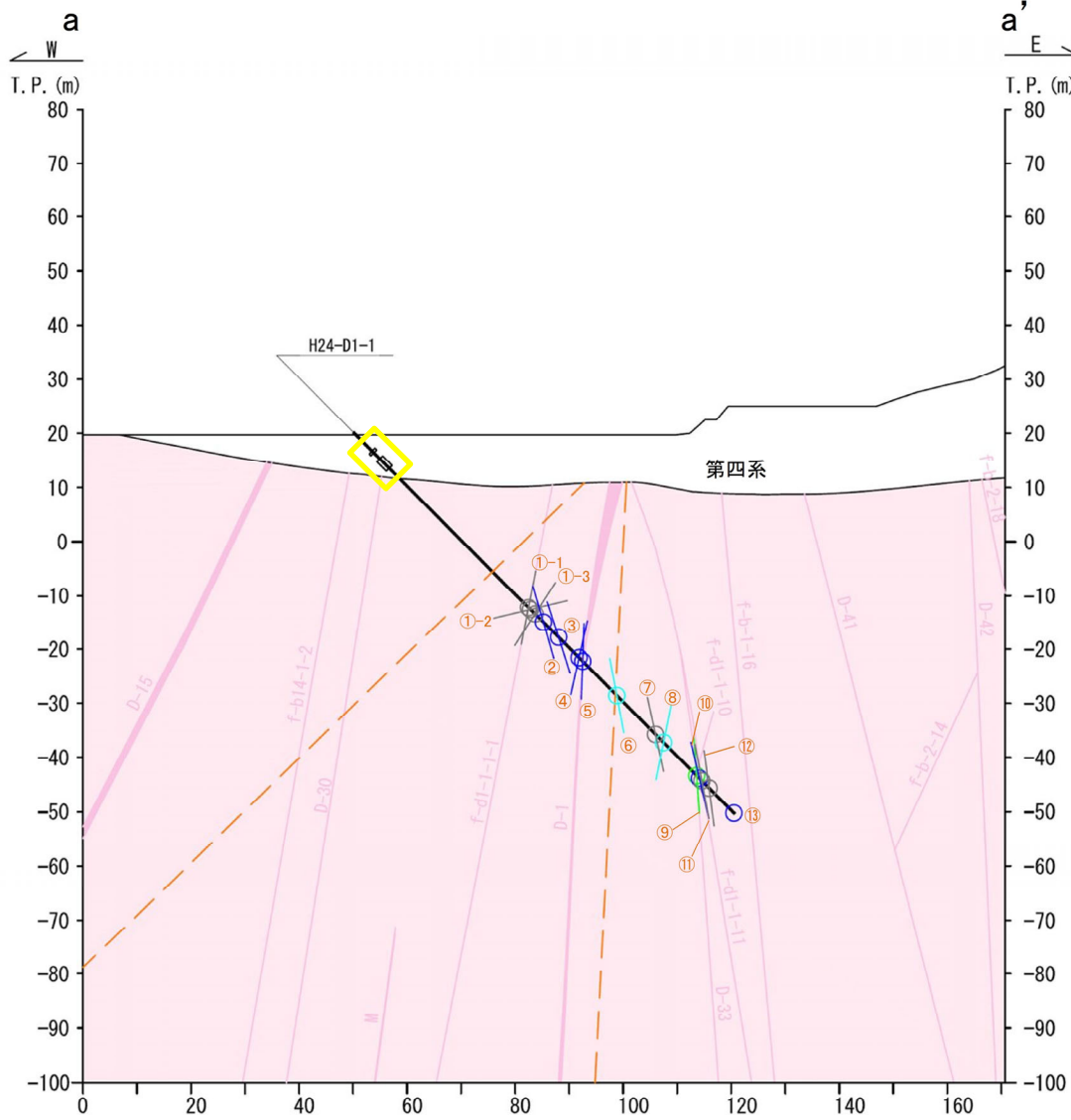
H24-D1-1孔沿いの地質断面図 (a-a' 断面)
