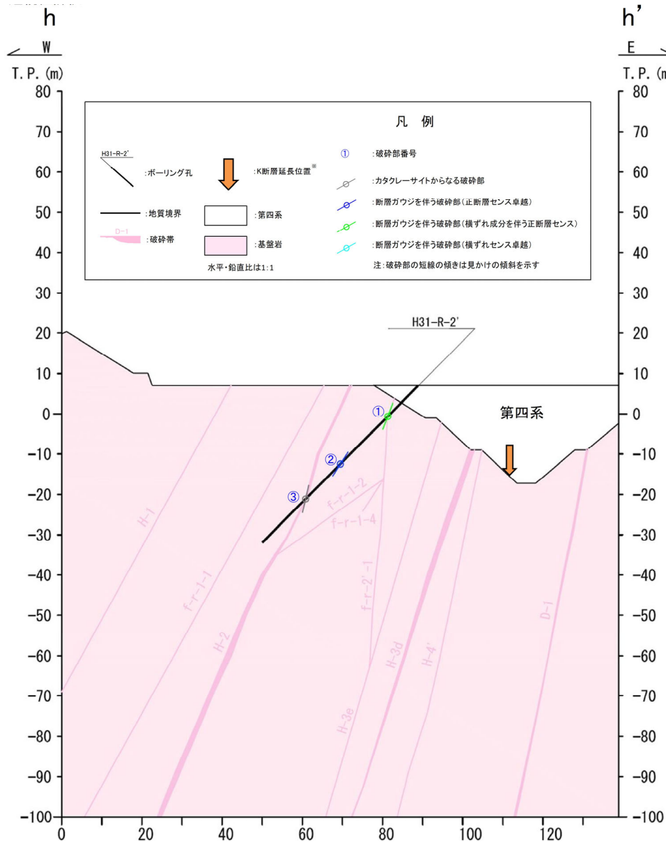
H31-R-2' 孔沿いの地質断面図(h-h' 断面)
