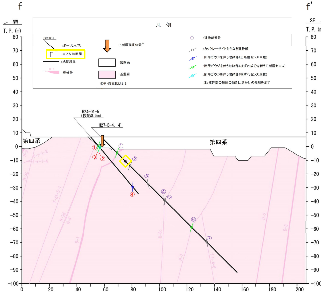
H24-D1-5孔, H27-B-4孔沿いの地質断面図(f-f' 断面)
