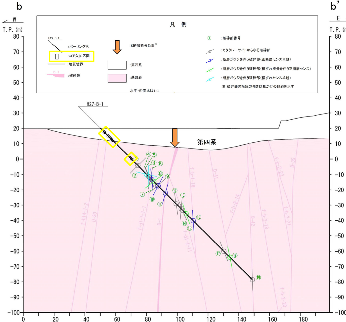
H27-B-1孔沿いの地質断面図(b-b'断面)
