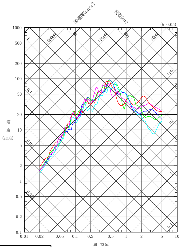
NS成分
