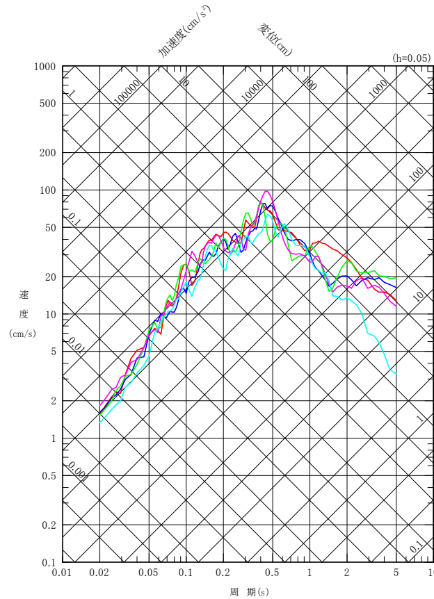
EW成分
