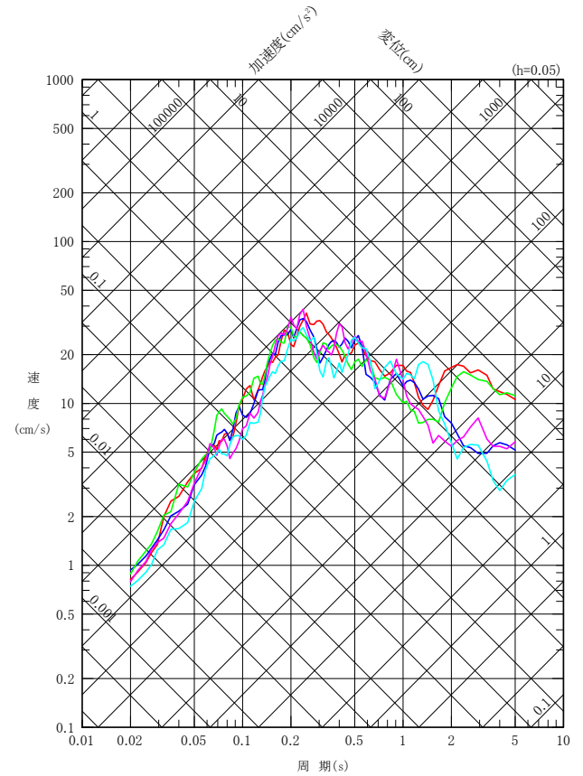
UD成分
