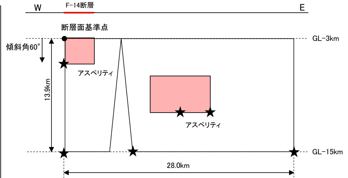
(b) 展開図
