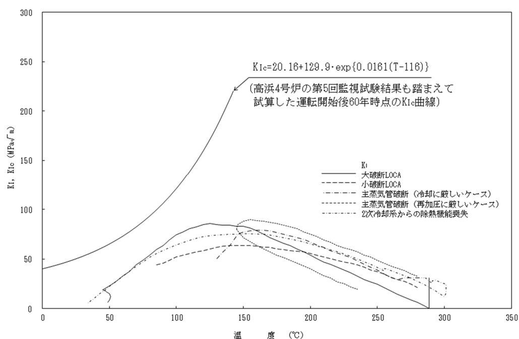
図10-4 高浜4号炉 第5回監視試験で得られた破壊靱性実測値を踏まえたPTS評価
