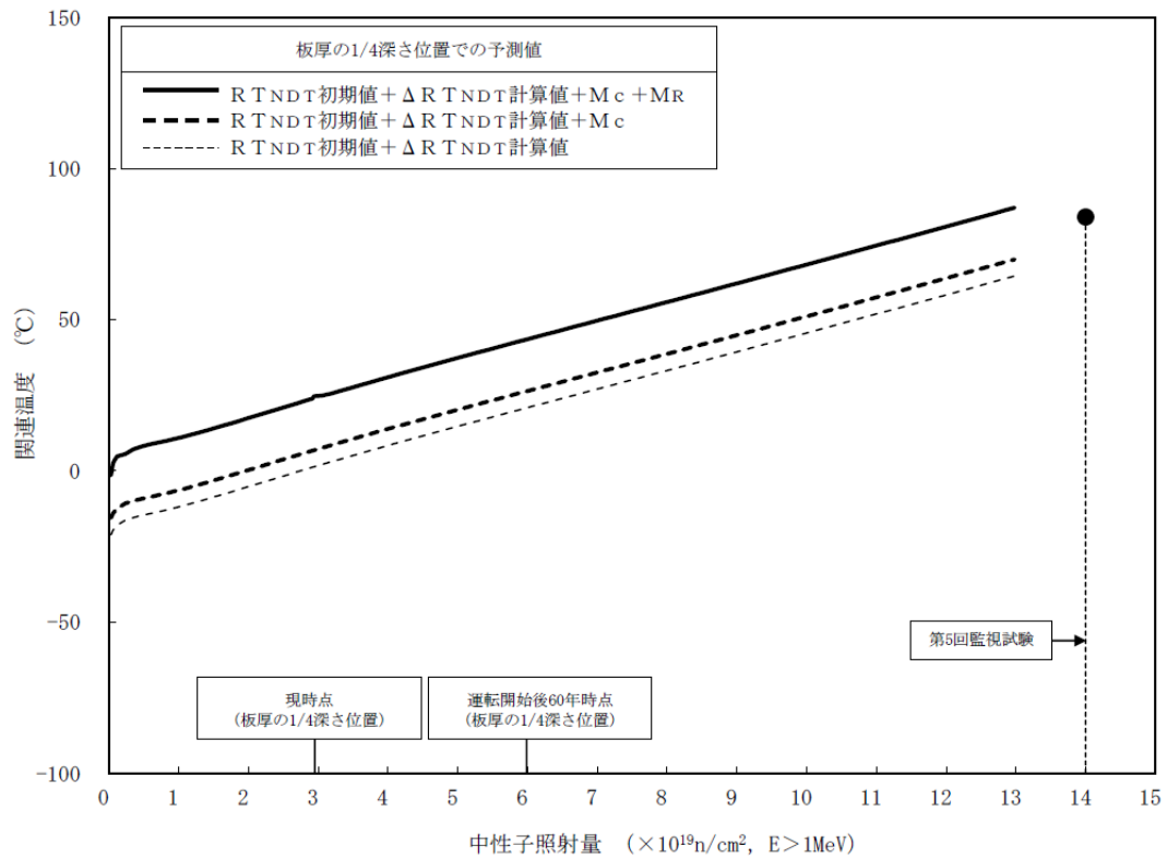
図 10-1 第 5 回監視試験で得られた関連温度実測値（母材）に対する分析結果
