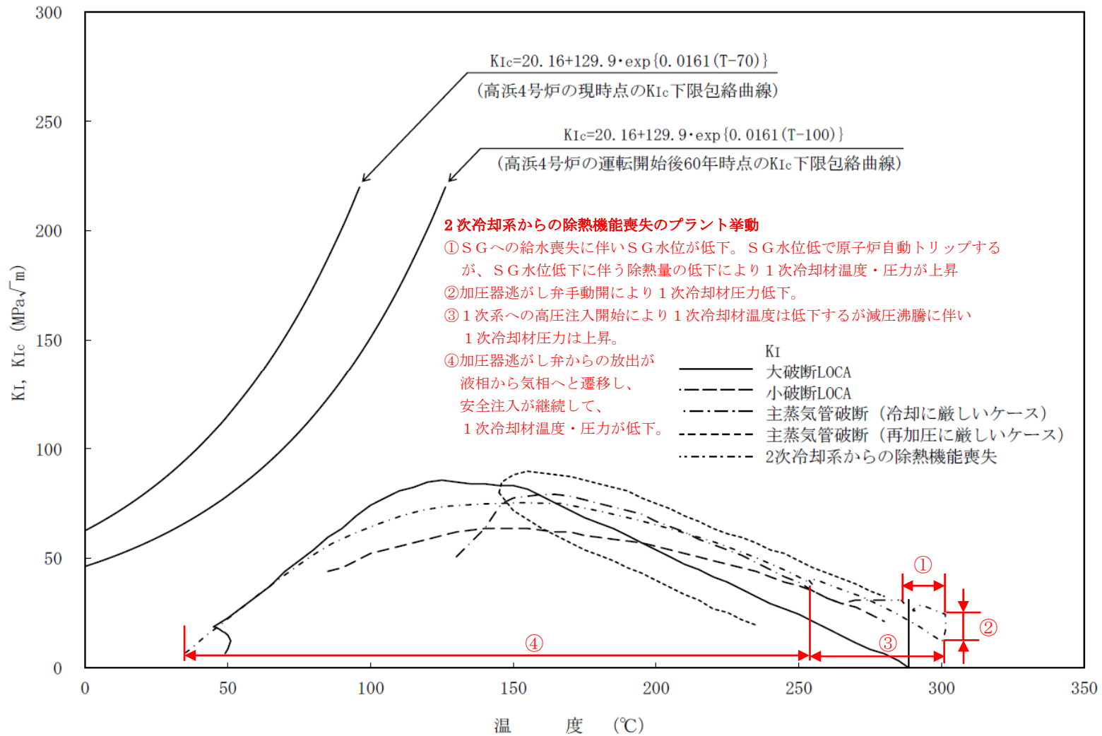
高浜4号炉 原子炉容器胴部（炉心領域部）中性子照射脆化に対するPTS評価結果
