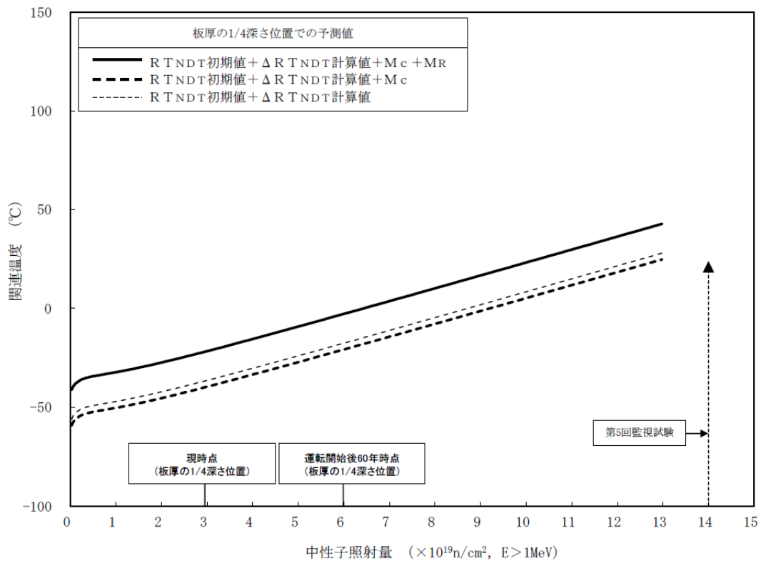
図 10-2 第 5 回監視試験で得られた関連温度実測値（溶接金属）に対する分析結果
