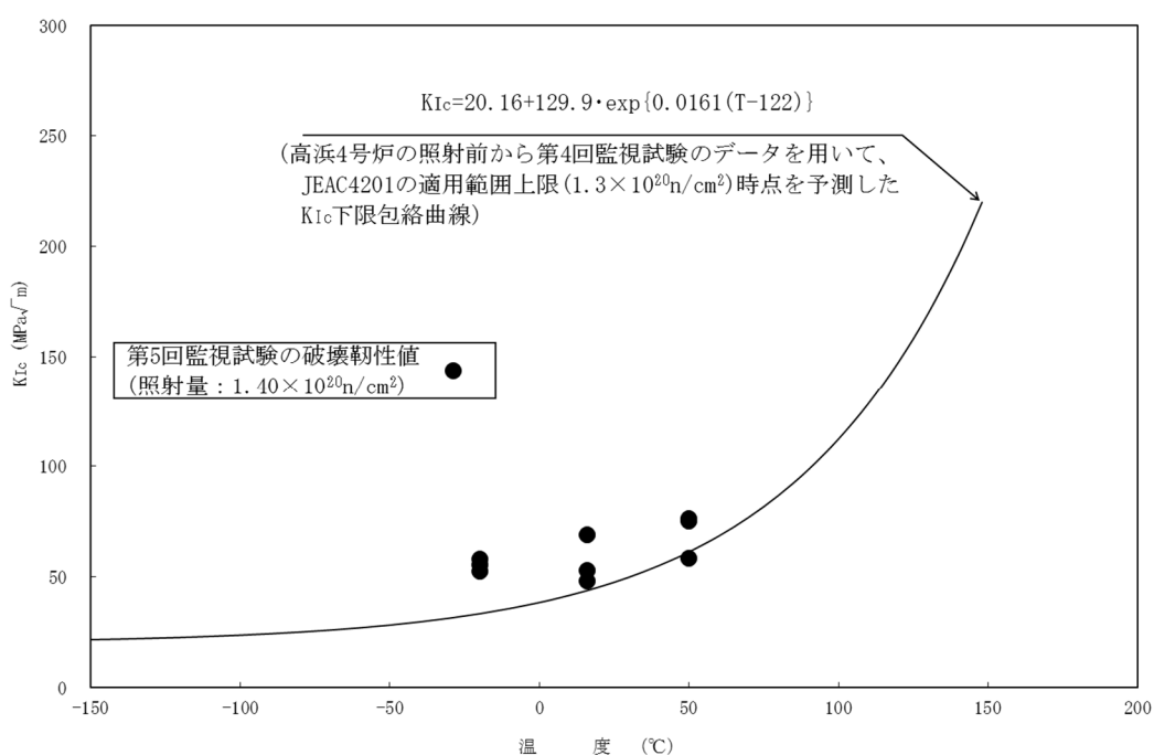
図 10-3 高浜 4 号炉 第 5 回監視試験で得られた破壊靱性実測値に対する分析結果
