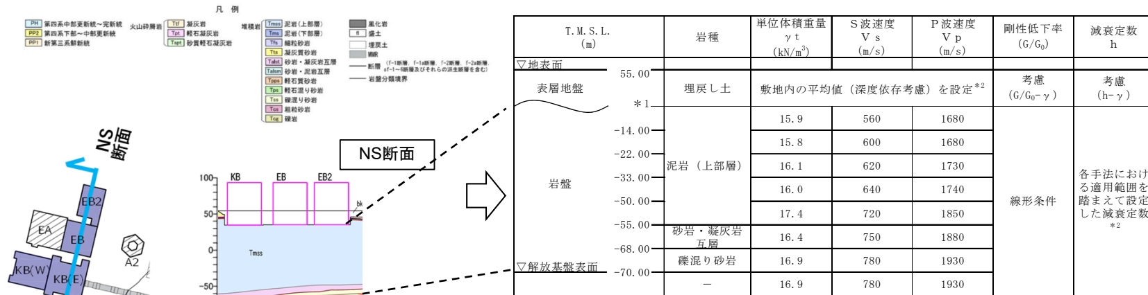
西側①エリアの地下構造
