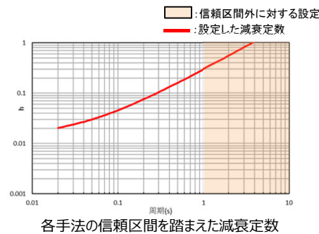
岩盤部分の減衰定数
