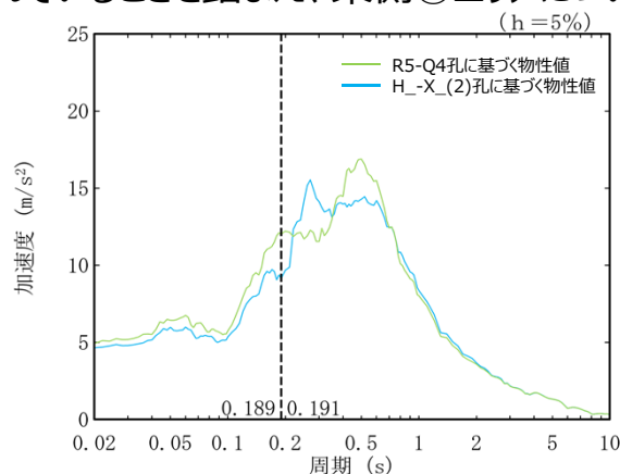
応答スペクトルの比較（G14、Ss-A）
