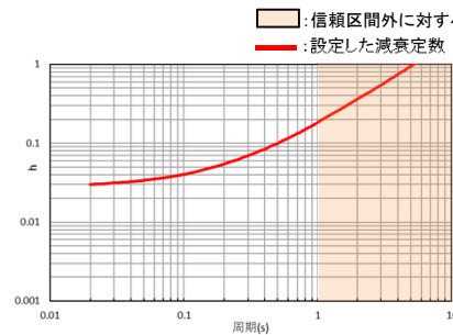
各手法の信頼区間を踏まえた減衰定数
