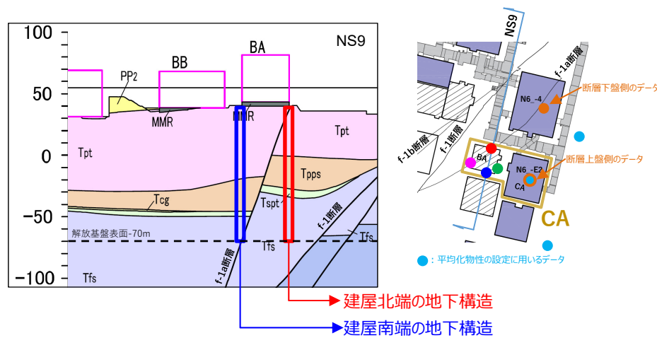
BA直下に存在する断層による地下構造の不連続性（南北断面の例）
