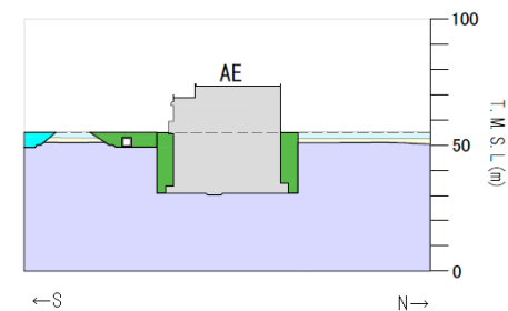
NS断面
