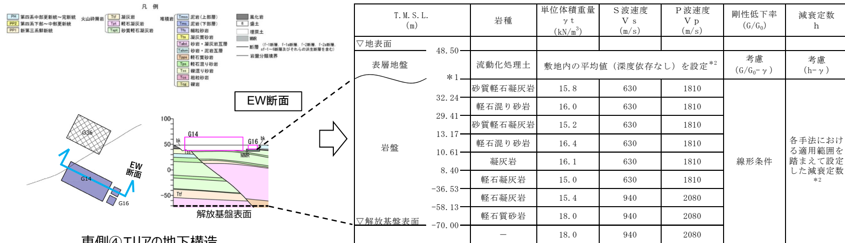
東側④エリアの地下構造
