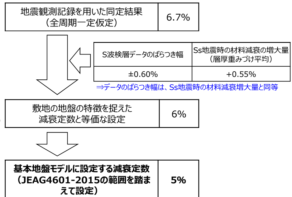
本エリアにおける基本地盤モデルに設定する減衰定数の考え方
