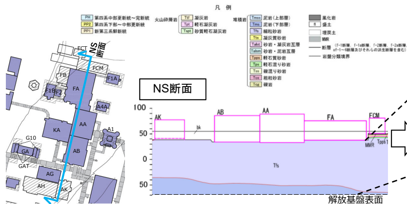
中央①エリアの地下構造
