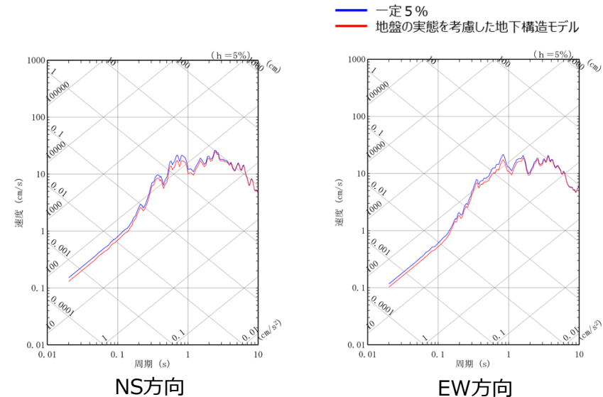
敷地の地盤の特徴を捉えた地下構造と周波数一定の設定（5%）の地盤応答比較（201103111446地震，東側③エリア）
