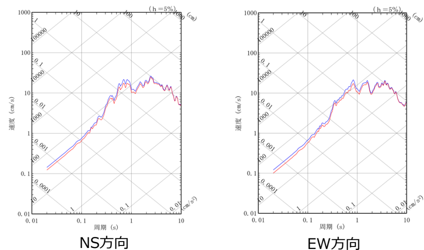
敷地の地盤の特徴を捉えた地下構造と周波数一定の設定（5%）の地盤応答比較（201103111446地震，東側②エリア）
