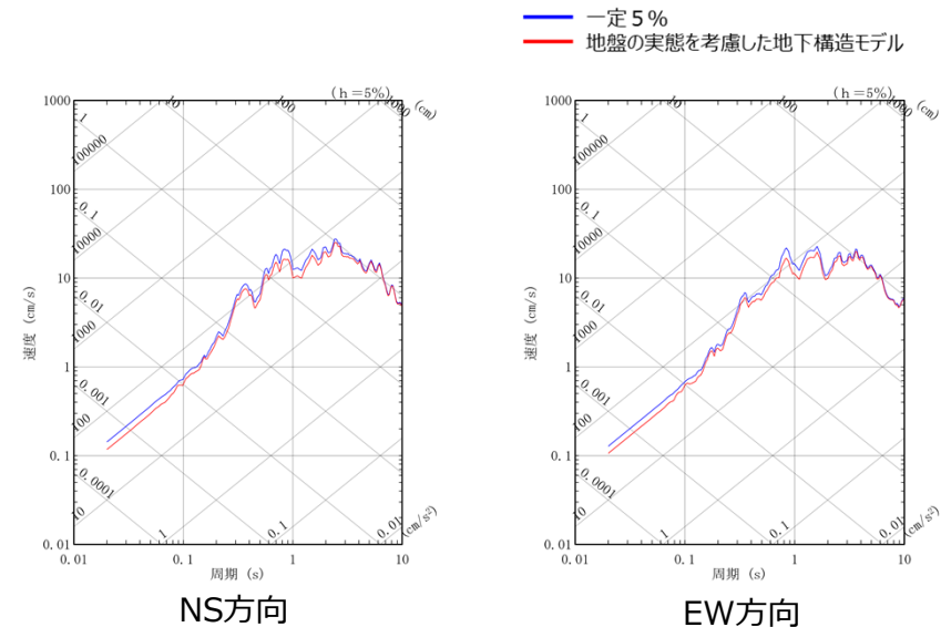
敷地の地盤の特徴を捉えた地下構造と周波数一定の設定（5%）の地盤応答比較（201103111446地震，東側⑤エリア）
