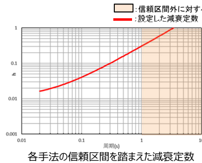
岩盤部分の減衰定数
