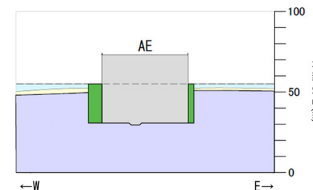
AEグループにおける断面図
