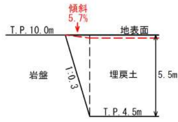
図7-17 想定される最大傾斜 (図7-13 No. 1)
