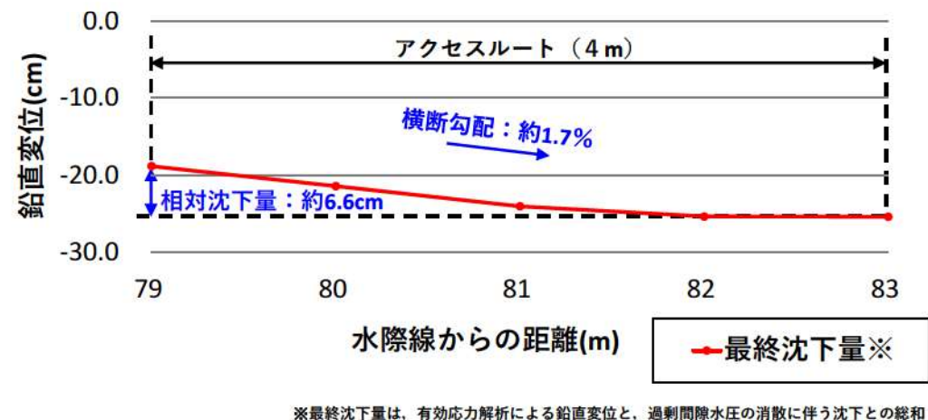
図7-27 側方流動を考慮した地表面変位評価結果 (アクセスルート)
