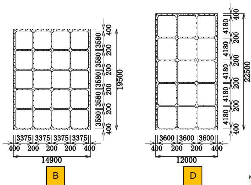
添付 7-18 図 放水池ケーソン部 (平面図)
