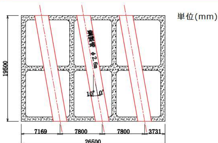
添付 7-19 図 放水口（縦断面図及び平面図）
