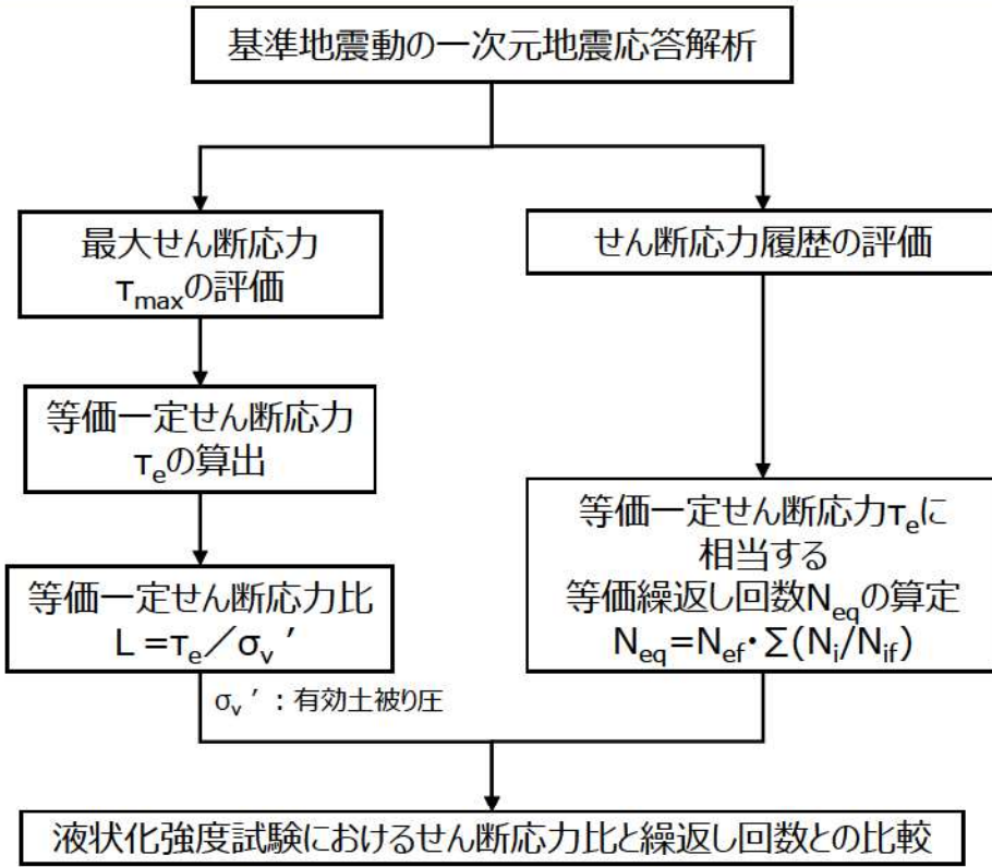
累積損傷度理論に基づく等価繰返し回数の評価フロー
