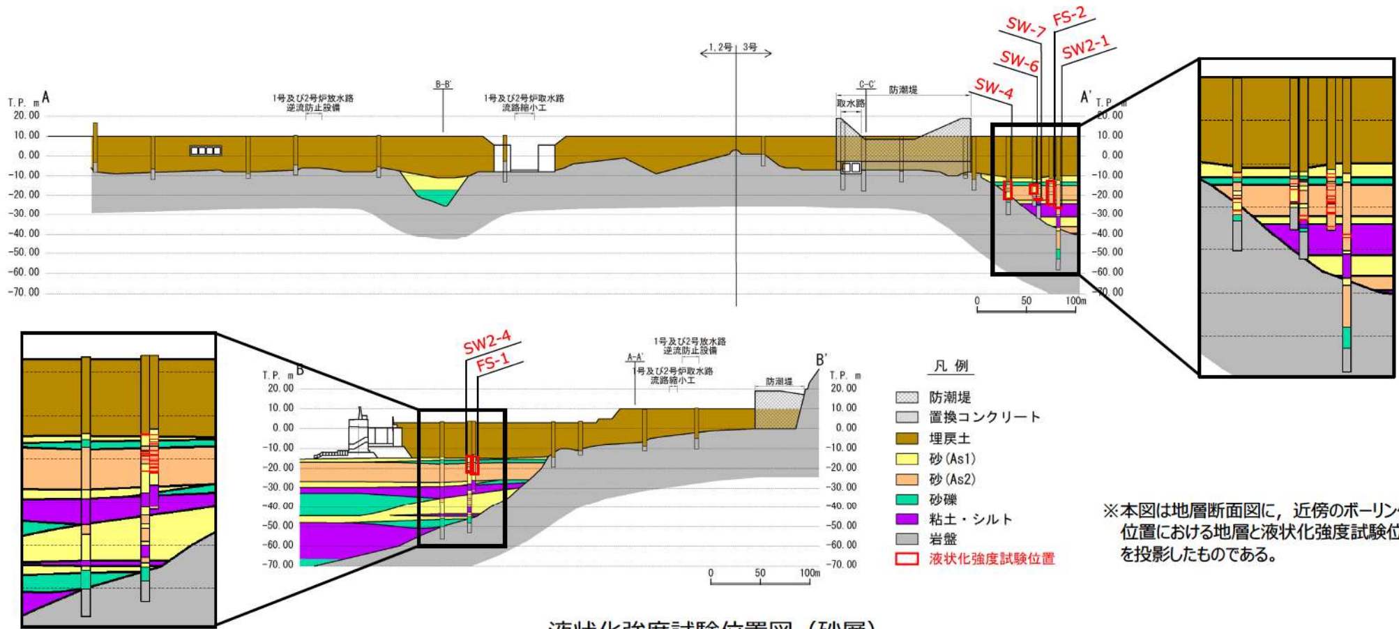
液状化強度試験位置図 (砂層)
