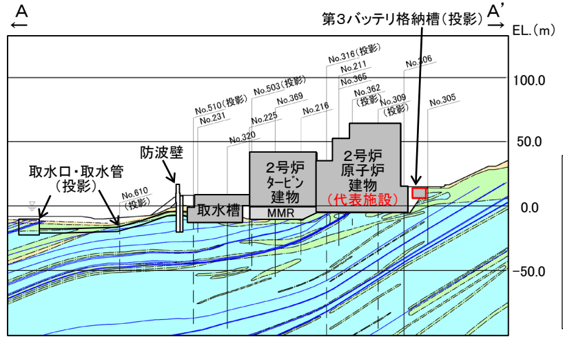
地質断面図 (A-A'断面, 岩級・シーム)
