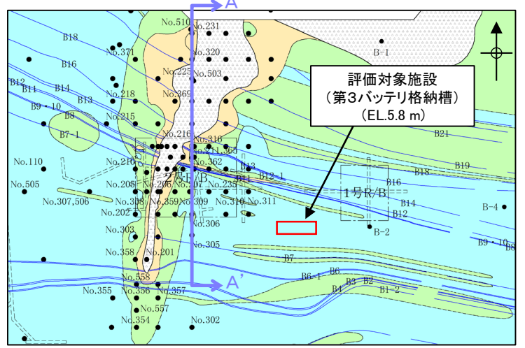
水平岩盤分類図 (評価対象施設設置位置付近 (岩級区分))
