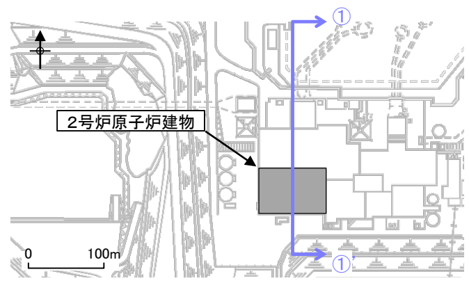
断面位置図
