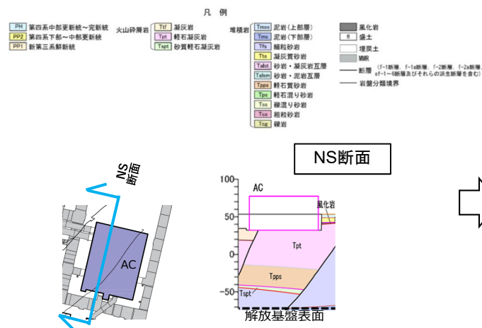
東側①エリアの地下構造
