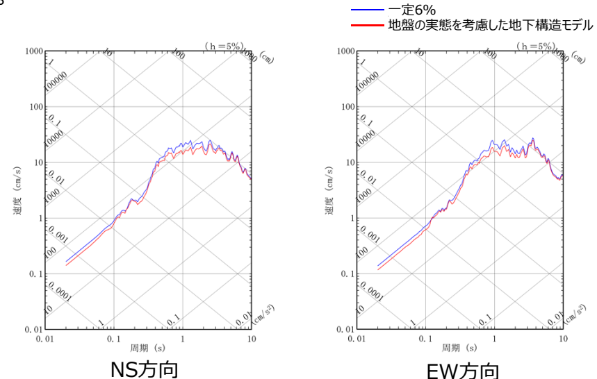
敷地の地盤の特徴を捉えた地下構造と周波数一定の設定（6%）の地盤応答比較（201103111446地震、西側①エリア）
