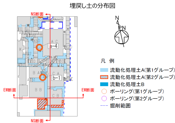
CBグループにおける表層分布図
