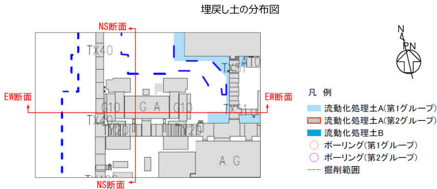
GAグループにおける表層分布図
