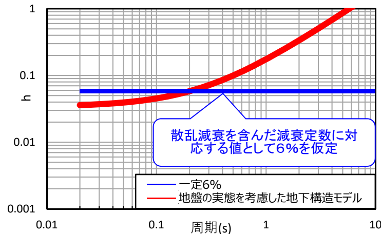
敷地の地盤の特徴を捉えた地下構造と仮定した値（6%一定）の比較（東側③エリア）
