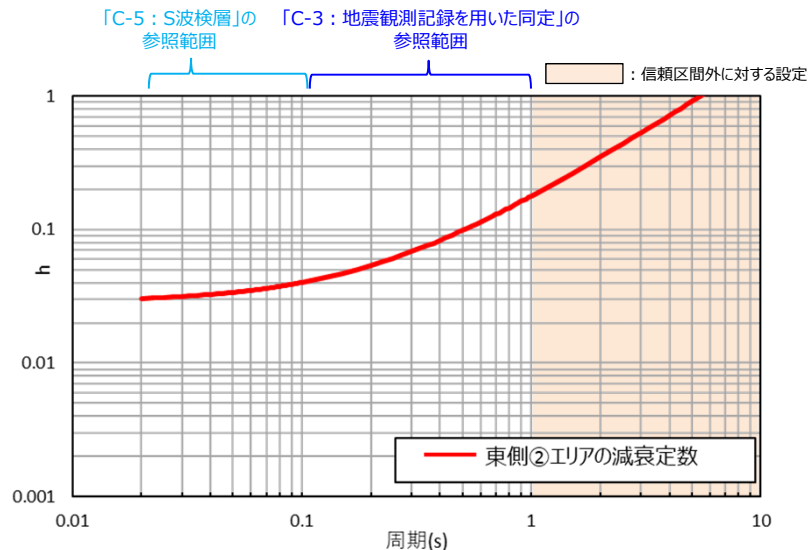
本エリアで仮定した減衰定数
