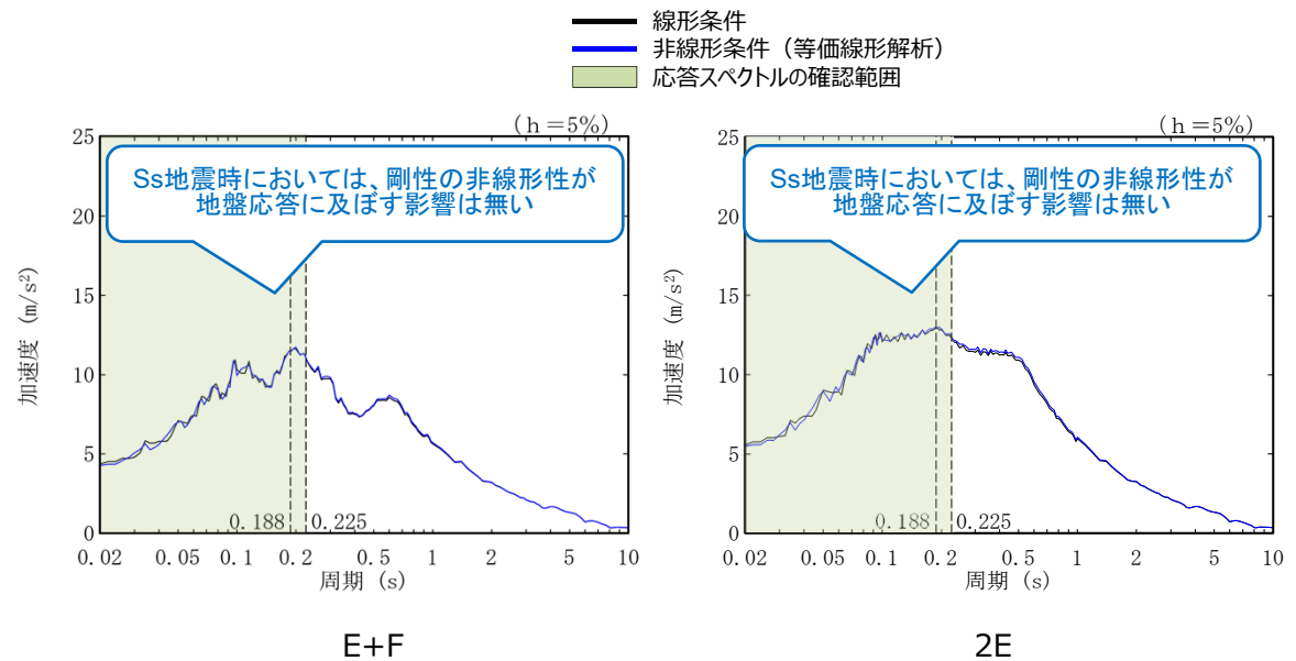
線形条件及び非線形条件における基礎底面レベルの入力地震動の比較 (AG)
