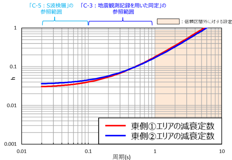
本エリアで仮定した減衰定数と 検証を行った減衰定数（東側②エリア）の比較
