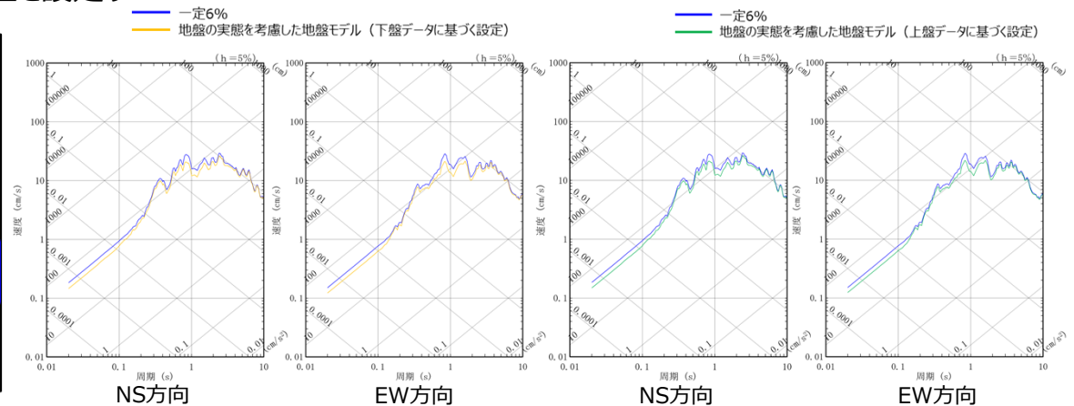
敷地の地盤の特徴を捉えた地下構造と周波数一定の設定（6%）の地盤応答比較（201103111446地震，東側⑥エリア）
