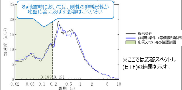
B: 岩盤部分の剛性の非線形性
