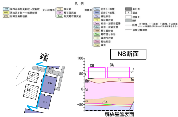
東側②エリアの地下構造
