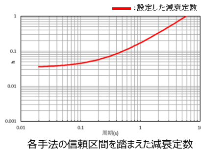
岩盤部分の減衰定数
