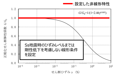
ひずみ依存特性 ( G/G_0 - \gamma 関係) (砂質軽石凝灰岩の例)
