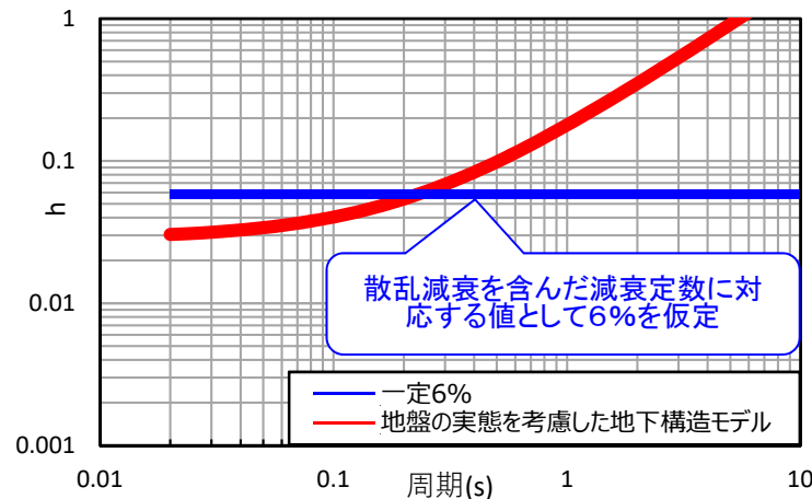
敷地の地盤の特徴を捉えた地下構造と仮定した値（6%一定）の比較（東側①エリア）
