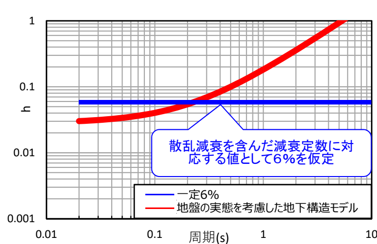
敷地の地盤の特徴を捉えた地下構造と仮定した値（6%一定）の比較（東側⑤エリア）
