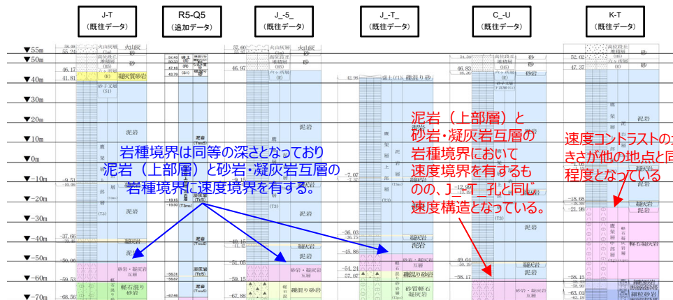
地質柱状図の比較 (グループ内の東西方向の順に整理)
