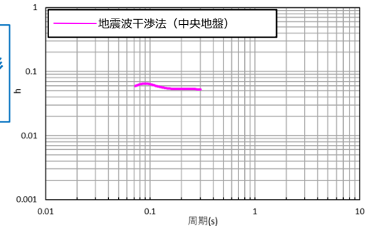
減衰定数の推定結果（中央地盤）
