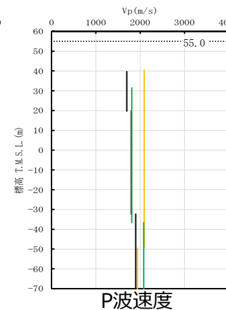
PS検層結果
