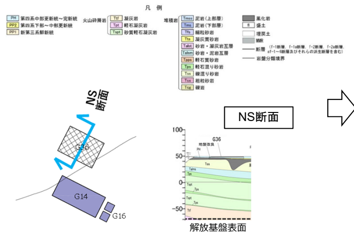
東側⑤エリアの地下構造
