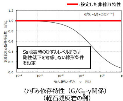
岩盤部分の剛性の非線形性
