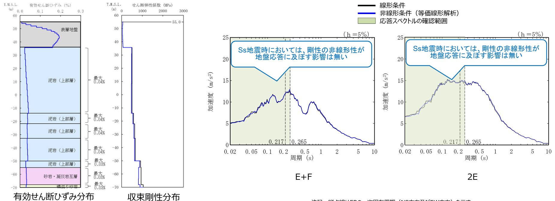
地盤の等価線形解析結果 (EB)
