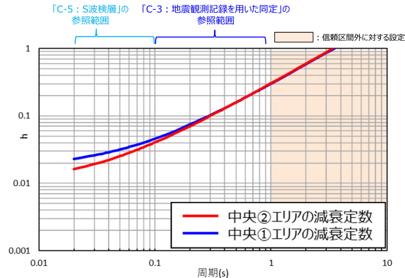
本エリアで仮定した減衰定数と 検証を行った減衰定数（中央①エリア）の比較
