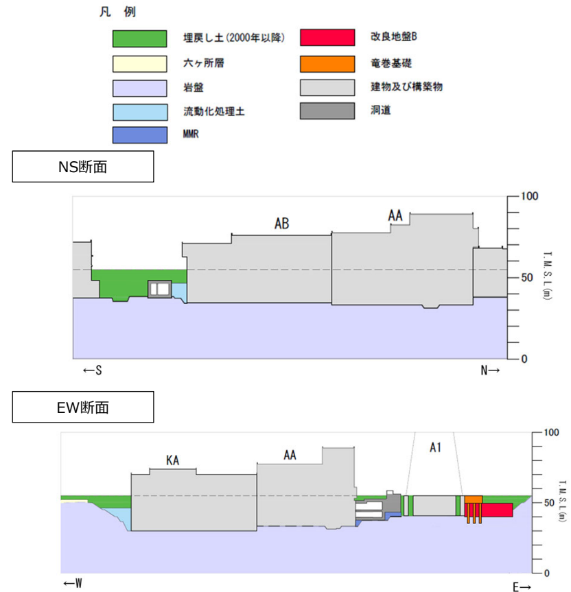
AA周辺グループにおける断面図
