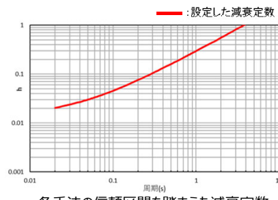
各手法の信頼区間を踏まえた減衰定数
