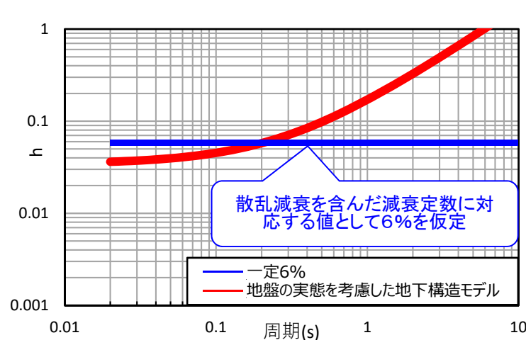
敷地の地盤の特徴を捉えた地下構造と仮定した値（6%一定）の比較（東側②エリア）
