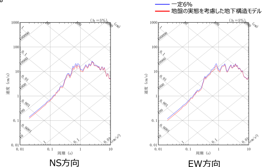
敷地の地盤の特徴を捉えた地下構造と周波数一定の設定（6%）の地盤応答比較（201103111446地震、東側②エリア）
