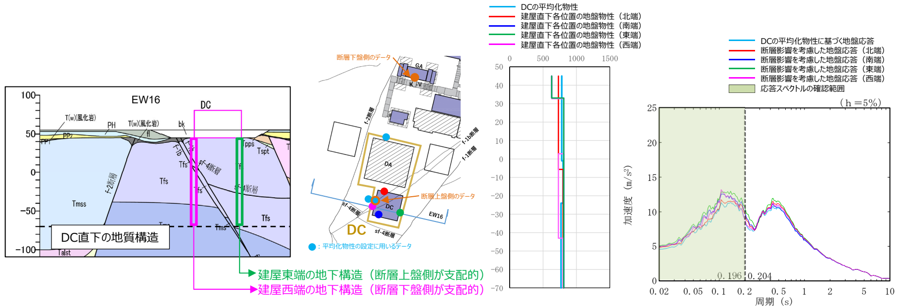
注記：縦点線はDCの一次固有周期（NS方向及びEW方向）を示す。 基礎底面レベルの応答スペクトル
