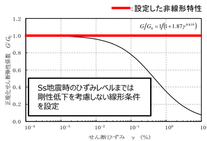
ひずみ依存特性 ( G/G_0-\gamma 関係) (細粒砂岩の例)
