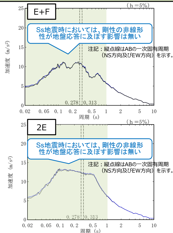
線形条件及び非線形条件における基礎底面レベルの入力地震動の比較（AB）
