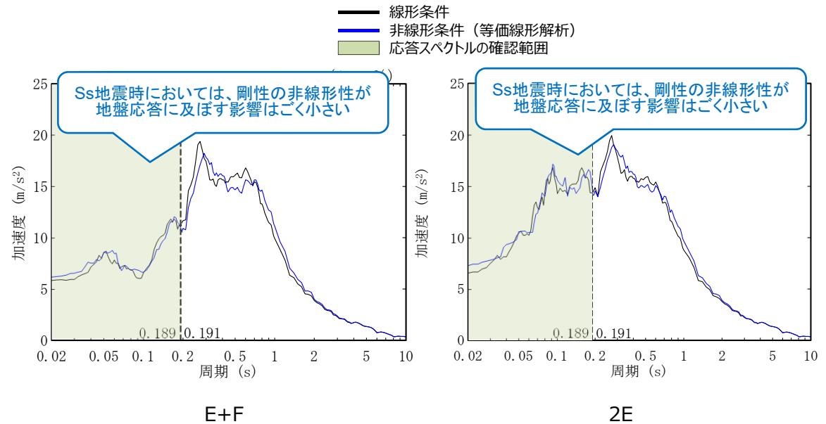
線形条件及び非線形条件における基礎底面レベルの入力地震動の比較（G14）
