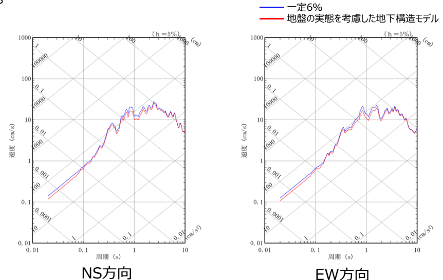
敷地の地盤の特徴を捉えた地下構造と周波数一定の設定（6%）の地盤応答比較（201103111446地震、東側⑤エリア）
