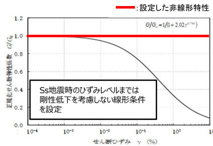
ひずみ依存特性 ( G/G_0-\gamma 関係) (軽石凝灰岩の例)
