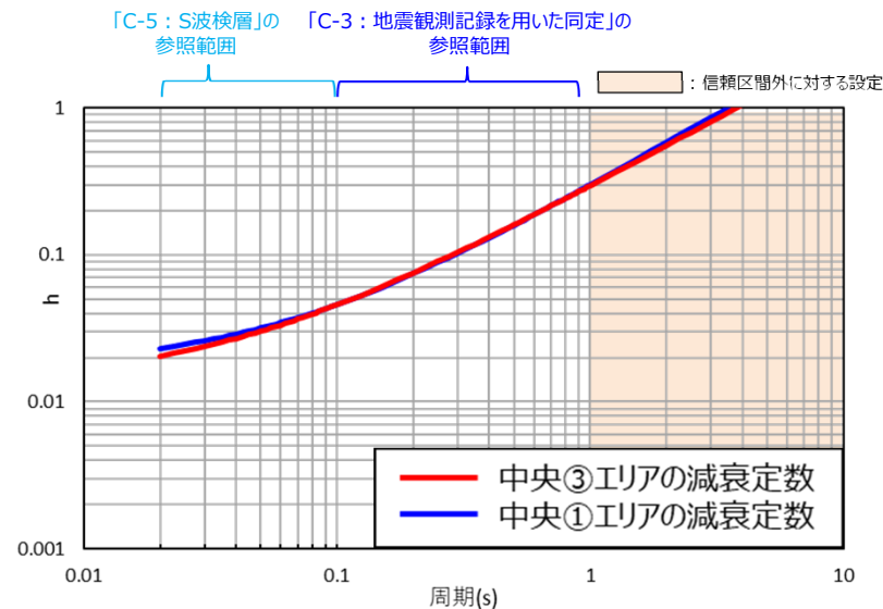
本エリアで仮定した減衰定数と 検証を行った減衰定数（中央①エリア）の比較
