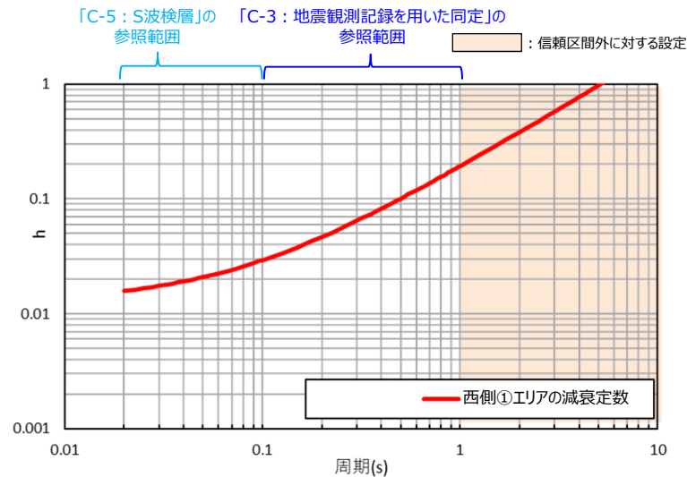
本エリアで仮定した減衰定数
