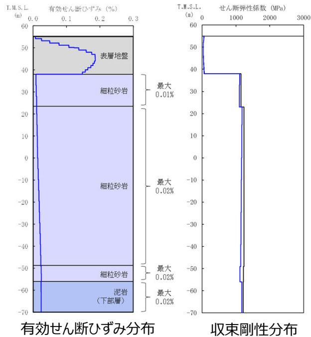
地盤の等価線形解析結果 (FA)
