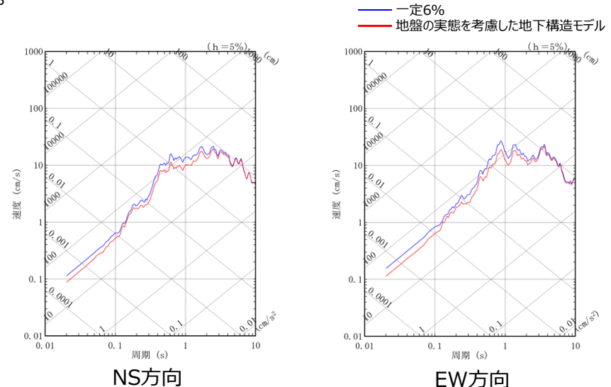
敷地の地盤の特徴を捉えた地下構造と周波数一定の設定（6%）の地盤応答比較（201103111446地震，中央②エリア）
