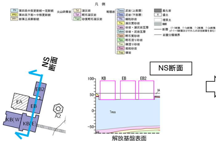
西側①エリアの地下構造
