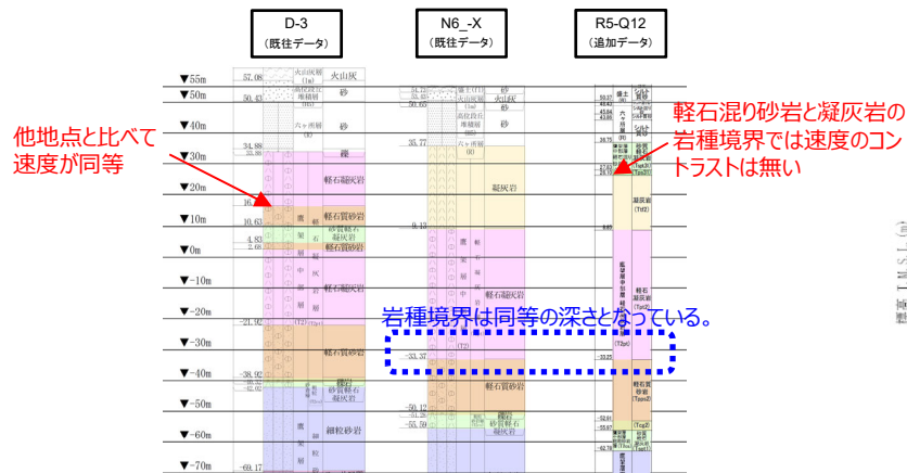
地質柱状図の比較 (グループ内の東西方向の順に整理)
