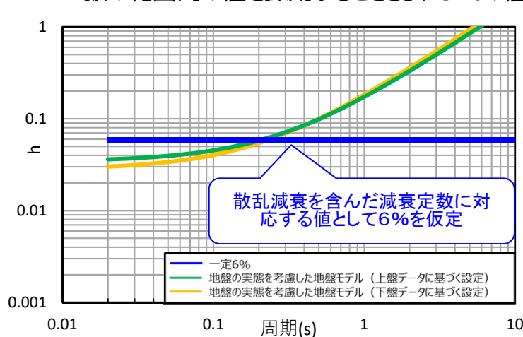
敷地の地盤の特徴を捉えた地下構造と仮定した値（6%一定）の比較（東側⑥エリア）
