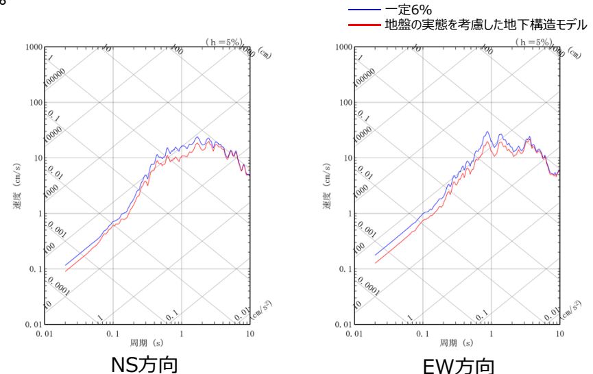
敷地の地盤の特徴を捉えた地下構造と周波数一定の設定（6%）の地盤応答比較（201103111446地震，中央③エリア）
