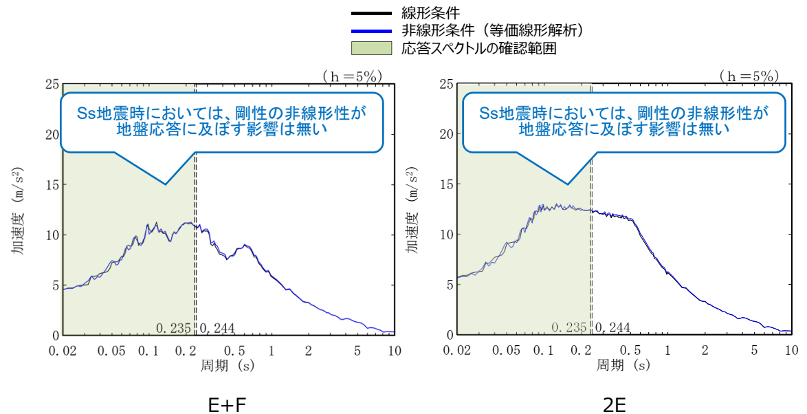
線形条件及び非線形条件における基礎底面レベルの入力地震動の比較 (FA)
