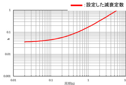
各手法の信頼区間を踏まえた減衰定数
