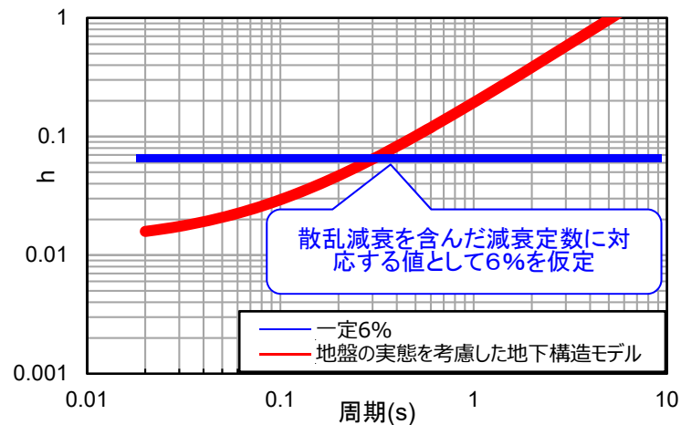
敷地の地盤の特徴を捉えた地下構造と仮定した値（6%一定）の比較（西側①エリア）
