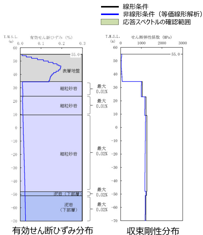
地盤の等価線形解析結果（AB）
