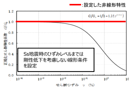
ひずみ依存特性 ( G/G_0-\gamma 関係) (泥岩（上部層）の例)
