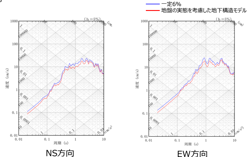
敷地の地盤の特徴を捉えた地下構造と周波数一定の設定（6%）の地盤応答比較（201103111446地震，中央①エリア）
