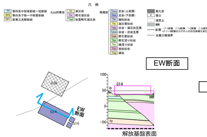
東側⑥エリアの地下構造
