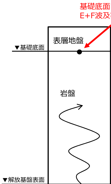
入力地震動の算定手法
