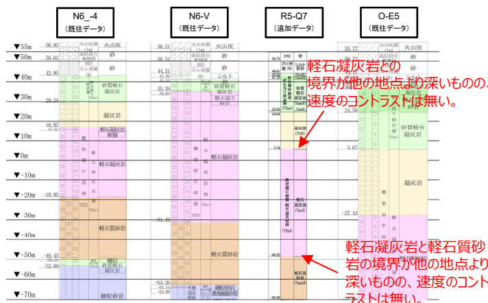
地質柱状図の比較 (グループ内の東西方向の順に整理)
