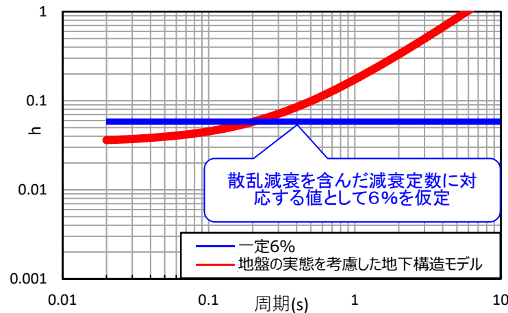
敷地の地盤の特徴を捉えた地下構造と仮定した値（6%一定）の比較（東側④エリア）
