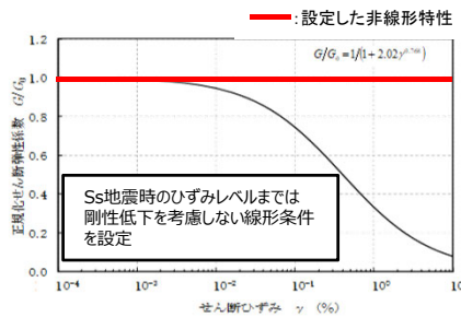
ひずみ依存特性 ( G/G_0 - \gamma 関係) (軽石凝灰岩の例)
