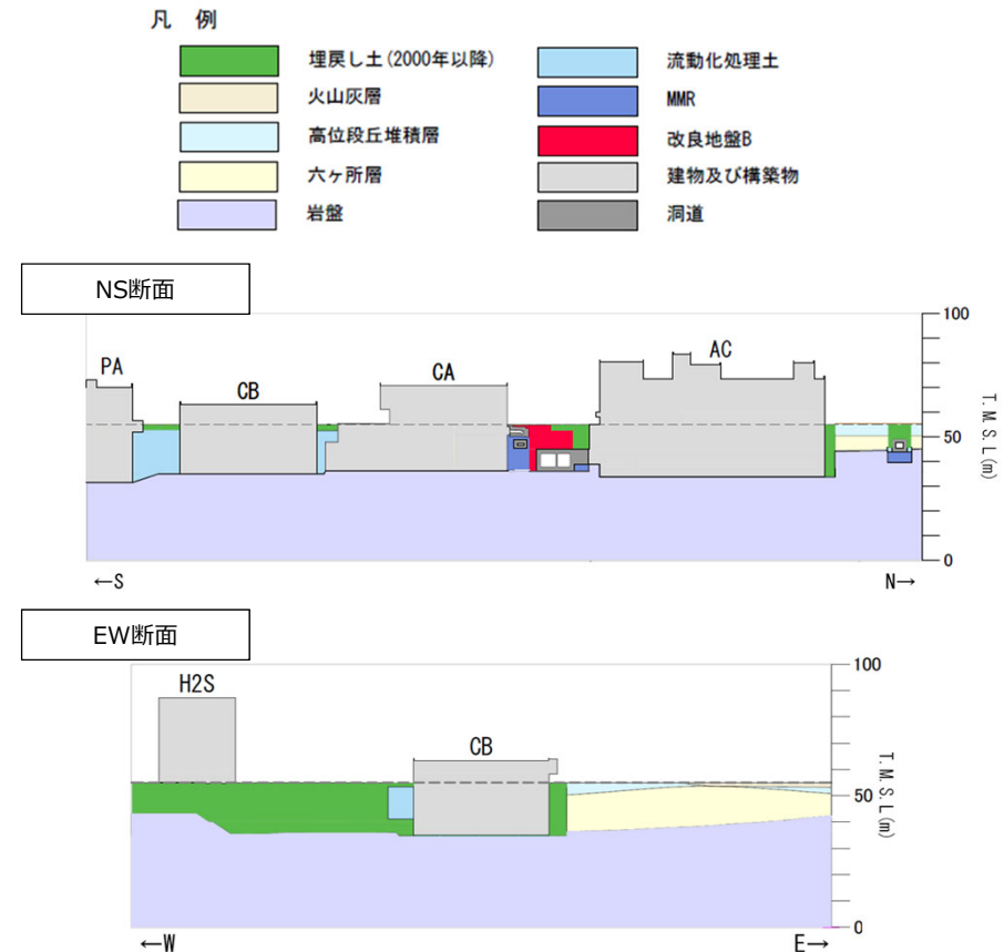
CBグループにおける断面図
