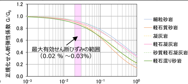
図b 各岩種のひずみ依存特性（ G/G_0 - \gamma 関係）
