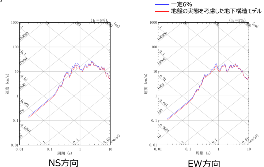
敷地の地盤の特徴を捉えた地下構造と周波数一定の設定（6%）の地盤応答比較（201103111446地震，東側③エリア）
