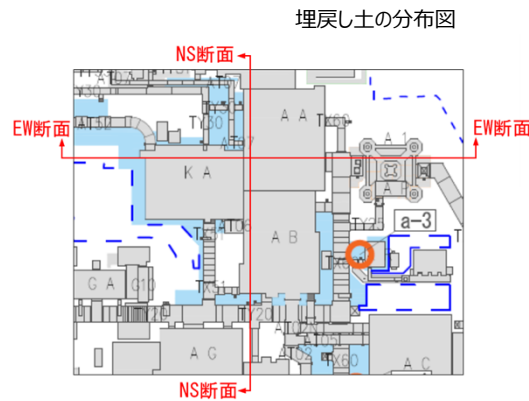
AA周辺グループにおける表層分布図
