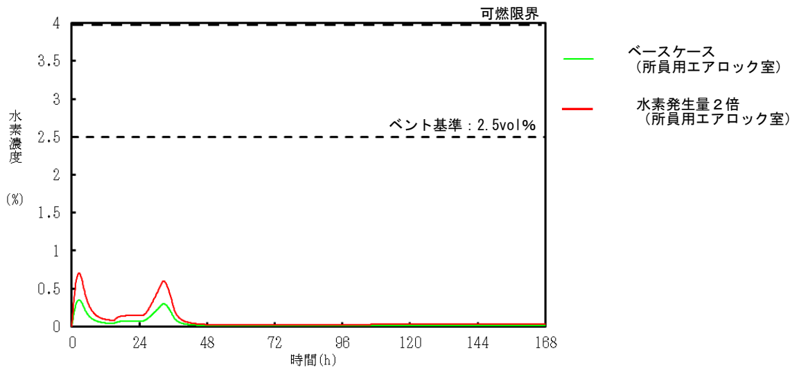
図4 所員用エアロック室の水素濃度推移 (水素発生量を増加させた場合の局所エリア格納容器ベントケース)
