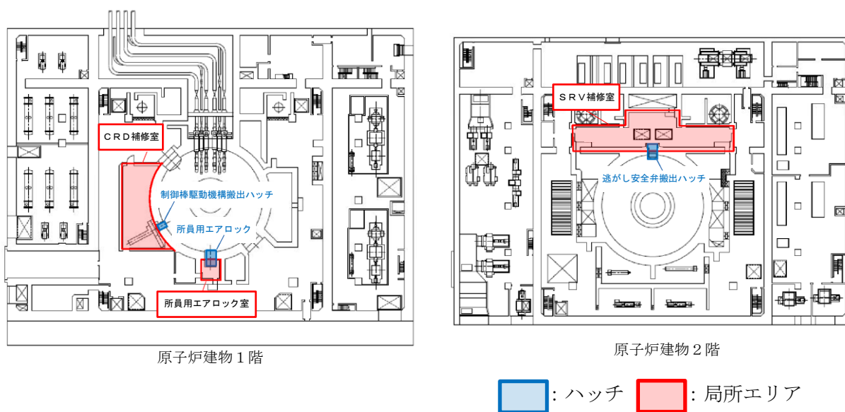
図 1.2.18 局所エリア配置図
