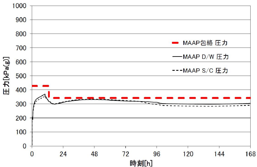
図 1. 2. 28 格納容器圧力の評価条件
