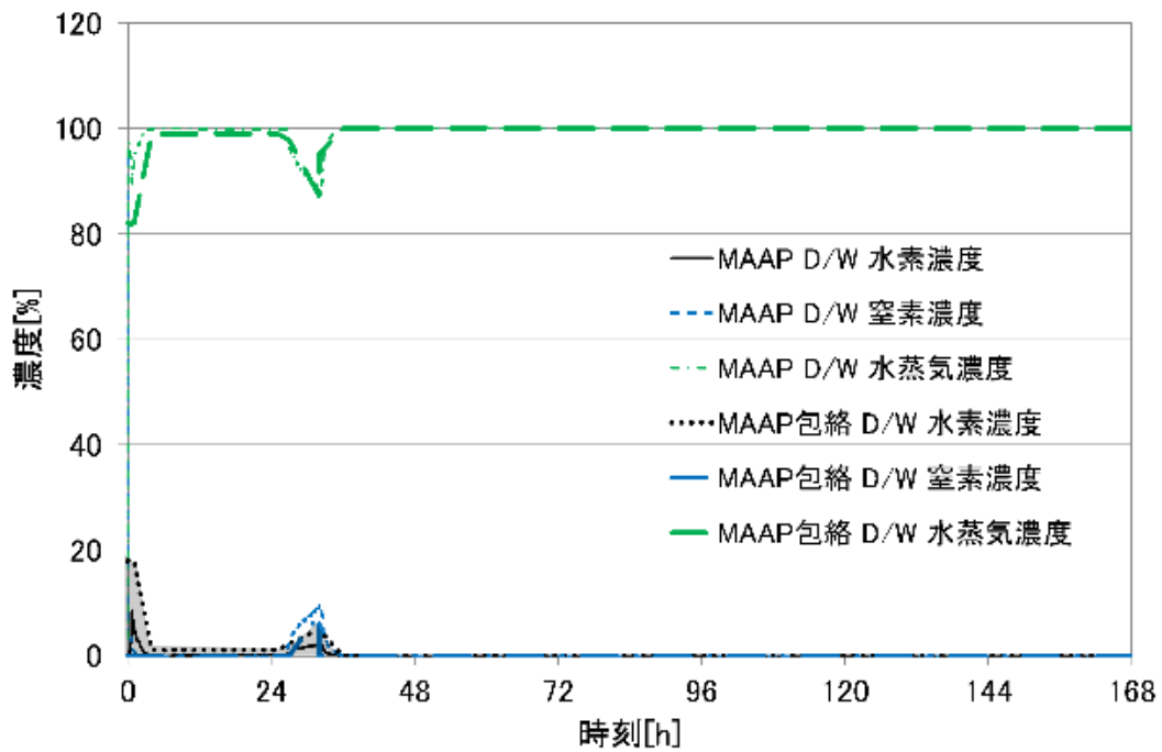
図 1. 2. 34 有効性評価の 2 倍相当の条件におけるドライウエルの気相濃度
