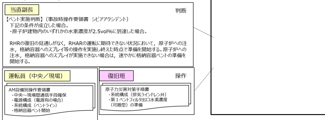
図 1.2.37 事故時操作要領書 シビアアクシデント等記載
