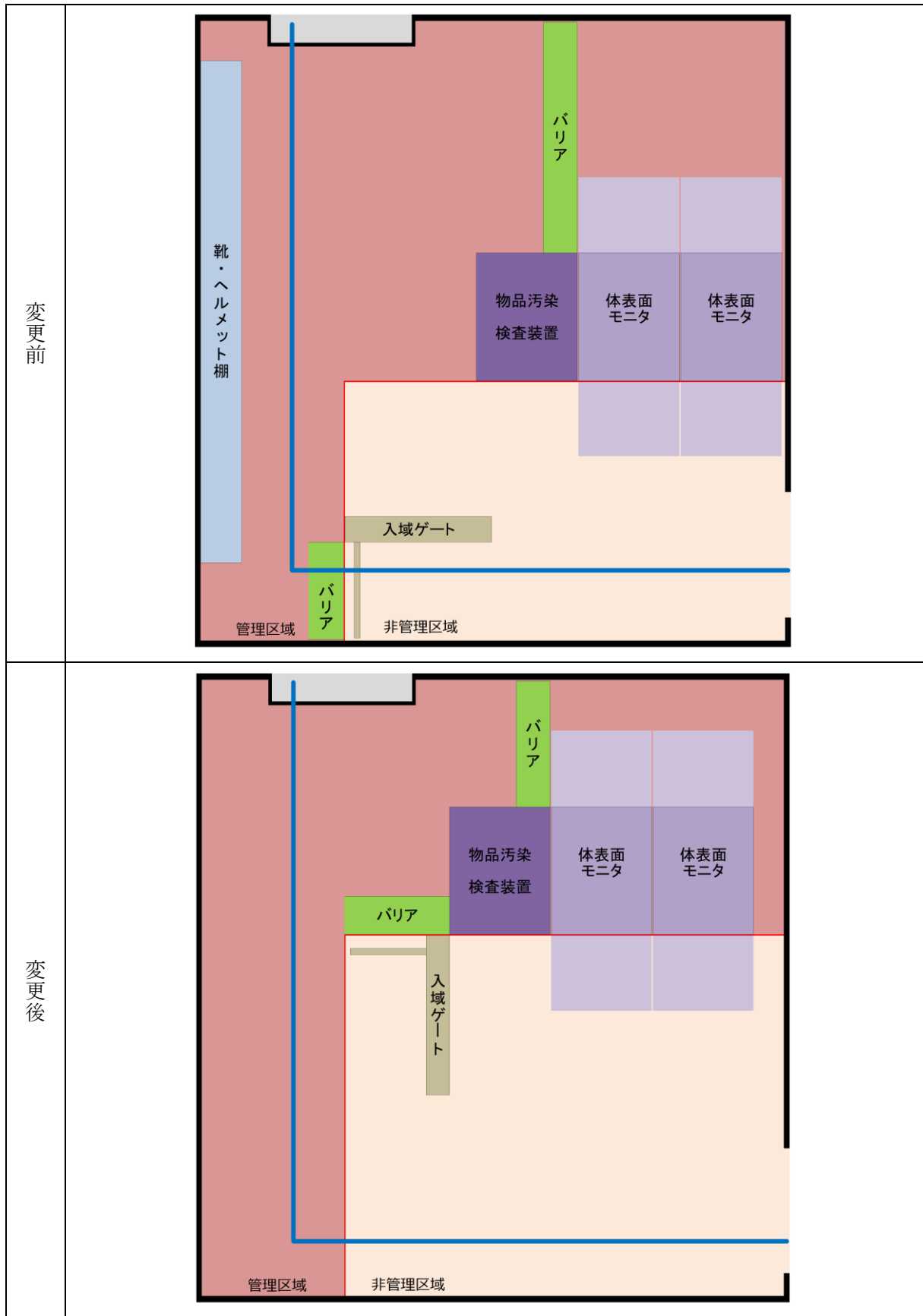
〔参考〕 具体的な変更内容（第2チェックポイント概略図）
