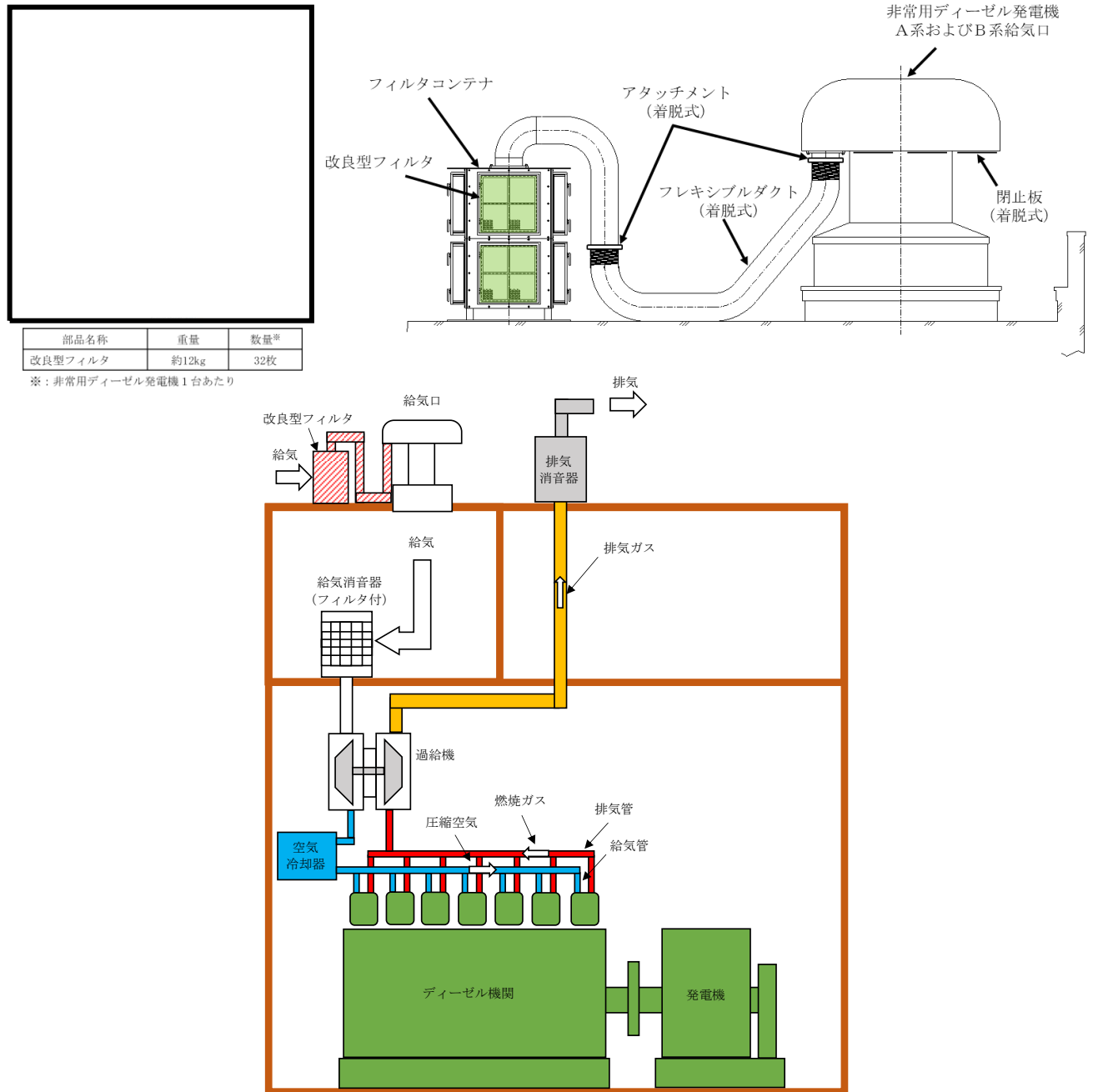
図1 フィルタ取付けおよび非常用ディーゼル発電機A系およびB系の給気ライン概略図
