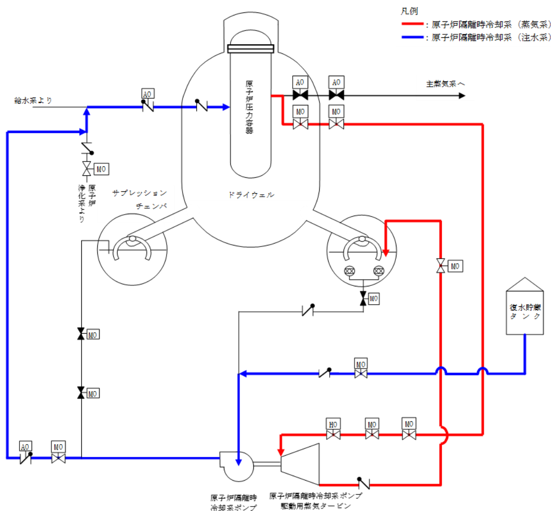
図3 原子炉隔離時冷却系使用時の系統図
