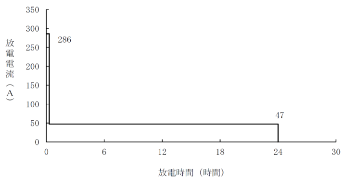
図 2.2.2-1 230V 系蓄電池(RCIC)負荷曲線
