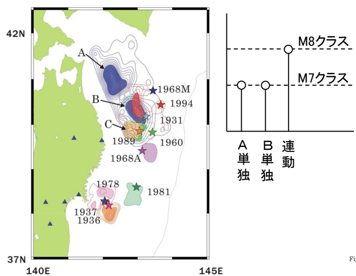
アスペリティの活動パターンと地震規模の関係 (Yamanaka and Kikuchi(2004), 永井ほか(2001))
