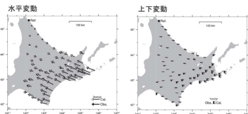
第2図 1999年9月から2003年8月までの平均的なすべり欠損速度分布。 Fig. 2 Distribution of slip-deficit rate from September, 1999 to August, 2003.
