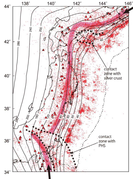
太平洋スラブ地殻内の地震の分布 (長谷川ほか(2012))
