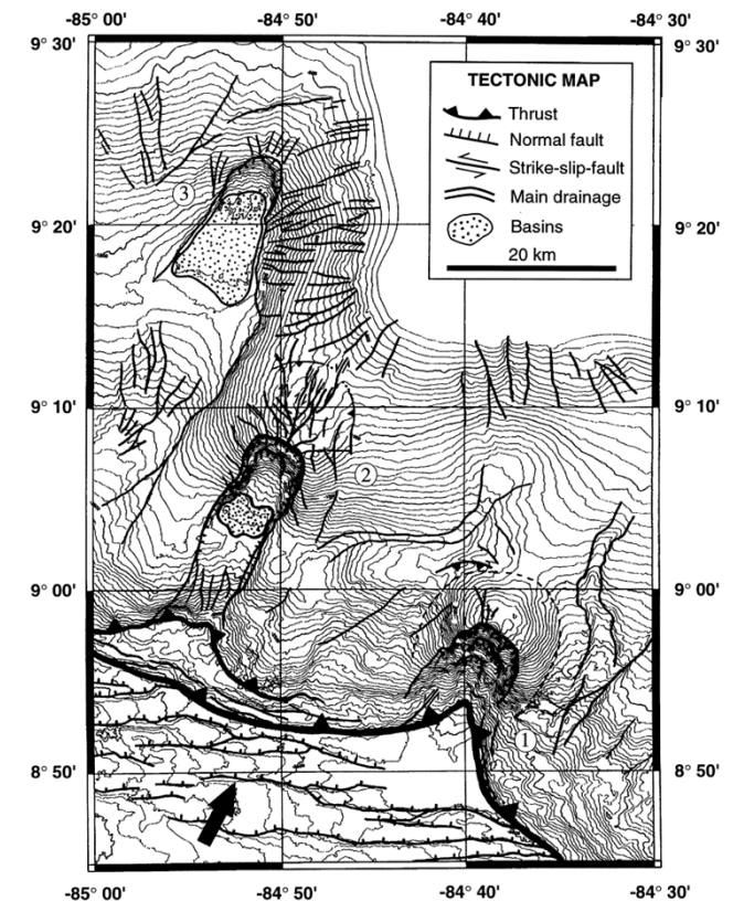
コスタリカ沖の海底地形図(○数字:沈み込む海山位置) (Dominguez et al.(1998))
