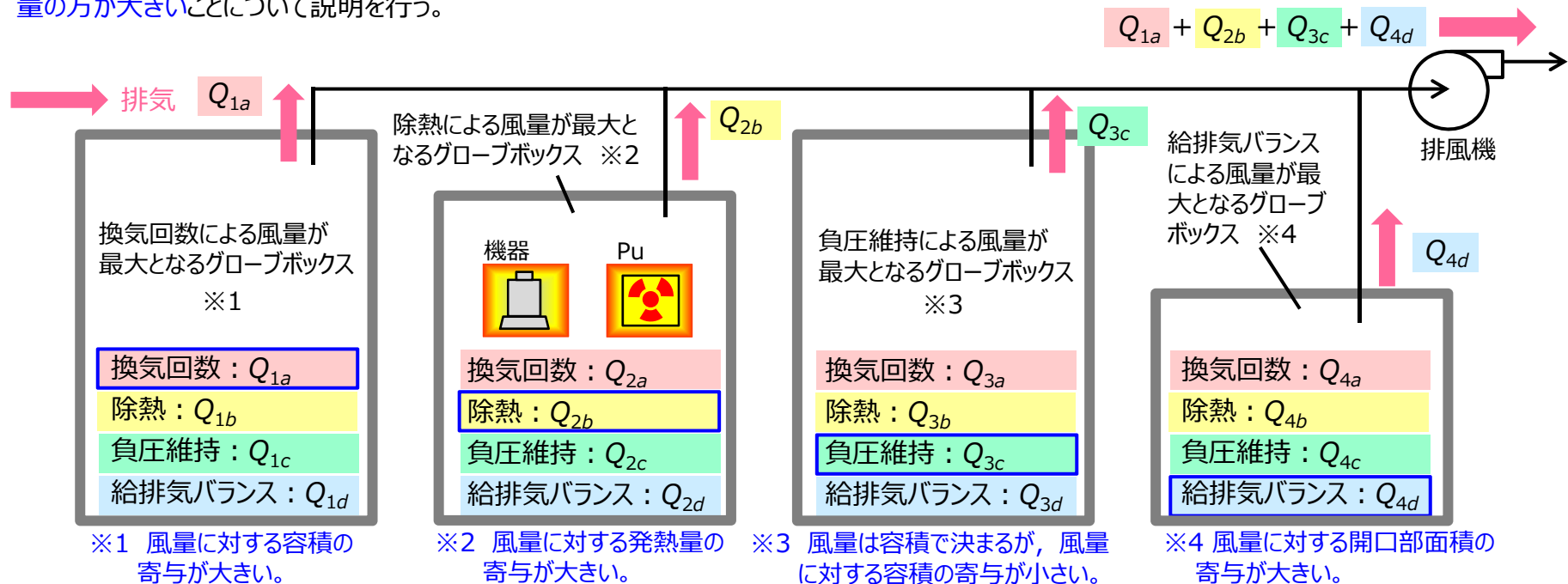
第1.7図 風量決定因子の中で最大となる風量の積み上げイメージ（グローブボックス）
