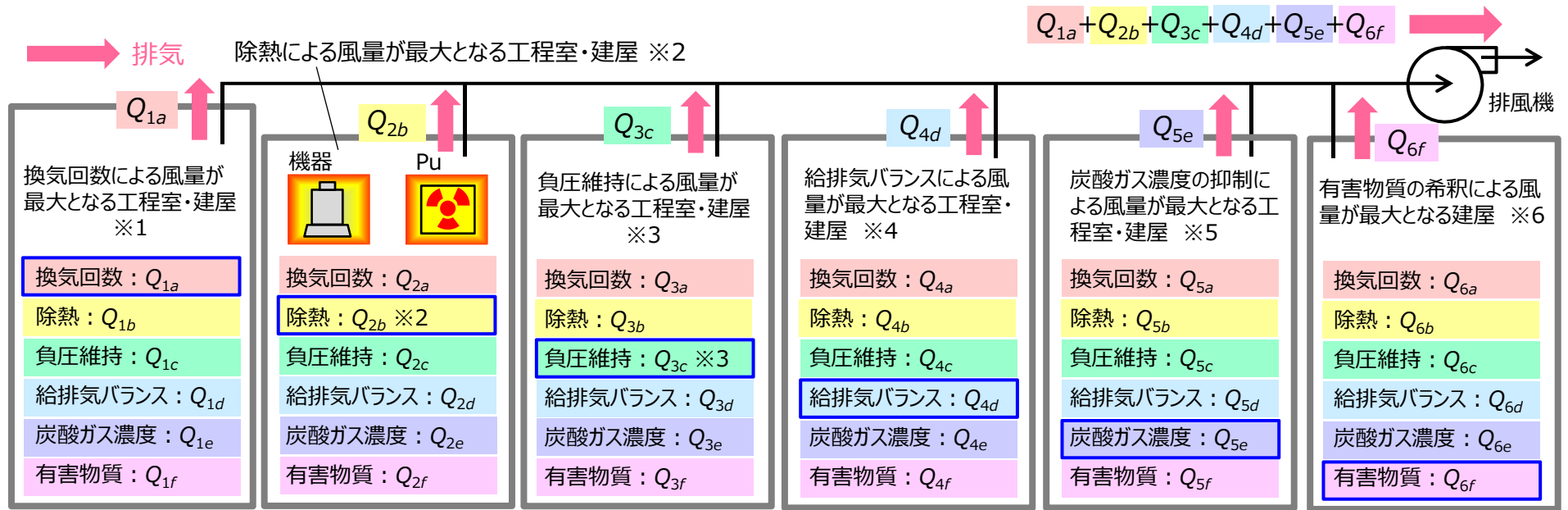
第1.8図 風量決定因子の中で最大となる風量の積み上げイメージ（工程室及び建屋）
