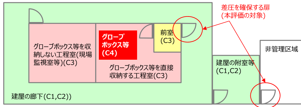
第2.2.1.4図 差圧を確保する扉（図中の括弧内は汚染区分を示す）
