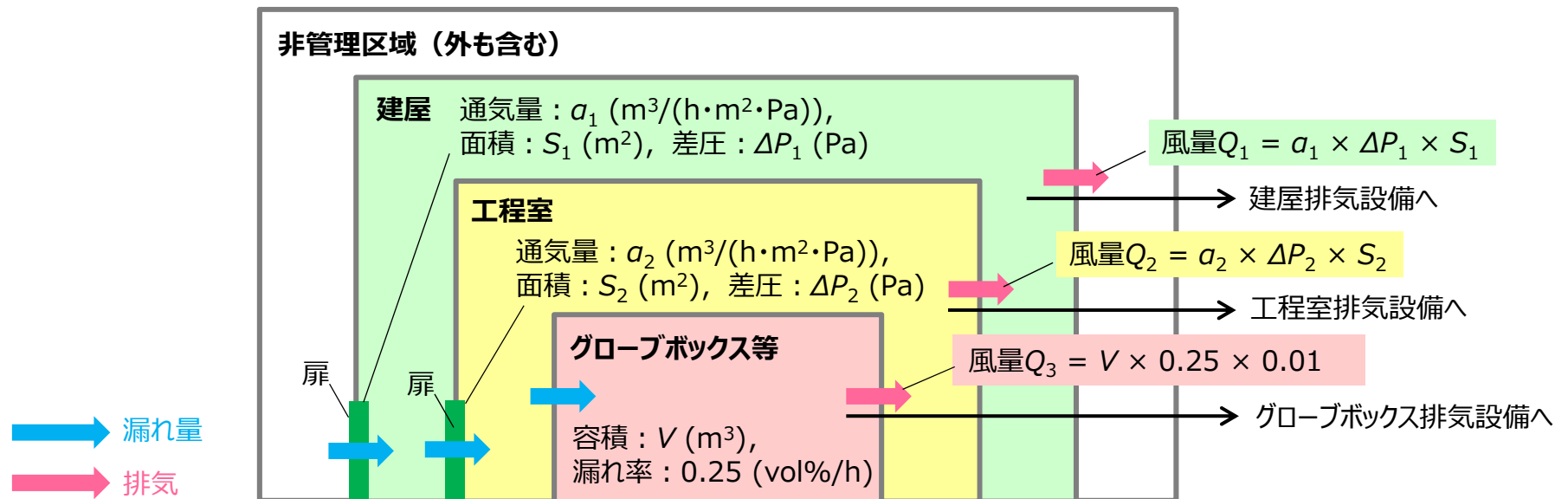
第1.4図 負圧維持による風量設定のイメージ
