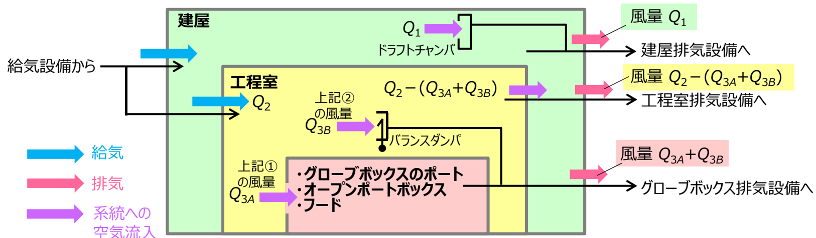
第1.5図 給排気バランス調整による風量設定のイメージ
