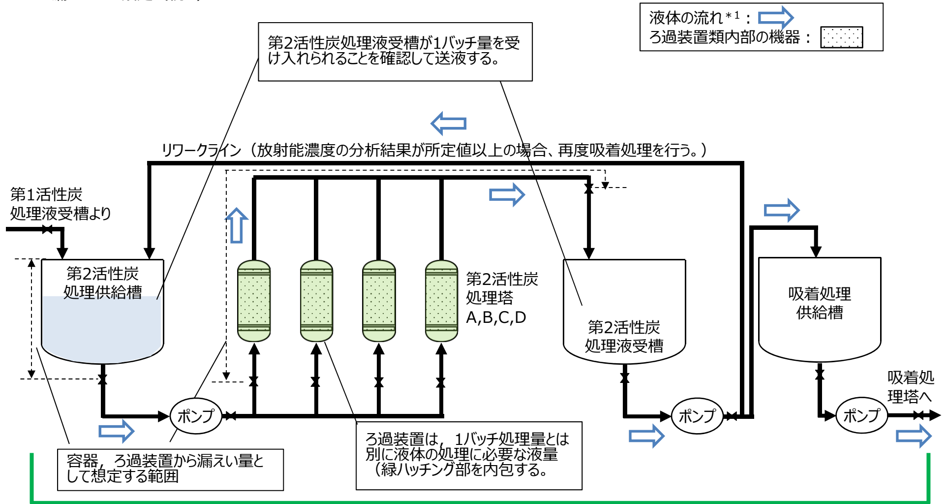
X-97 第2活性炭・吸着処理GB漏えい液受皿1
