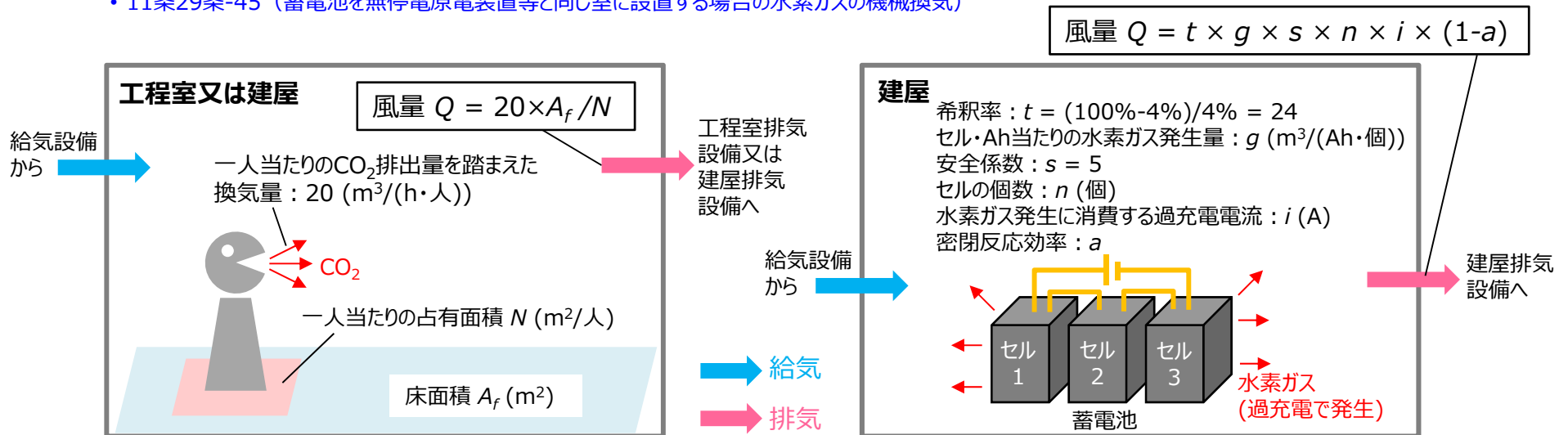
第1.6図 炭酸ガス濃度の抑制による風量設定のイメージ(左図)及び有害物質の希釈による風量設定のイメージ(右図)
