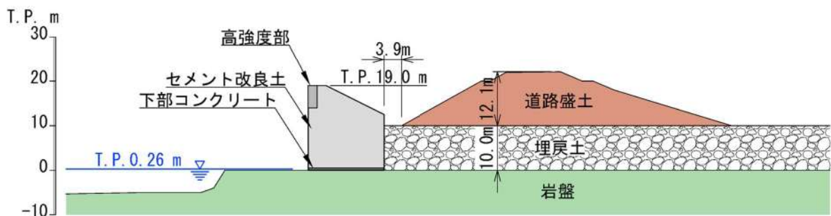
断面図 (7a-7a')
