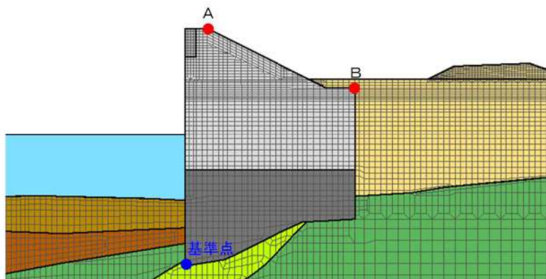
第 7-50 図 防潮堤天端（T.P. 19.0m）及び防潮堤平場端部（T.P. 8.5m）の全時刻最大の相対変位
