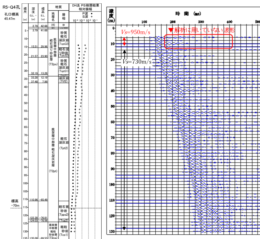
参考 1-3-7 図 表層の影響が考えられる観測波形 (R5-Q4 : コリレーション後 V_s )
