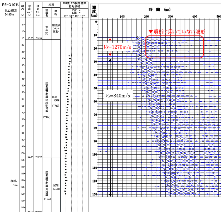
参考 1-3-8 図 表層の影響が考えられる観測波形 (R5-Q10 : コリレーション後 V_s )
