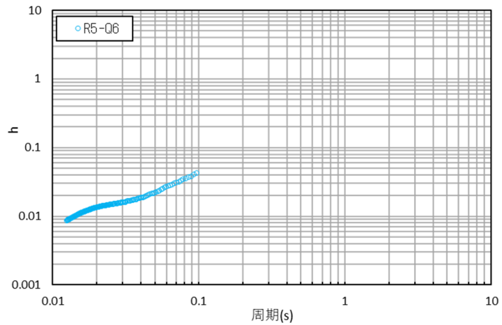
参考 1-3-14 図 コリレーション波形と減衰定数 (R5-Q6 孔: 観測深度 GL-8m~-130m)
