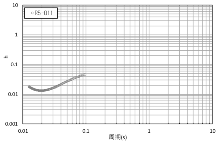
参考 1-3-19 図 コリレーション波形と減衰定数 (R5-Q11 孔: 観測深度 GL-12m~-130m)
