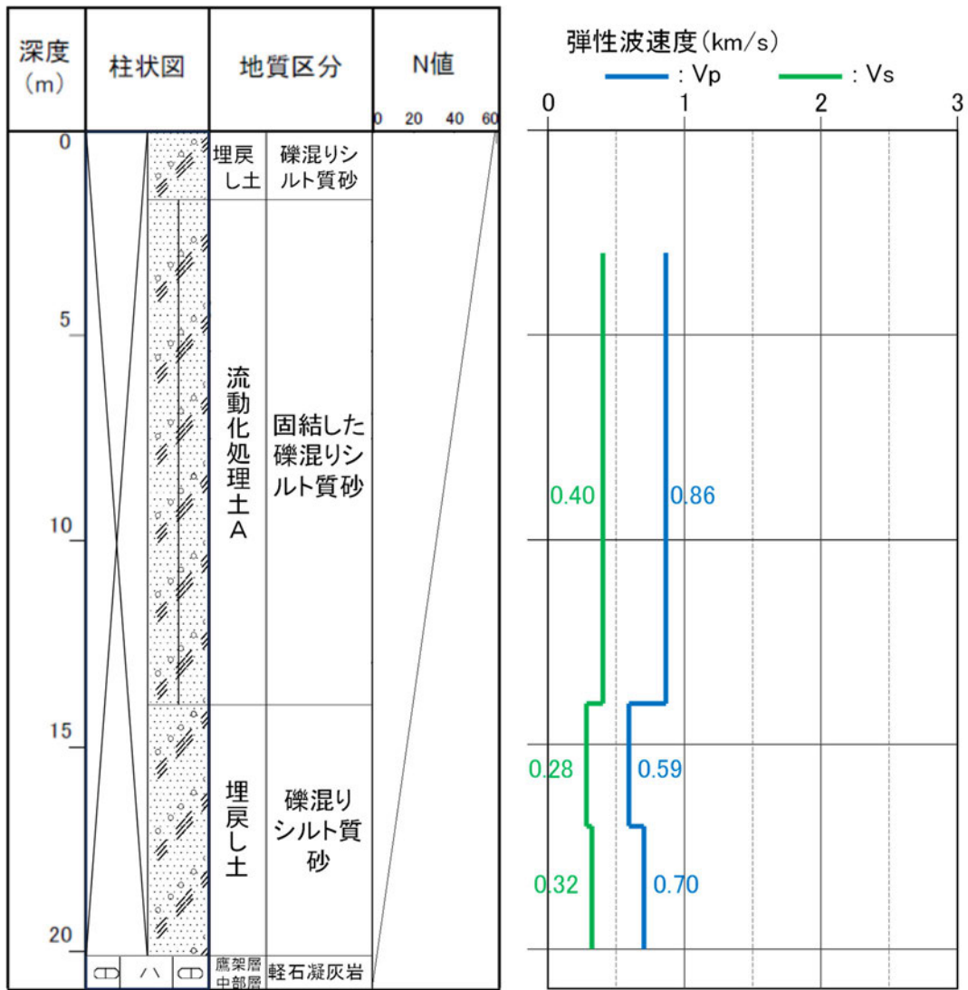
参考2-26図 ボーリング柱状図 (f1-11孔)
