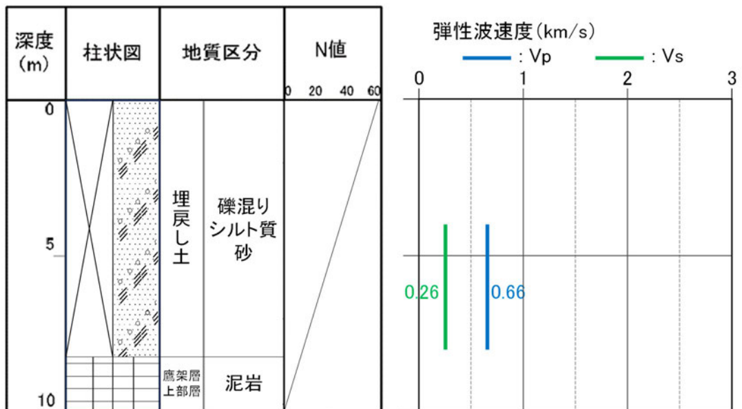
参考2-30図 ボーリング柱状図 (f1-15孔)
