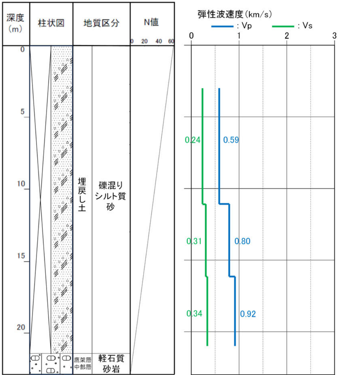
参考2-27図 ボーリング柱状図 (f1-12孔)
