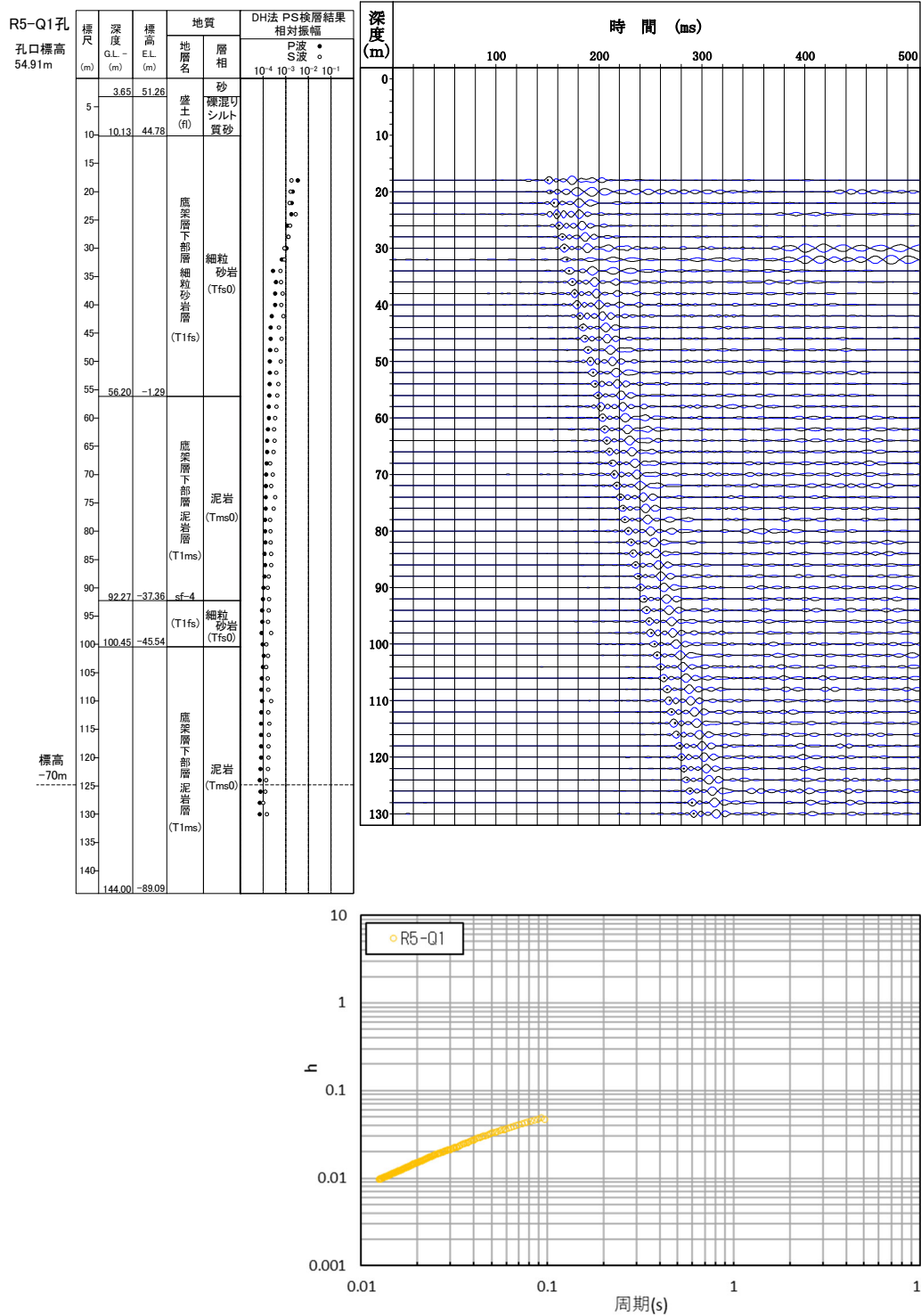
参考 1-3-9 図 コリレーション波形と減衰定数
