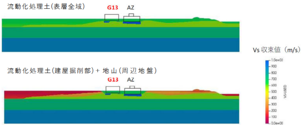
参考 9-2 図 (3) G13 建屋 (NS 方向) 解析断面 Vs 分布図
