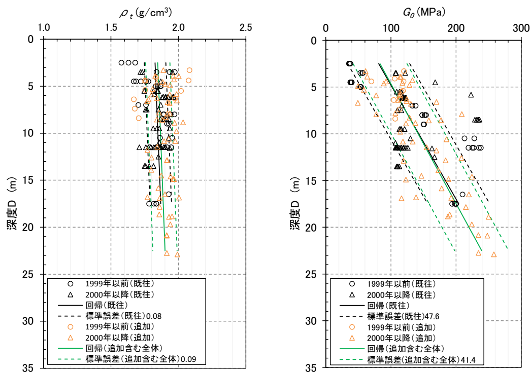
第 3.4-1 図 湿潤密度分布(全 30 孔)
