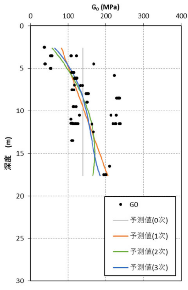
第 3.3.2-2 図 動せん断弾性係数 G_0 の任意次数回帰
