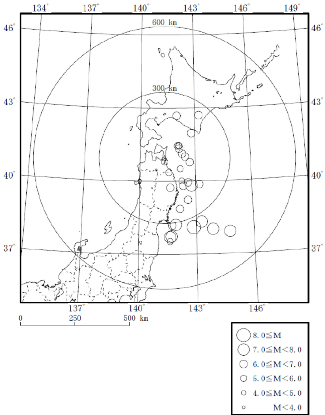
参考 2-2 図 地震数を 30 地震とした評価に用いた地震の震央分布 (西側地盤)
