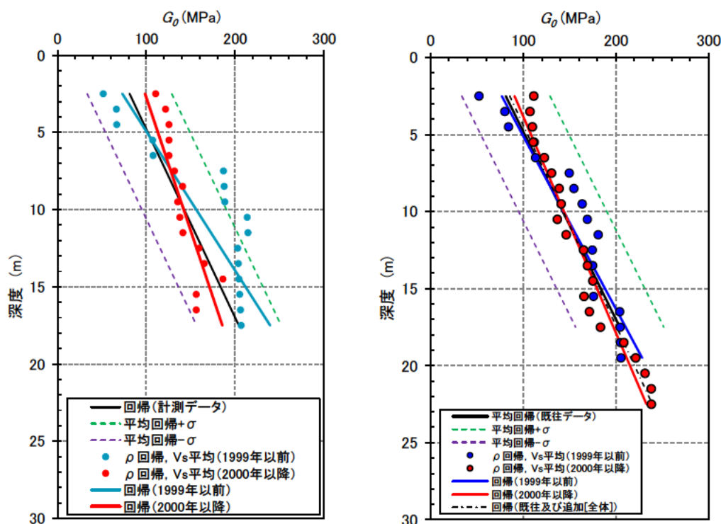
既往ボーリングデータ (第3.3.3-6図)
