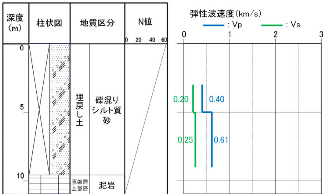
参考2-19図 ボーリング柱状図 (f1-4孔)
