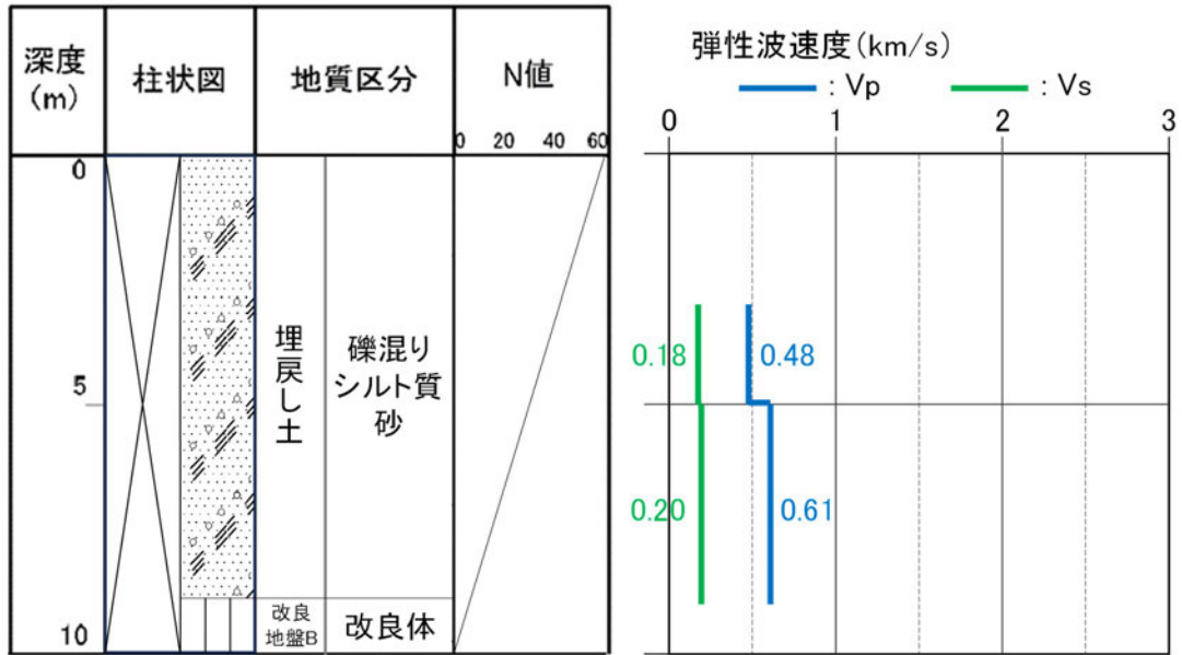
参考2-25図 ボーリング柱状図 (f1-10孔)
