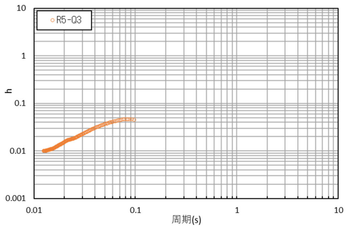
参考 1-3-11 図 コリレーション波形と減衰定数 (R5-Q3 孔: 観測深度 GL-8m~-130m)
