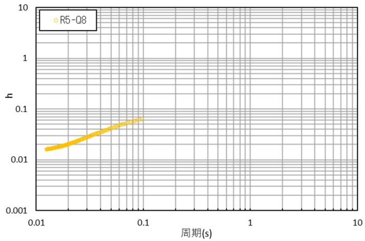
参考 1-3-16 図 コリレーション波形と減衰定数 (R5-Q8 孔: 観測深度 GL-30m~-130m)
