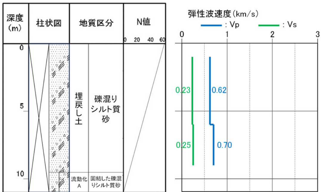
参考2-24図 ボーリング柱状図 (f1-9孔)
