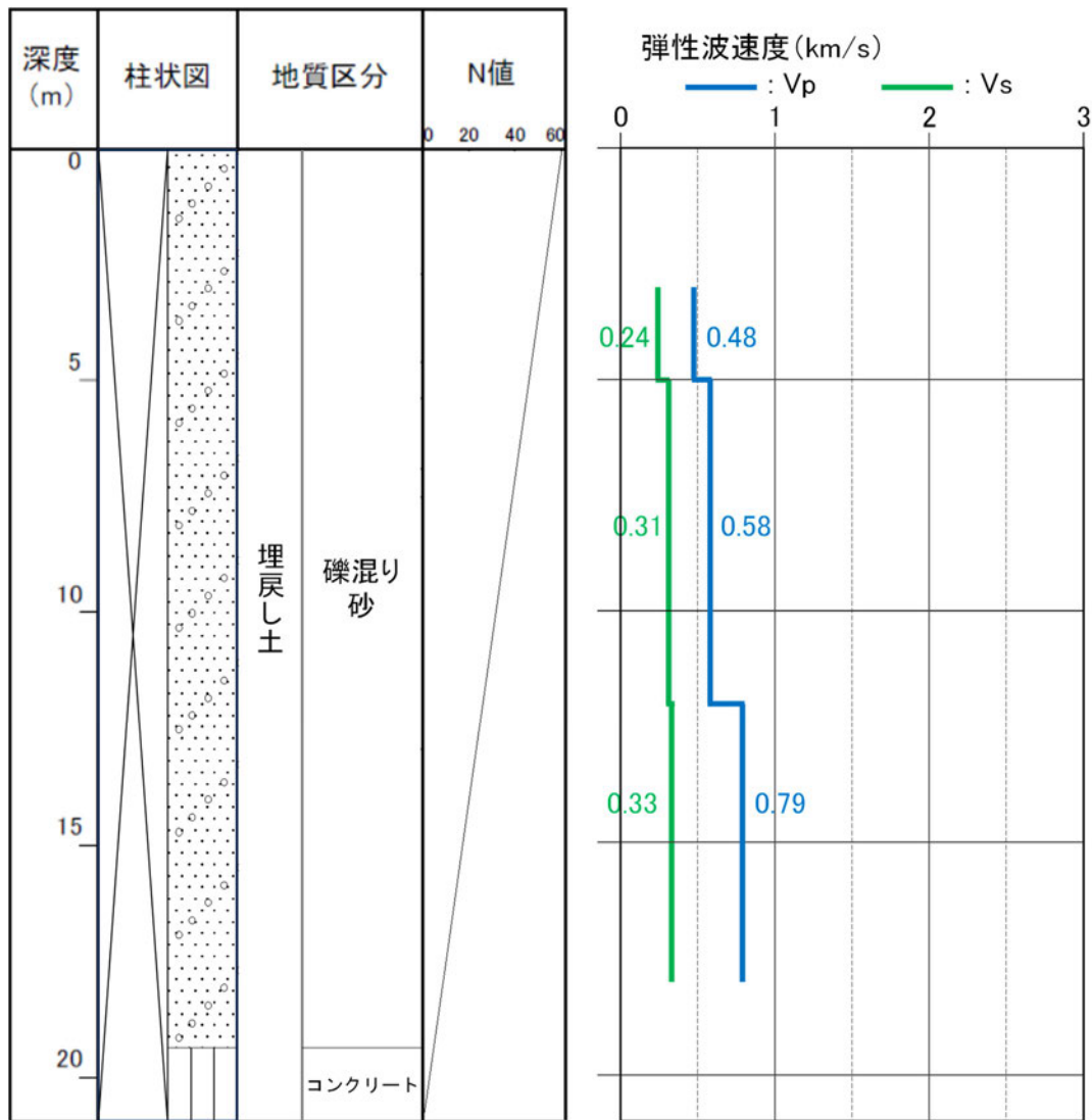
参考 2-31 図 ボーリング柱状図 (w-1 孔 [地下水位観測孔])
