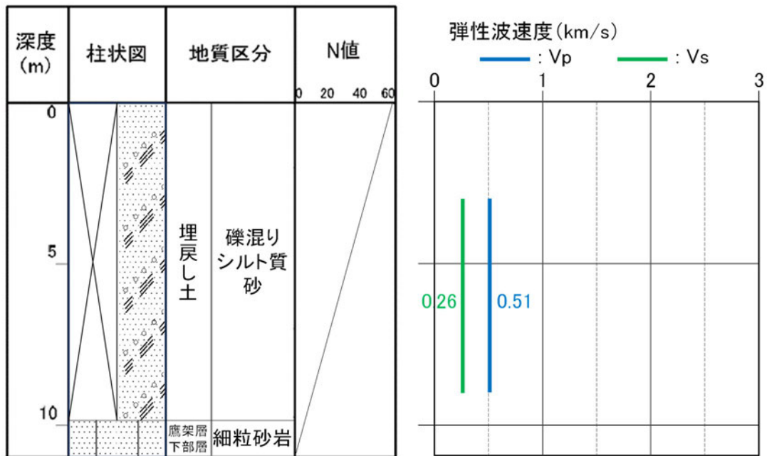
参考2-23図 ボーリング柱状図 (f1-8孔)
