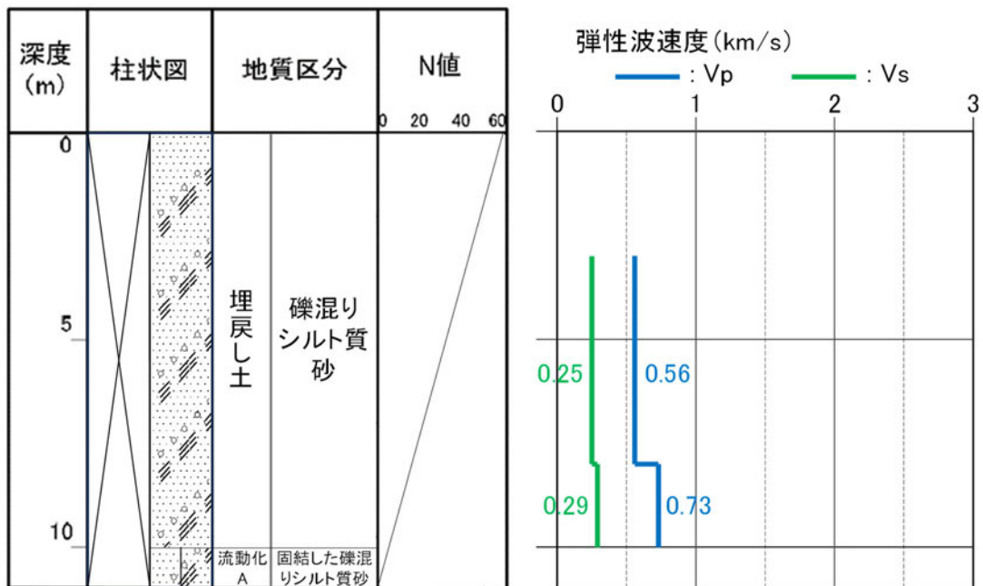
参考2-21図 ボーリング柱状図 (f1-6孔)
