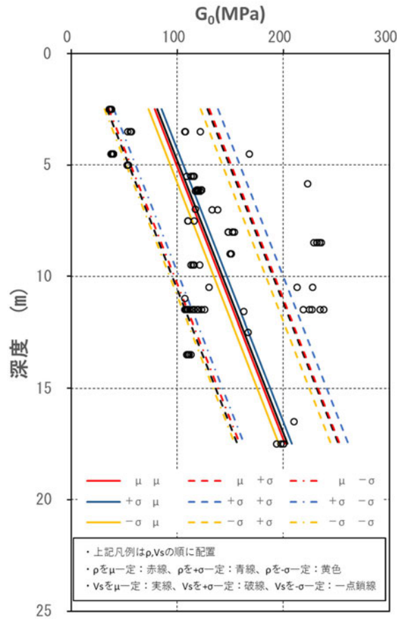
第 3.3.3-3 図 G_0 回帰の比較
