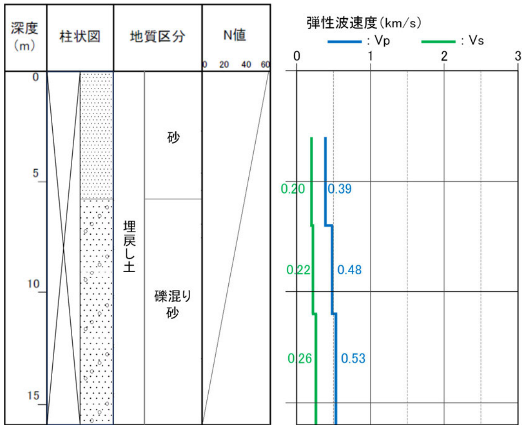
参考2-32図 ボーリング柱状図 (w-2孔[地下水位観測孔])
