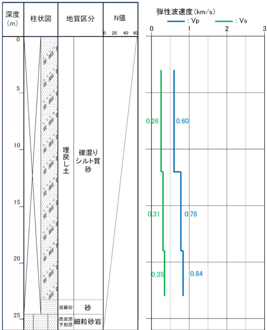
参考2-17図 ボーリング柱状図 (f1-2孔)
