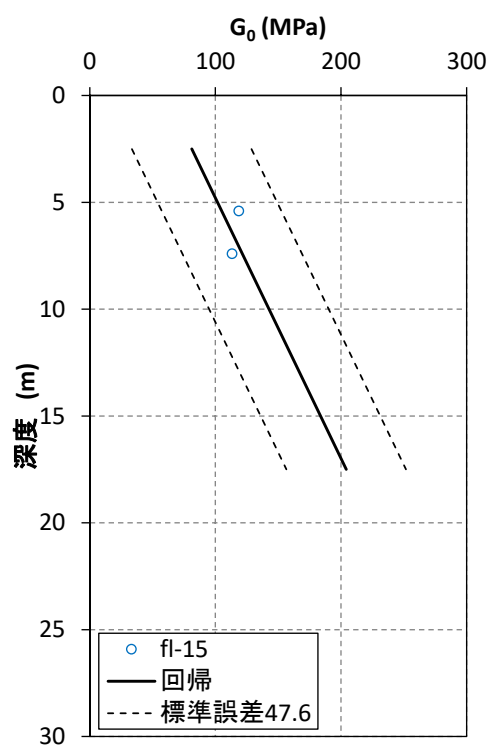
参考 3-1 図(2) ボーリング孔毎の埋戻し土の G_0 (1999 年以前)
