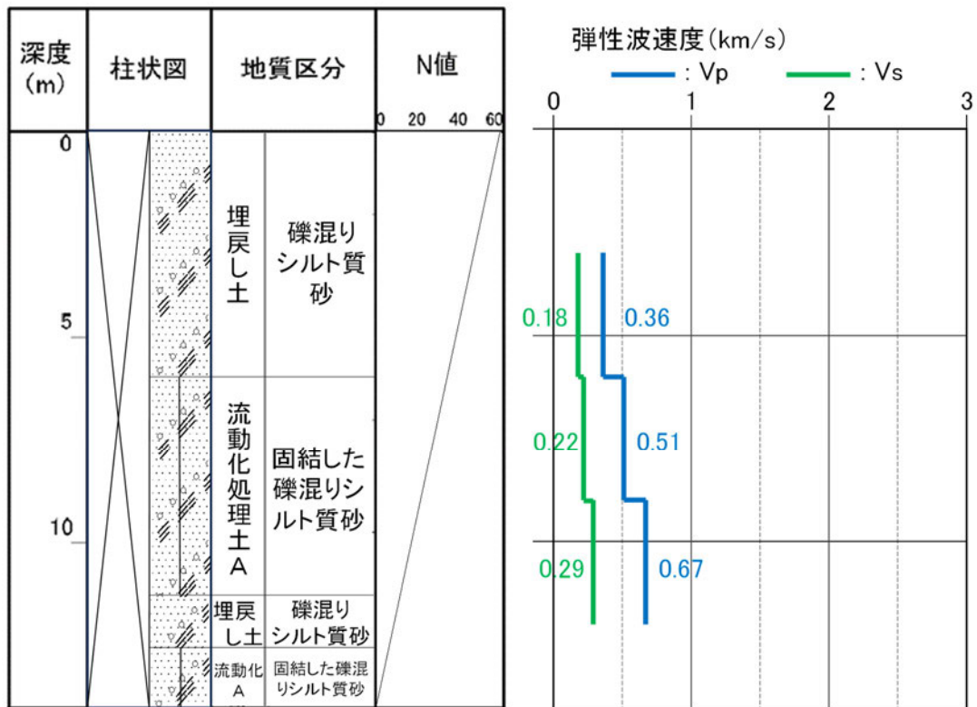
参考2-28図 ボーリング柱状図 (f1-13孔)
