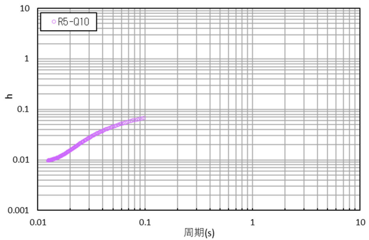
参考 1-3-18 図 コリレーション波形と減衰定数 (R5-Q10 孔: 観測深度 GL-28m~-130m)
