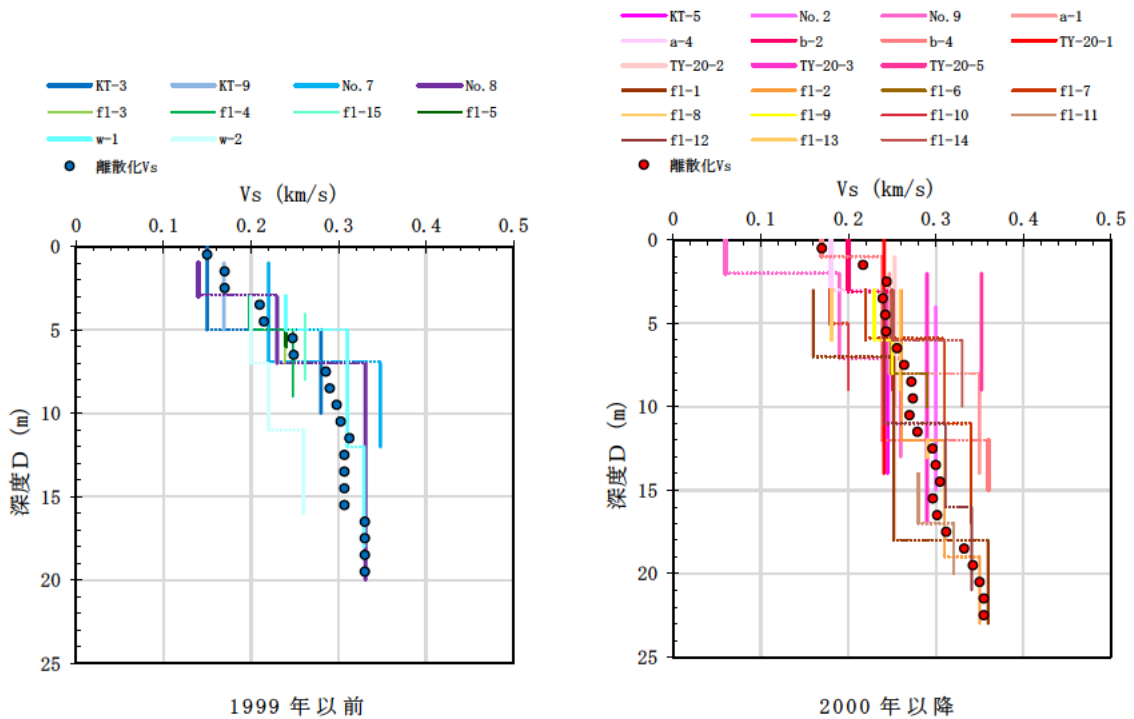
第 3.4-4 図 施工年代別の V_s と離散化 V_s
