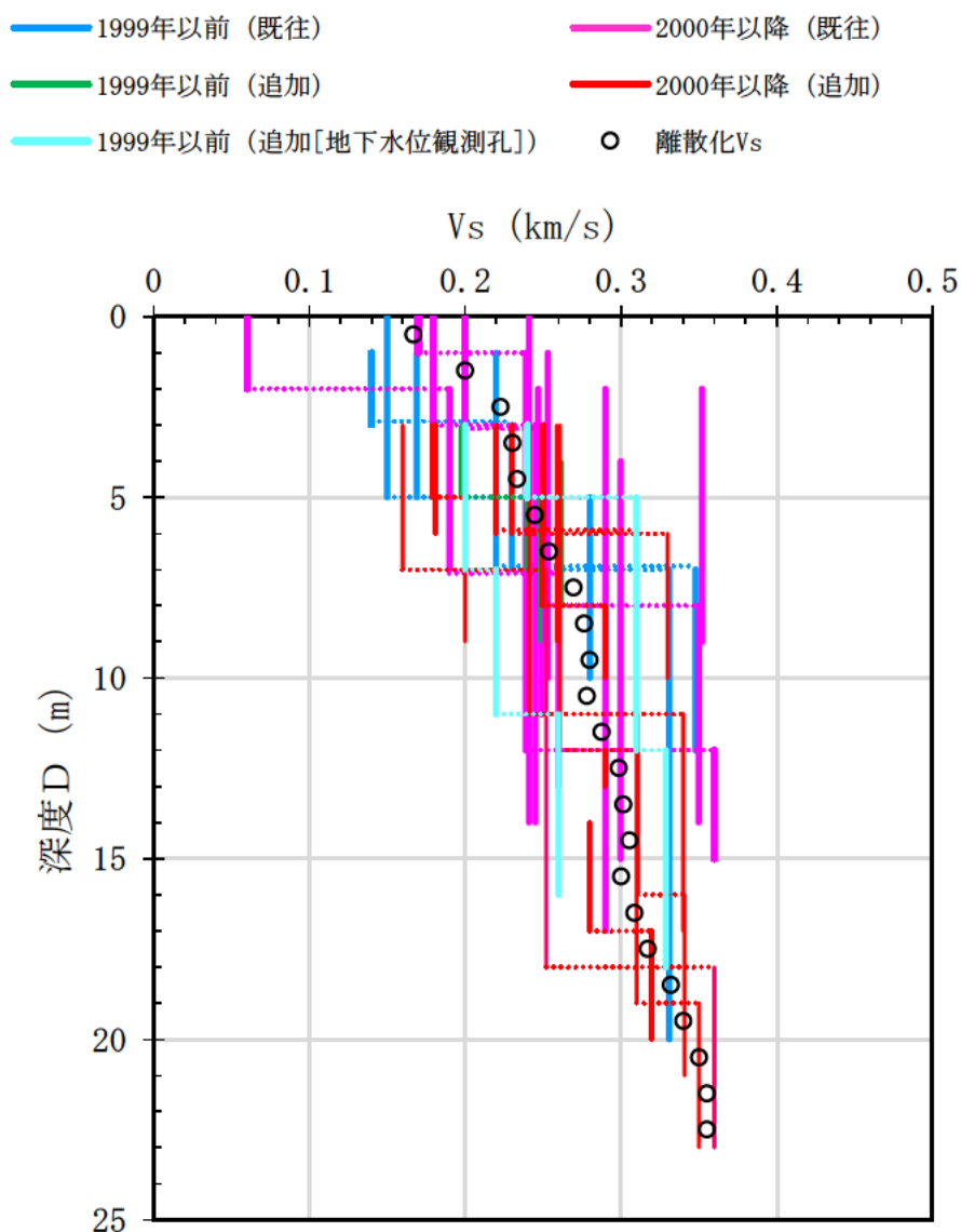
第 3.4-3 図 ボーリング柱状図による V_s と離散化 V_s (全 32 孔)
