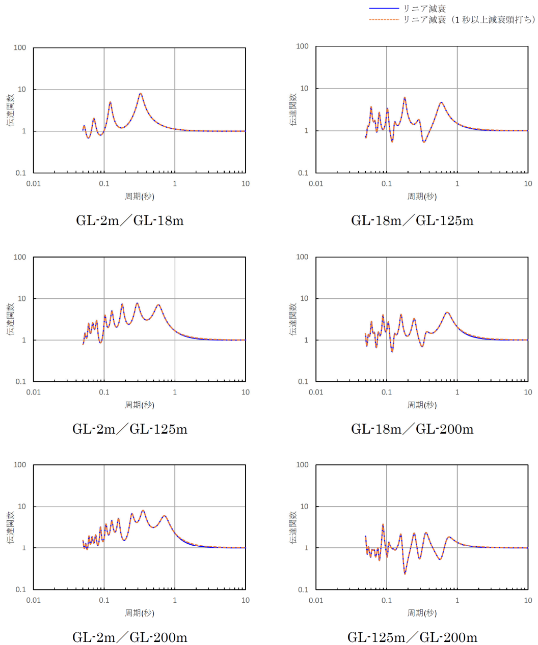
参考 3-5 図 伝達関数（長周期側の減衰定数パラメータスタディ結果） （東側地盤 水平方向）
