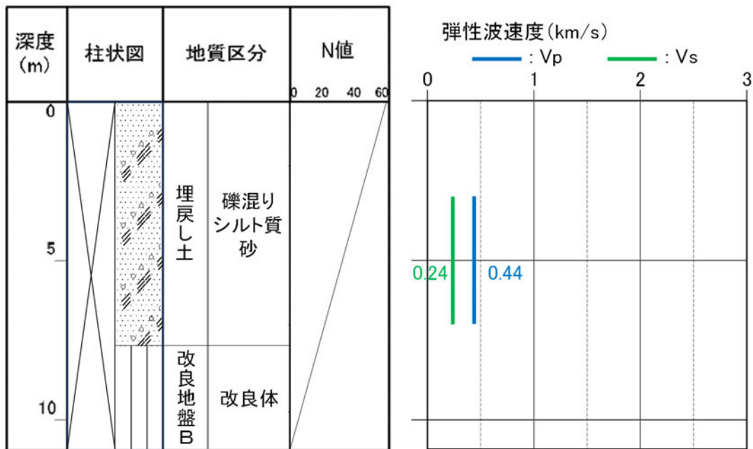
参考2-18図 ボーリング柱状図 (f1-3孔)
