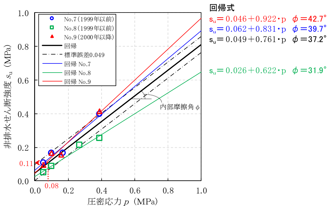
第 3.2-9 図 埋戻し土の強度特性（非排水せん断強度と圧密応力の関係） （再処理施設，廃棄物管理施設及びMOX燃料加工施設の事業変更許可申請書より抜粋して加筆）
