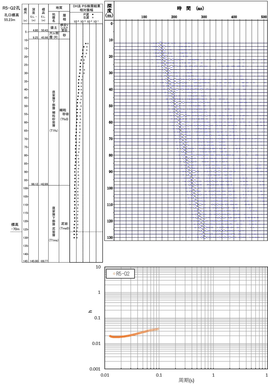
参考 1-3-10 図 コリレーション波形と減衰定数 (R5-Q2 孔: 観測深度 GL-12m~-130m)
