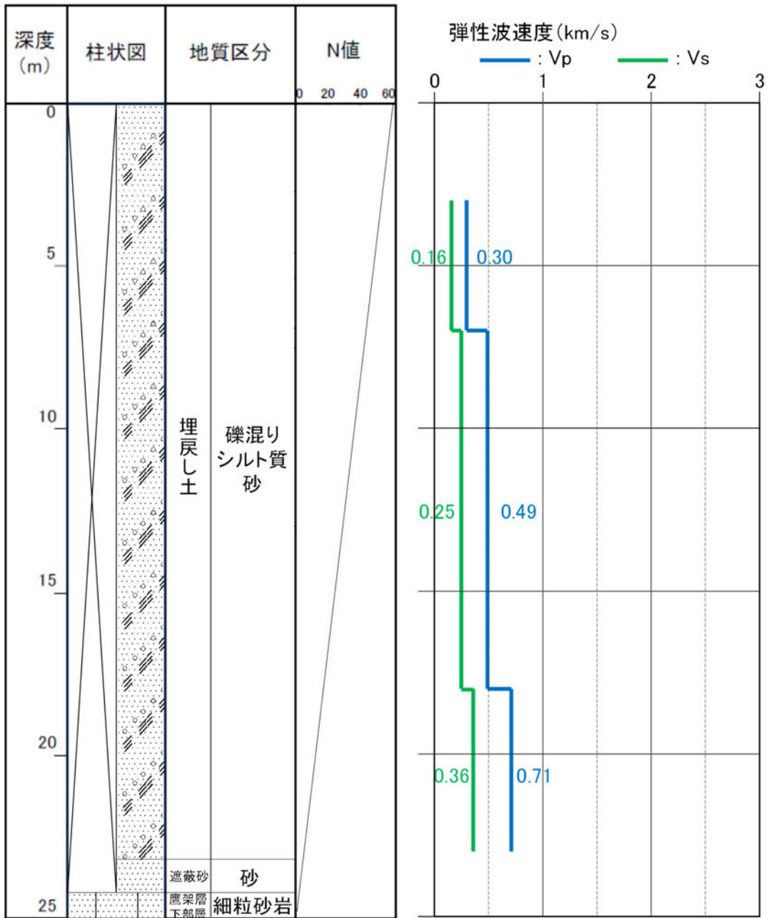
参考2-16図 ボーリング柱状図 (f1-1孔)
