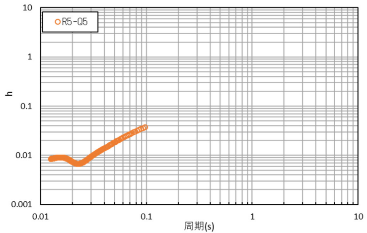
参考 1-3-13 図 コリレーション波形と減衰定数 (R5-Q5 孔: 観測深度 GL-12m~-130m)
