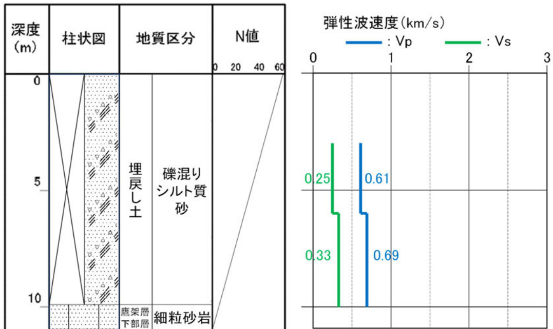
参考2-29図 ボーリング柱状図 (f1-14孔)
