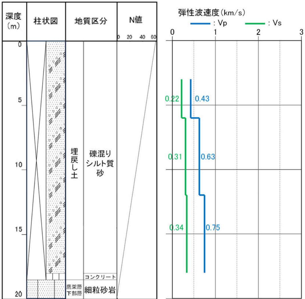
参考2-22図 ボーリング柱状図 (f1-7孔)
