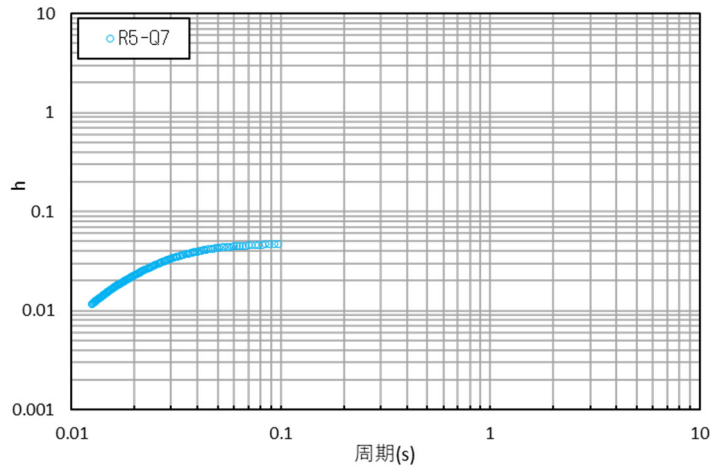
参考 1-3-15 図 コリレーション波形と減衰定数 (R5-Q7 孔: 観測深度 GL-16m~-130m)
