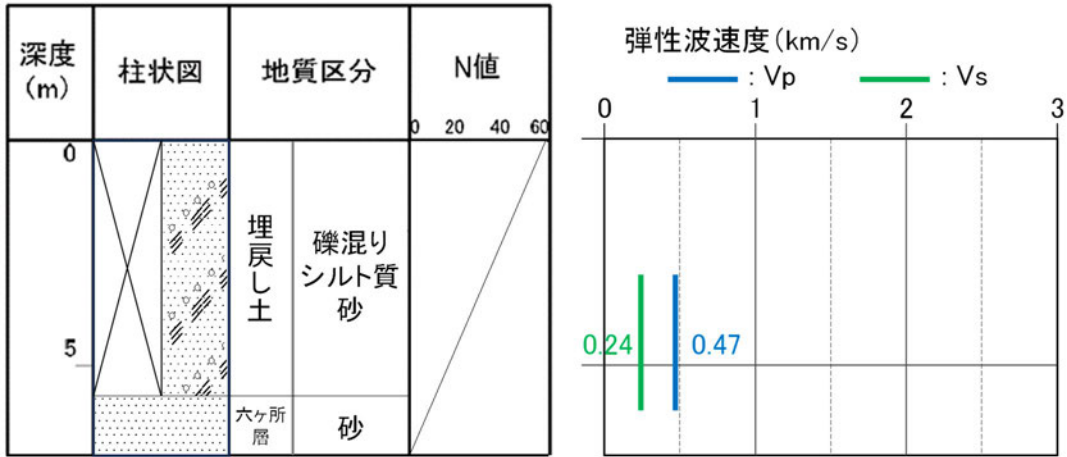
参考2-20図 ボーリング柱状図 (f1-5孔)
