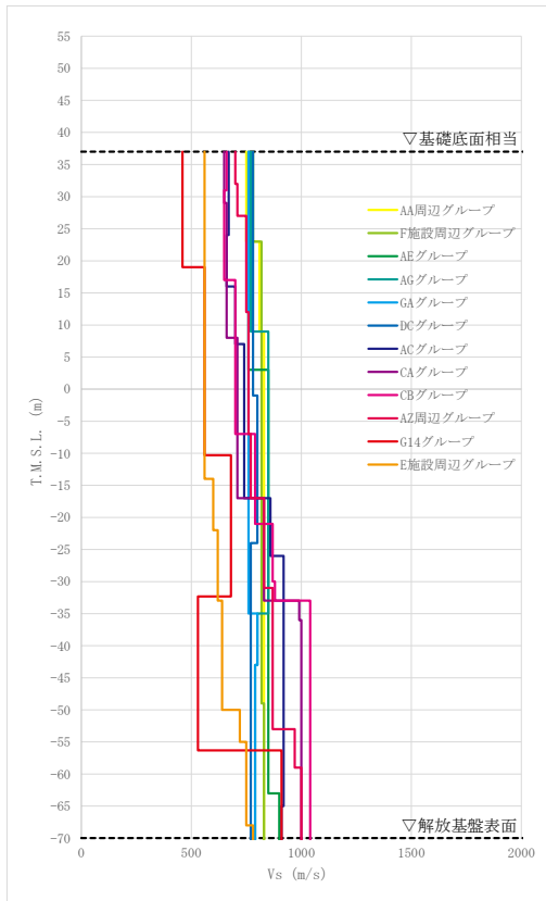
(a) S波速度
