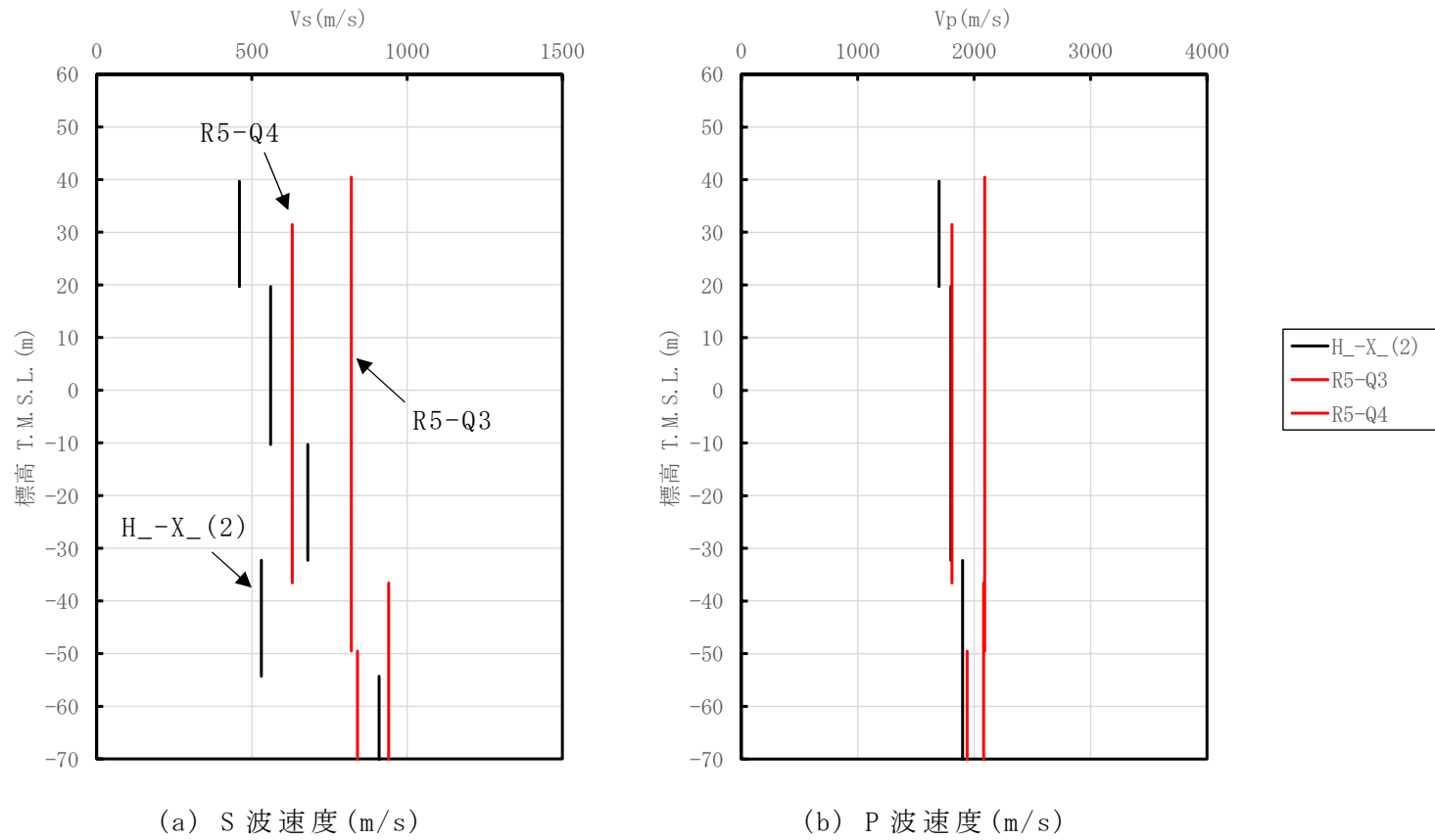
第 4.11-3 図 PS 検層結果の比較 (G14 グループ)
