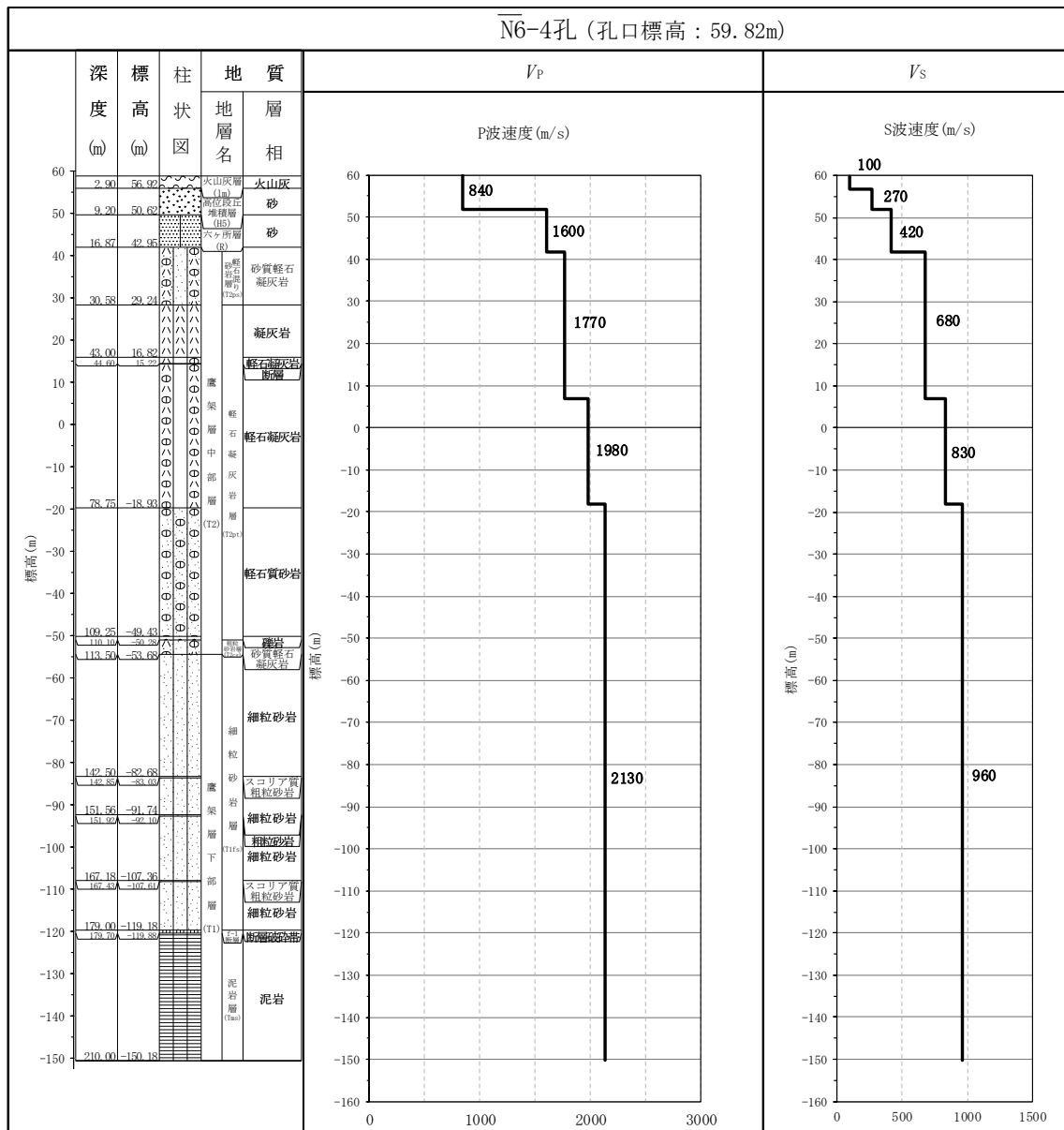
第 4.7-1 図 PS 検層結果 (AC グループ) (1/4)
