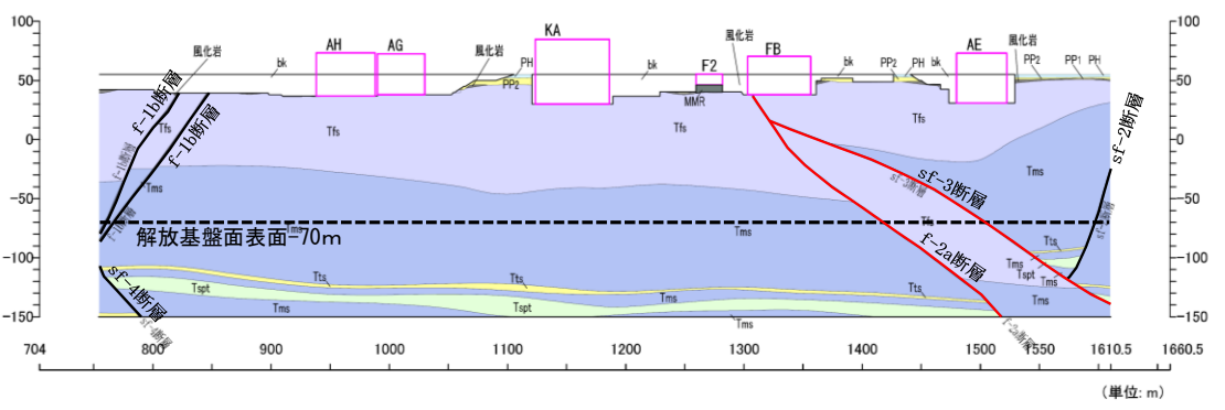
第3-2図 岩盤分類図 (NS5断面) (5/35)
