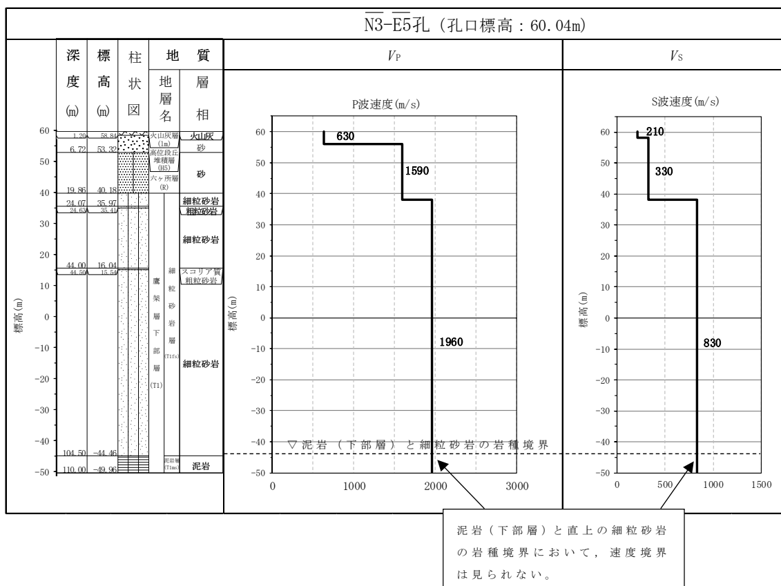
第 4.1-1 図 PS 検層結果 (AA 周辺グループ) (3/9)
