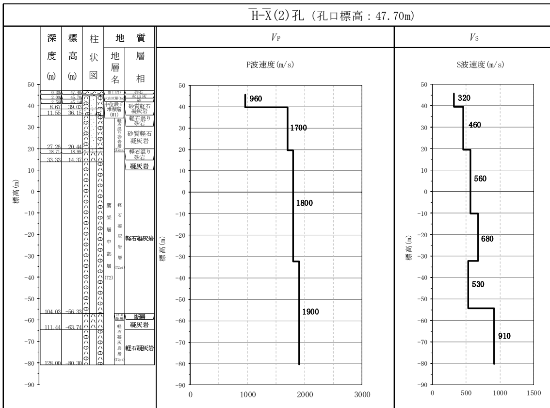
第 4.11-1 図 PS 検層結果 (G14 グループ) (1/3)
