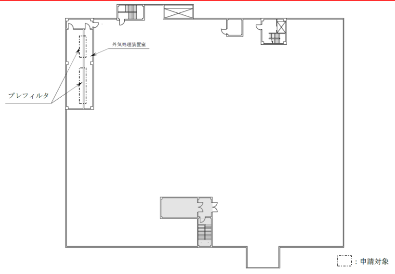
減容処理棟（屋上階）プレフィルタ据付場所
