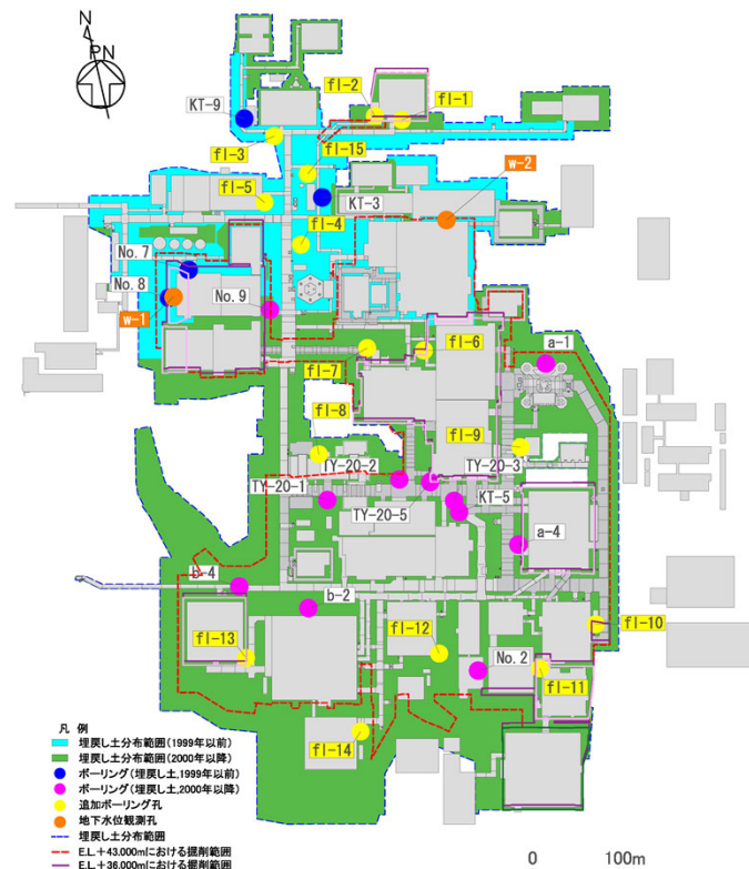
PS検層データ取得位置図
