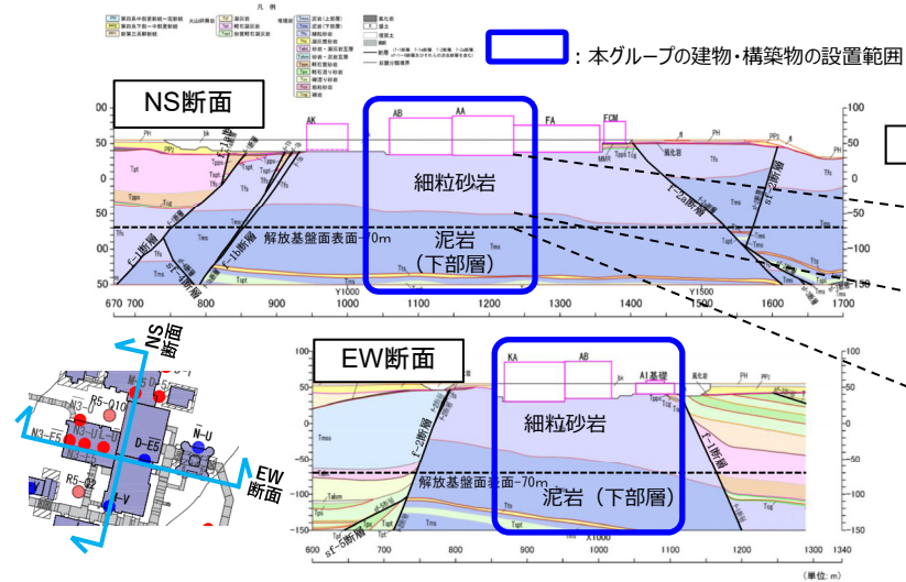
AA周辺グループの地下構造
