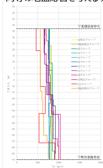
速度構造の比較 (S波速度)
