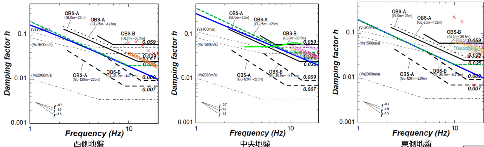
手法間の減衰定数の差（材料減衰 + 散乱減衰）
