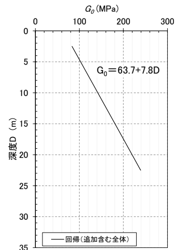
図(a) 埋戻し土の物性値
