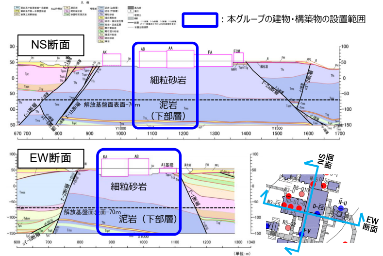
岩盤分類図
