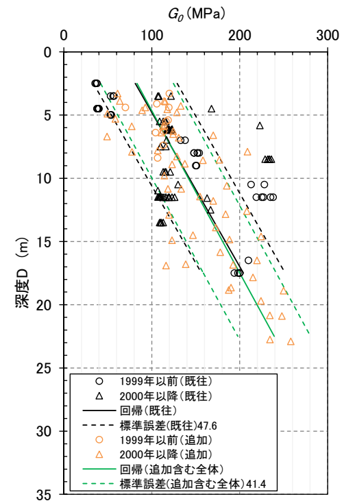
施工年代別の埋戻し土の動せん断弾性係数 G_0
