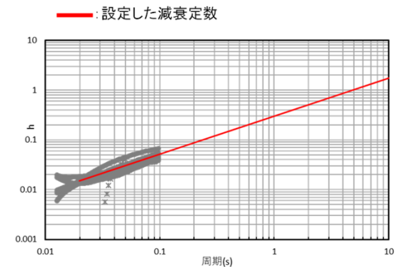
図(b) 岩盤部分の減衰定数
