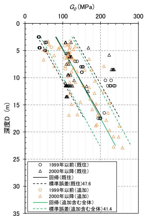
第 3.4-2 図 G_0 分布(全 30 孔)
