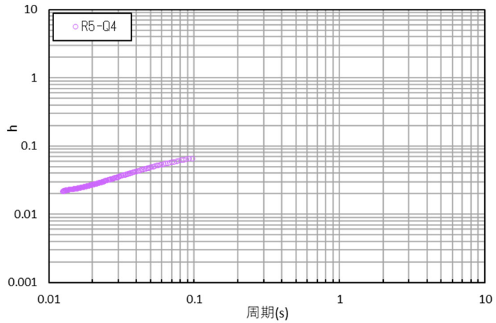
参考 1-3-19 図 コリレーション波形と減衰定数 (R5-Q4 孔: 観測深度 GL-14m~-130m)
