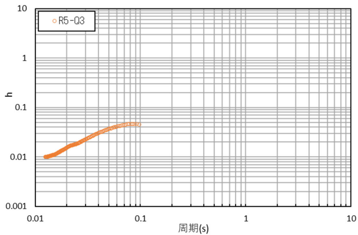
参考 1-3-18 図 コリレーション波形と減衰定数 (R5-Q3 孔: 観測深度 GL-8m~-130m)
