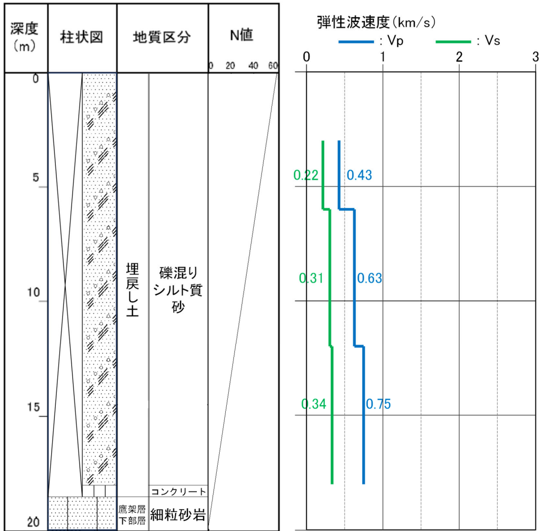
参考2-22図 ボーリング柱状図 (f1-7孔)
