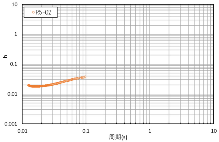
参考 1-3-17 図 コリレーション波形と減衰定数 (R5-Q2 孔: 観測深度 GL-12m~-130m)
