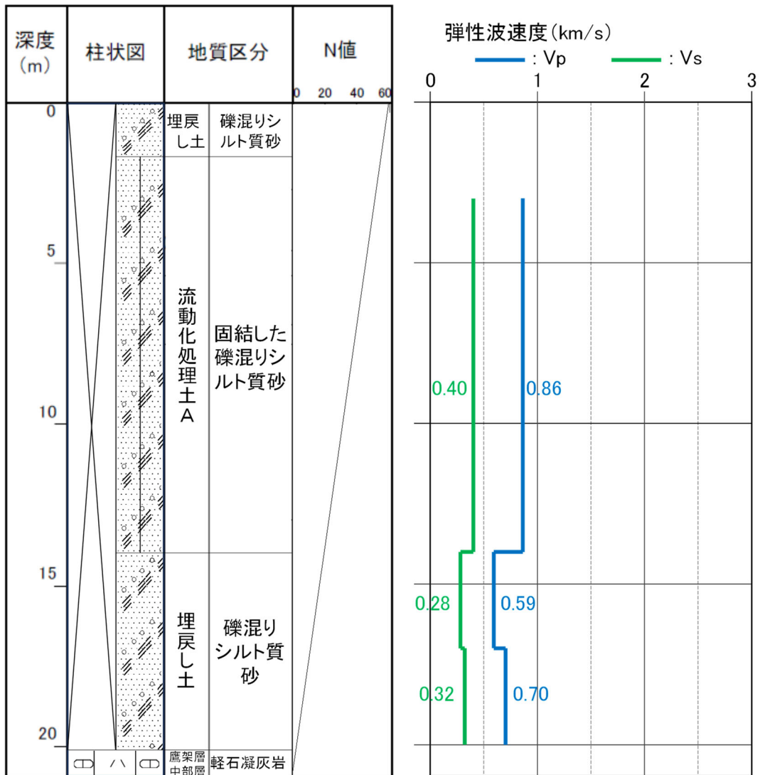
参考2-26図 ボーリング柱状図 (f1-11孔)
