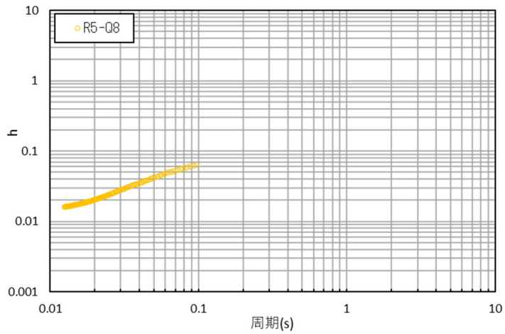
参考 1-3-23 図 コリレーション波形と減衰定数 (R5-Q8 孔: 観測深度 GL-30m~-130m)
