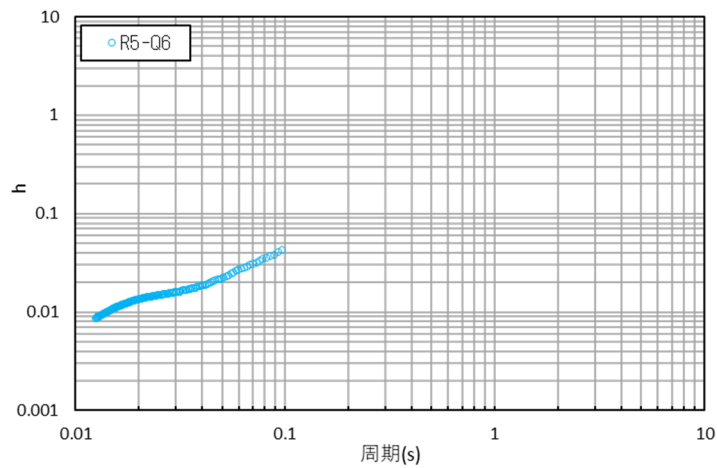
参考 1-3-21 図 コリレーション波形と減衰定数 (R5-Q6 孔: 観測深度 GL-8m~-130m)
