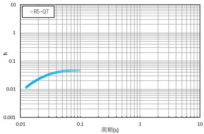
参考 1-3-22 図 コリレーション波形と減衰定数 (R5-Q7 孔: 観測深度 GL-16m~-130m)
