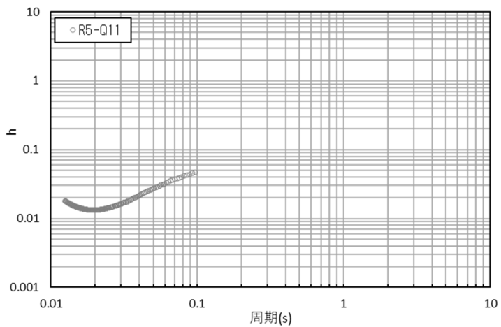
参考 1-3-26 図 コリレーション波形と減衰定数 (R5-Q11 孔: 観測深度 GL-12m~-130m)
