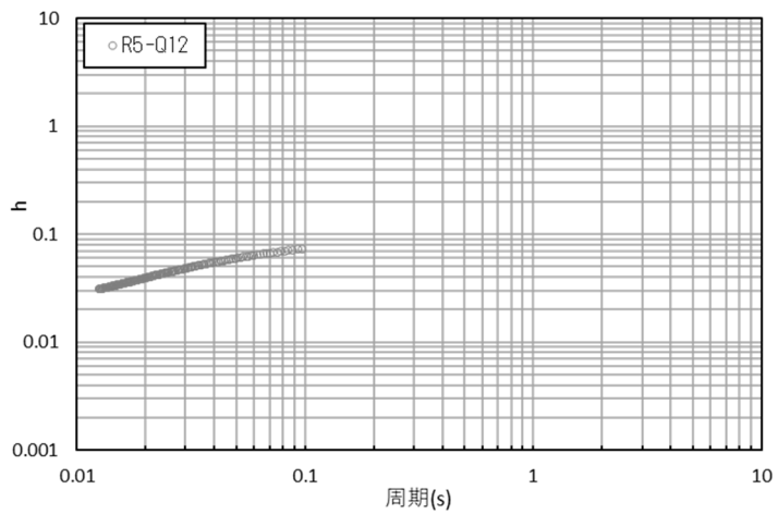
参考 1-3-27 図 コリレーション波形と減衰定数 (R5-Q12 孔: 観測深度 GL-12m~130m)
