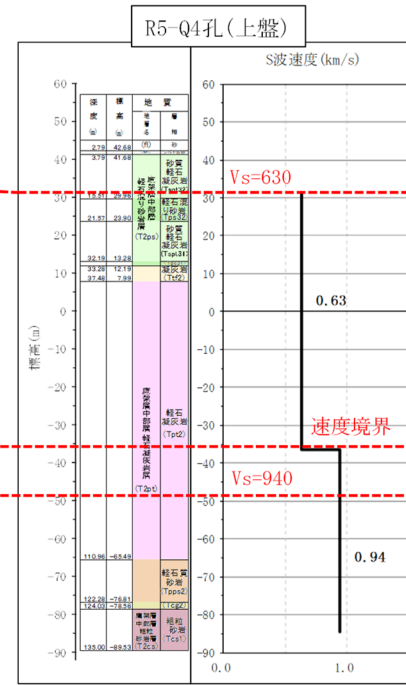
第 3.5-2 図 G14 建屋において選定した PS 検層結果による層境界レベルの補正の結果 (2/4)
