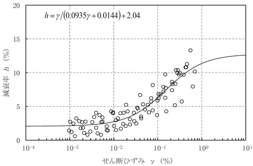
第 4.1-6 図 ひずみ依存特性 (砂岩・凝灰岩互層)
