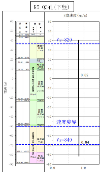
第 3.5-2 図 G14 建屋において選定した PS 検層結果による層境界レベルの補正の結果 (4/4)
