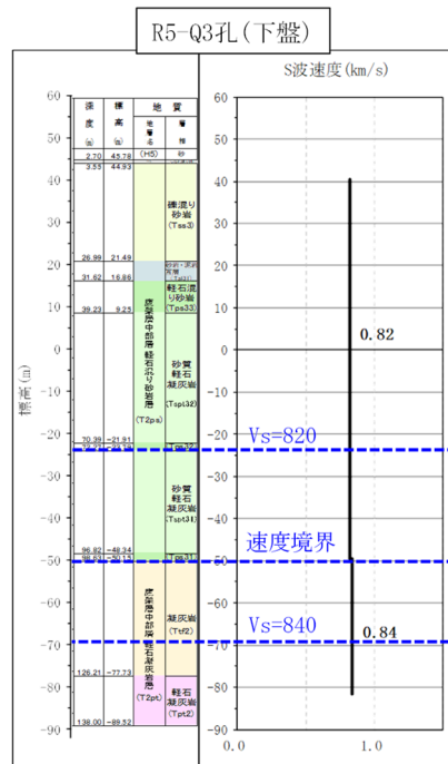
第3.5-2図 G14 建屋において選定したPS検層結果による層境界レベルの補正の結果 (1/4)
