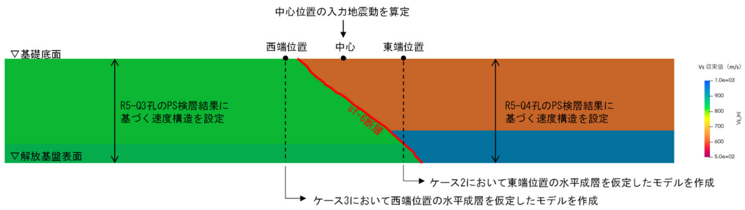
第 2.2-1 図 解析モデルの速度構造 (ケース 1)
