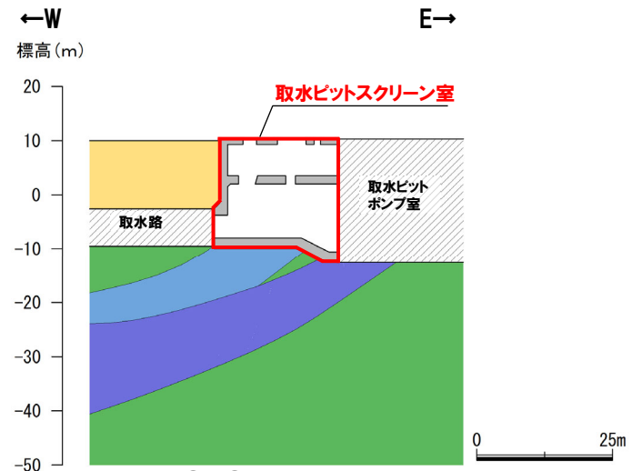
⑭-⑭'断面
