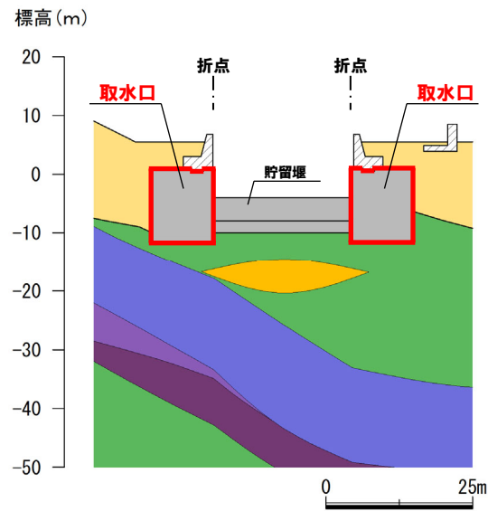
②①-②①' 断面
