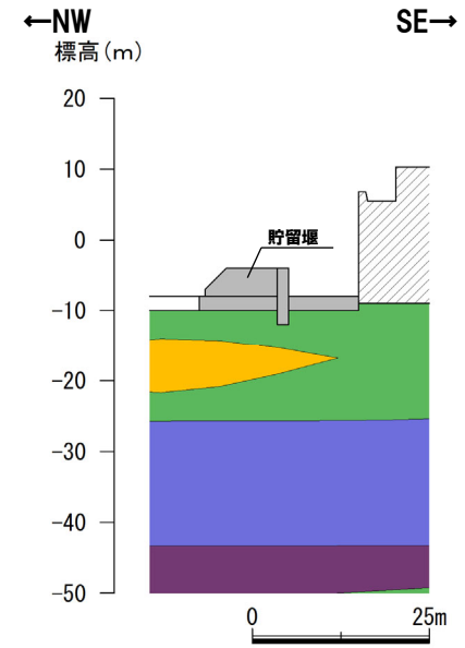
②①-②①' 断面
