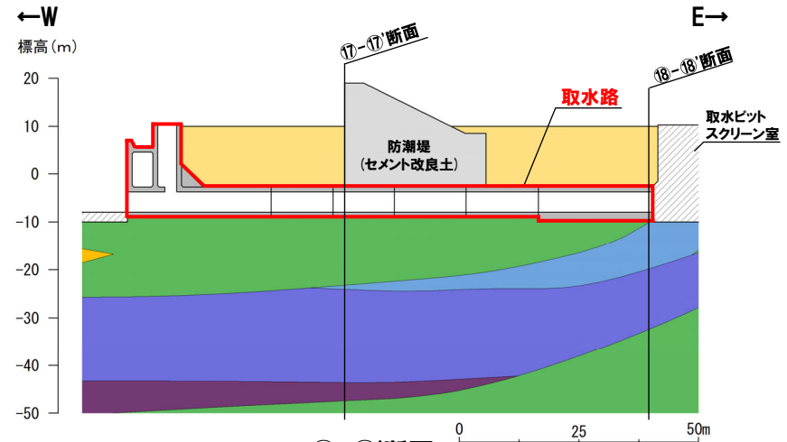
19-19' 断面
