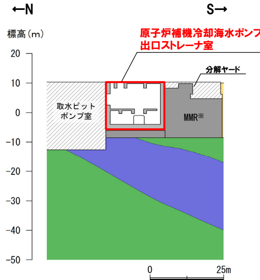
⑨-⑨'断面
