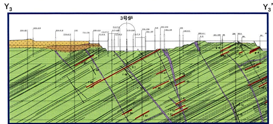
地質鉛直断面図 (Y 3 -Y 3 ' 断面)
