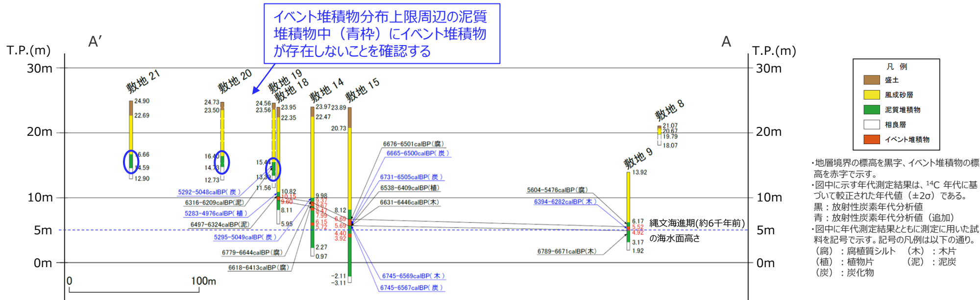
地質断面図
