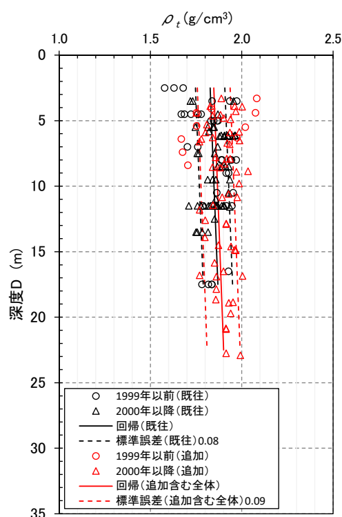
第 3.4-1 図 湿潤密度分布(全 30 孔)
