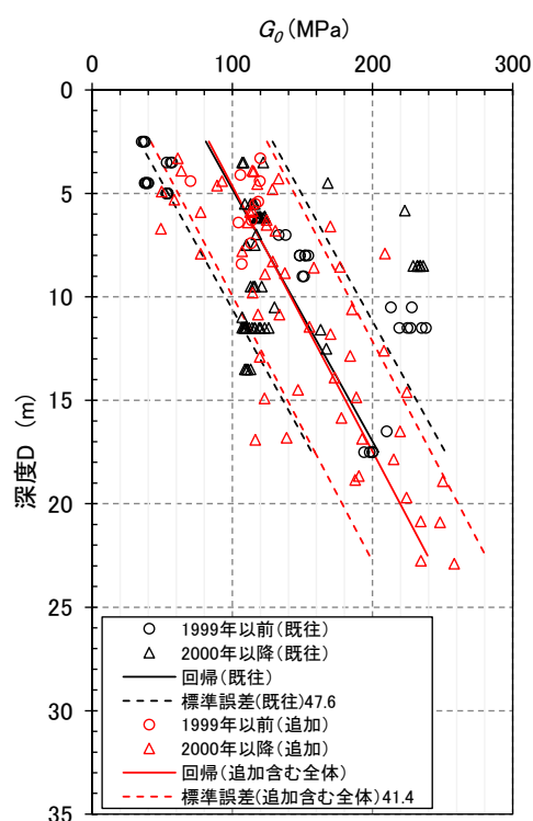
第 3.4-2 図 G_0 分布(全 30 孔)
