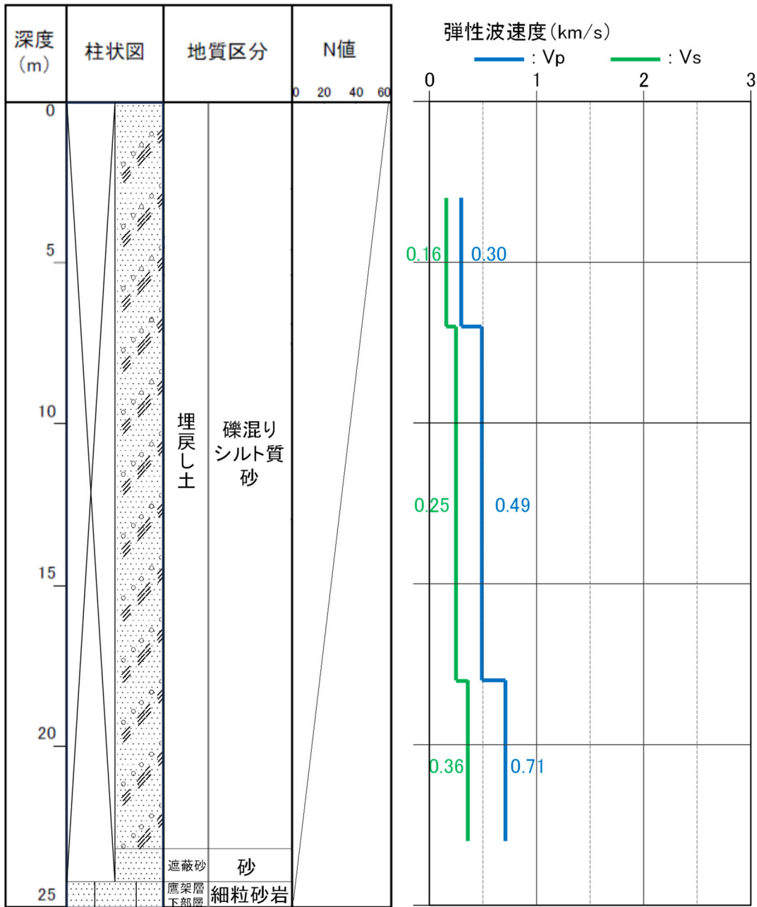
参考2-16図 ボーリング柱状図 (f1-1孔)
