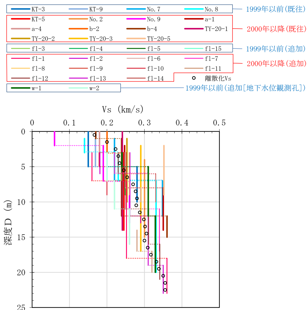
第 3.4-3 図 ボーリング柱状図による V_s と離散化 V_s (全 32 孔)
