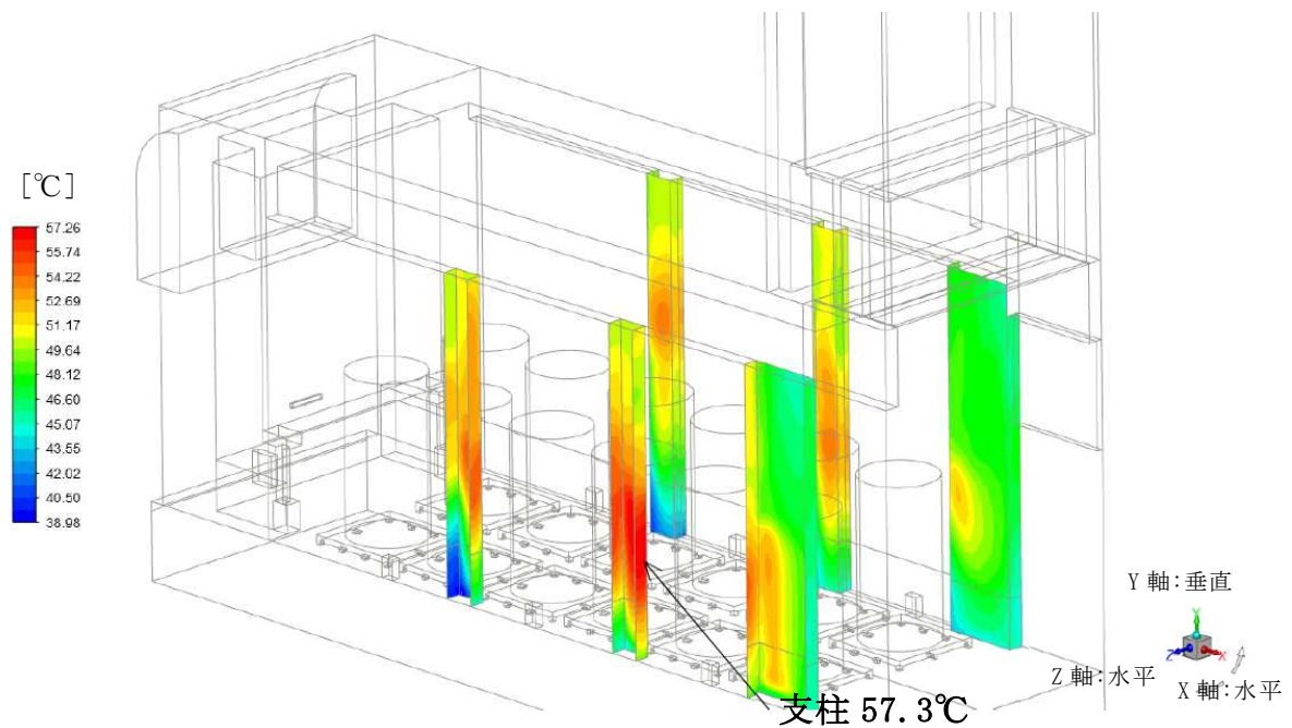
第 12-3 図 支柱表面温度分布 (PWR用キャスク(タイプ1))
