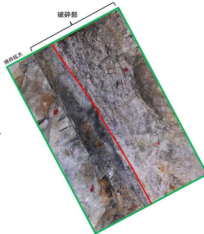
H-3c破碎帯
