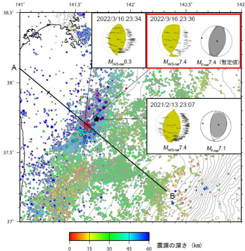
第1図. 観測点補正值による再決定震源の分布。2022年3月16日から17日7時までの地震を赤色アウトラインのシンボルで示す。また、2017年1月1日から2022年3月10日までの地震を灰色アウトラインのシンボルで、特にそのうち2021年2月13日から14日までの地震を黒色アウトラインのシンボルでそれぞれ示す。シンボル内の色は地震の深さを表す。防災科研によるルーチン処理震源カタログ(S-net記録使用、手動検測)の検測値に観測点補正值[浅野(2021)]を加えて再決定した。主要な地震を星印で示し、Hi-net/S-netによる初動解とF-net MT解を併せて示す。測線ABは第2図における鉛直断面の水平位置を表す。
