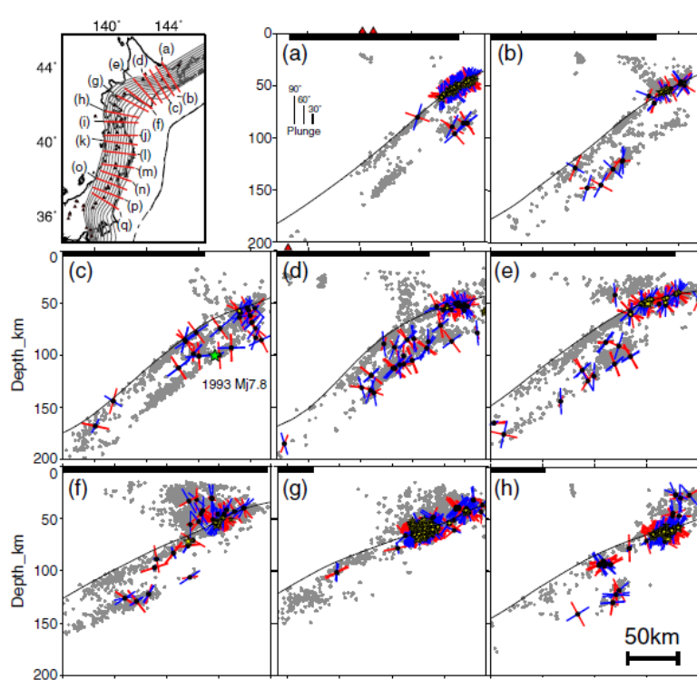
●: 各断面から10km以内で発生した地震, 青線:T軸, 赤線:P軸, ☆: 繰返し地震, ●: プレート境界で発生した低角逆断層地震, 黒線: プレート上面
