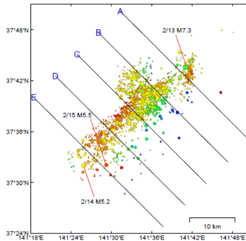
震央分布
