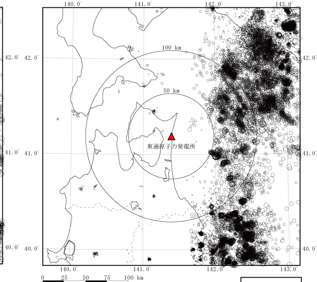
震源深さ 30～60km
