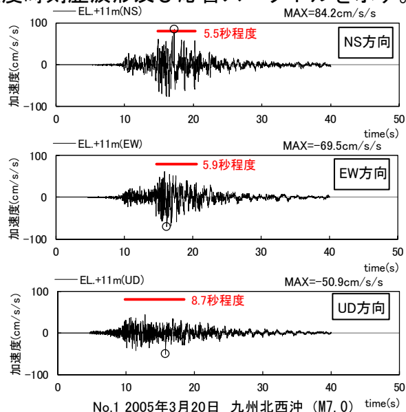
No.1 2005年3月20日 九州北西沖 (M7.0)
