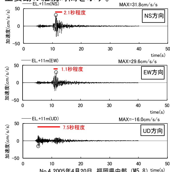
No.4 2005年4月20日 福岡県中部 (M5.8)
