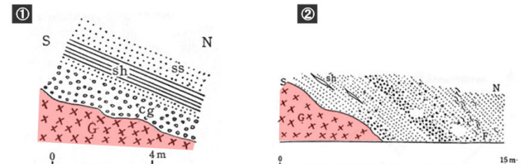
第3図 妻村日坂露頭 第5図 打上村中平露頭 ss: 砂岩 sh: 頁岩 cg: 礫岩 G: 花崗岩 F: 貝化石 sh: 頁岩 G: 花崗岩
