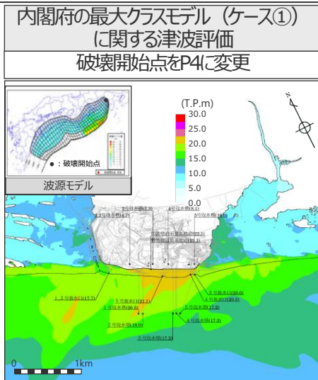
最大上昇水位分布 敷地前面
