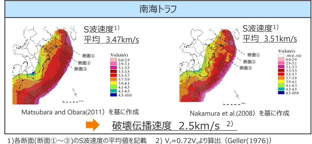
沈み込み帯のS波速度構造と、S波速度構造から推定される破壊伝播速度
