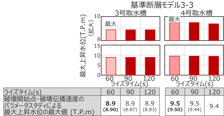
水位上昇側：取水槽のパラメータスタディ因子の影響確認 (基準断層モデル3-1~3-3)
