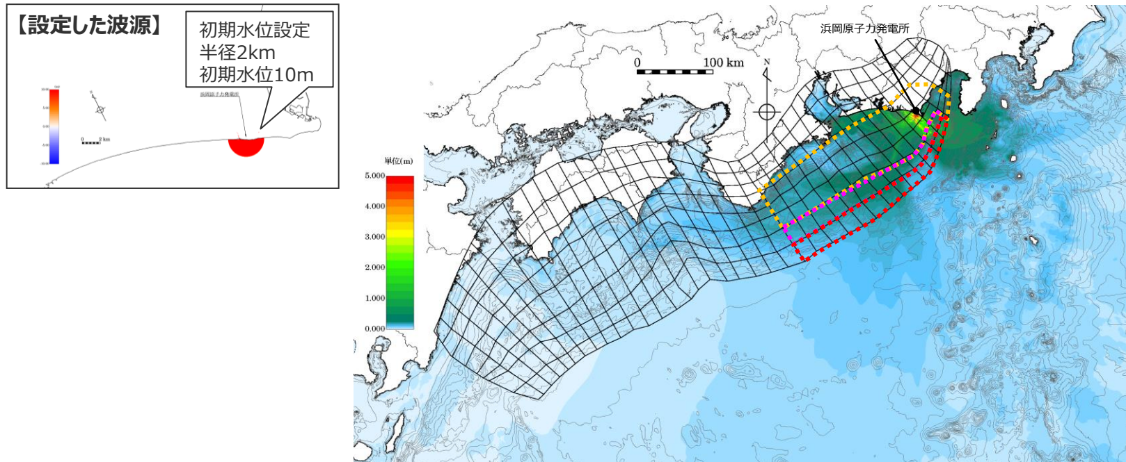
南海トラフ周辺の最大水位上昇量
