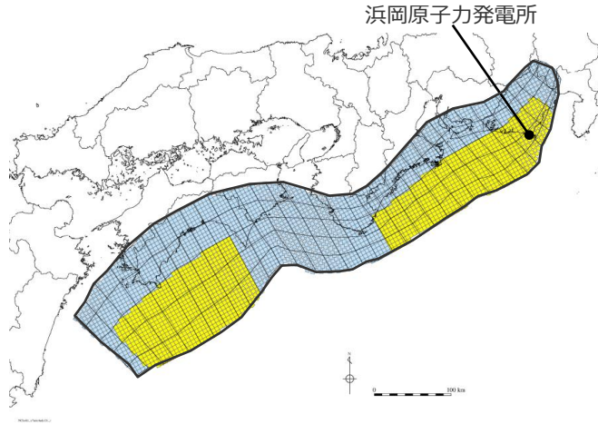
既往最大地震の津波痕跡再現モデル
