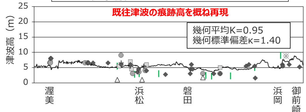
遠州灘沿岸域の5地震の津波痕跡再現モデル（特性化モデル）による海岸線の津波高と既往津波の痕跡高との比較
