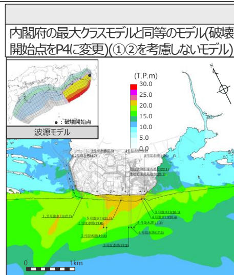
最大上昇水位分布 敷地前面
