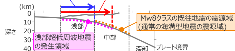
超大すべり域の設定深さと南海トラフの地震学的知見との関係
