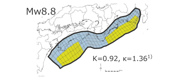
既往最大地震の津波痕跡再現モデル
