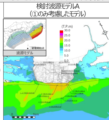
最大上昇水位分布 敷地前面
