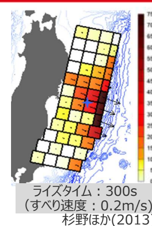
2011年東北沖地震
