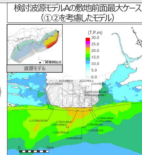
最大上昇水位分布 敷地前面
