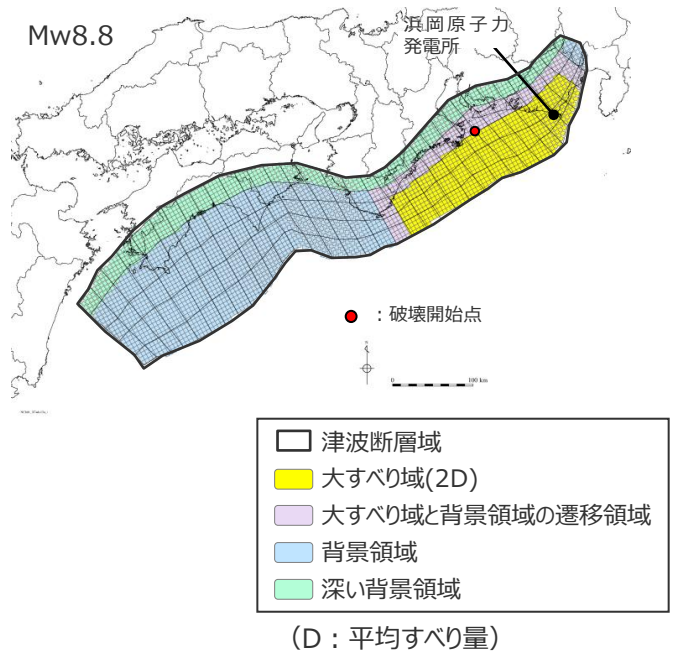
遠州灘沿岸域の5地震の津波痕跡再現モデル (特性化モデル)
