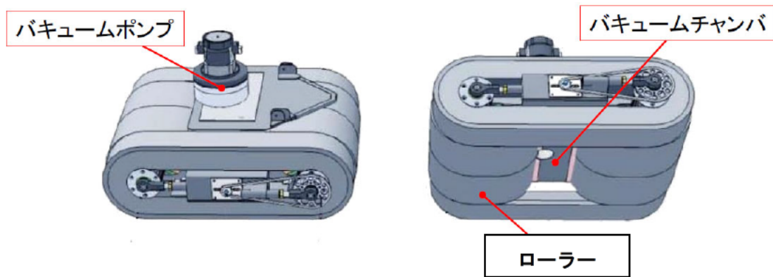
図3. 5 点検装置（壁面走行ロボット）本体イメージ図
