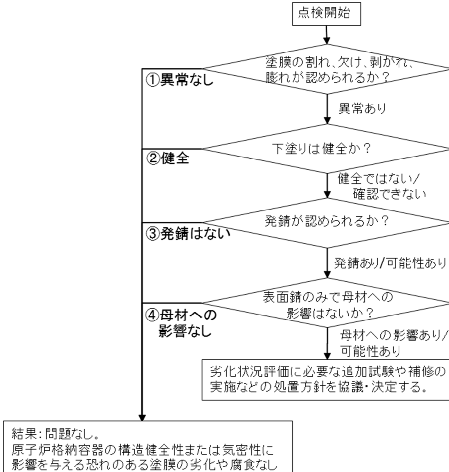
図3. 1 2 点検フロー
