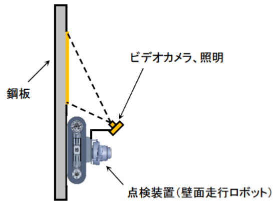
図3. 4 点検装置（壁面走行ロボット）イメージ図
