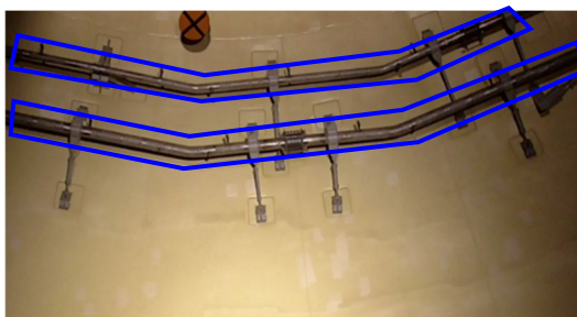
図3. 10 従来の点検で確認が容易でない範囲の例（内面高所の干渉物裏） （高浜4号炉の写真）
