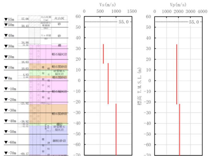
(a)地質柱状図 (b)S波速度 (c)P波速度 PS検層から得られたデータ (D-3孔)
