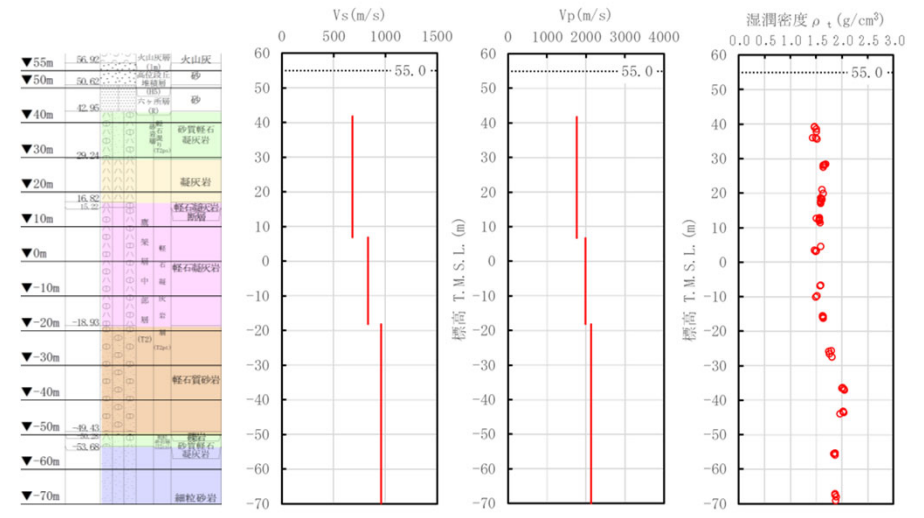
(a)地質柱状図 (b)S波速度 (c)P波速度 (d)単位体積重量 PS検層から得られたデータ (N6_-4孔)
