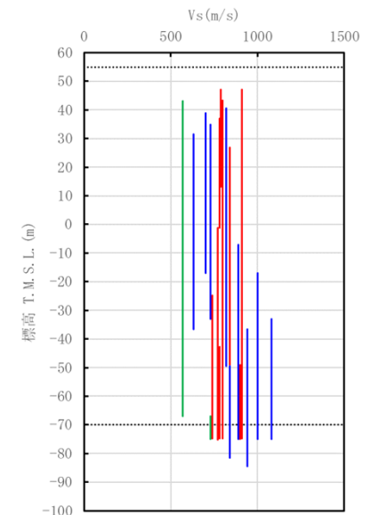
S波検層実施地点の速度構造
