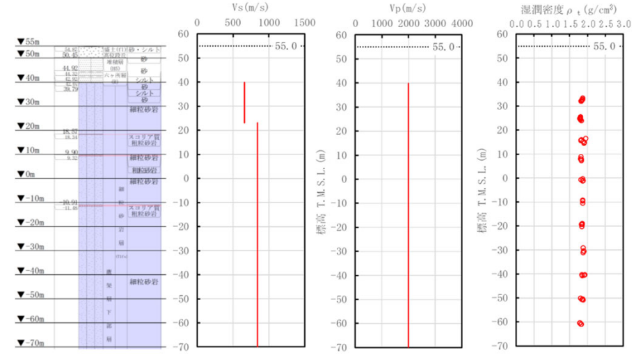
(a)地質柱状図 (b)S波速度 (c)P波速度 (d)単位体積重量 PS検層から得られたデータ (N-U孔)
