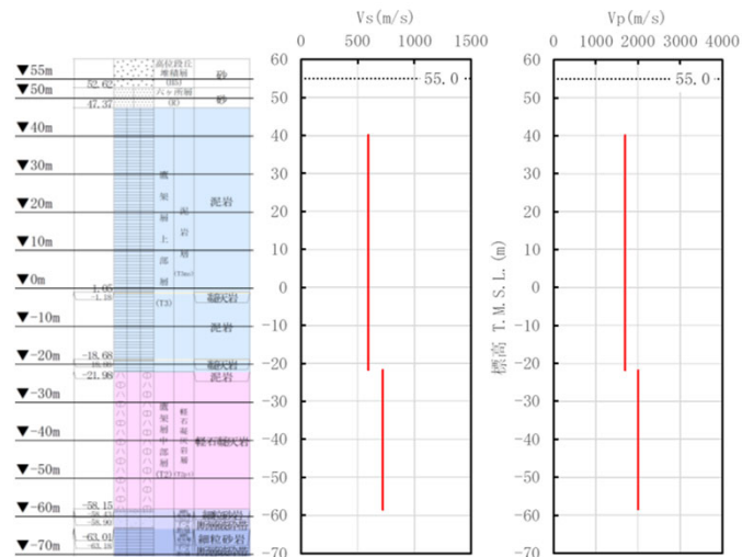
(a)地質柱状図 (b)S波速度 (c)P波速度 PS検層から得られたデータ (K-T孔)
