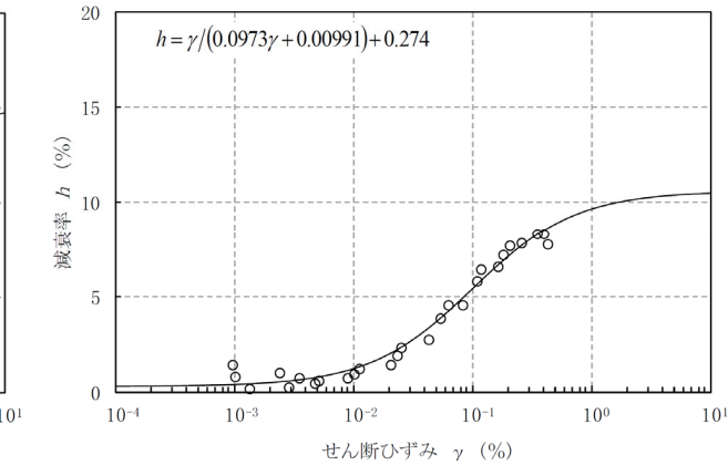
礫岩
