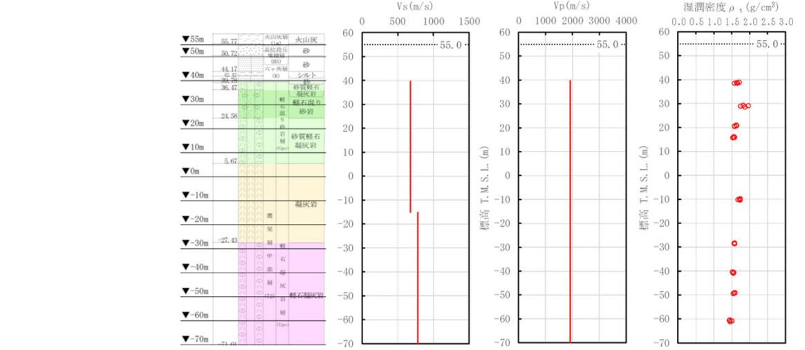
(a)地質柱状図 (b)S波速度 (c)P波速度 (d)単位体積重量 PS検層から得られたデータ (O-E5孔)
