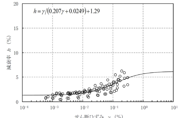
細粒砂岩
