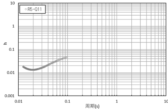
コリレーション波形と減衰定数(R5-Q11孔:観測深度GL-16m~-130m)
