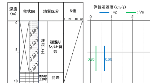
fl-15 (孔口標高 55.04m)
