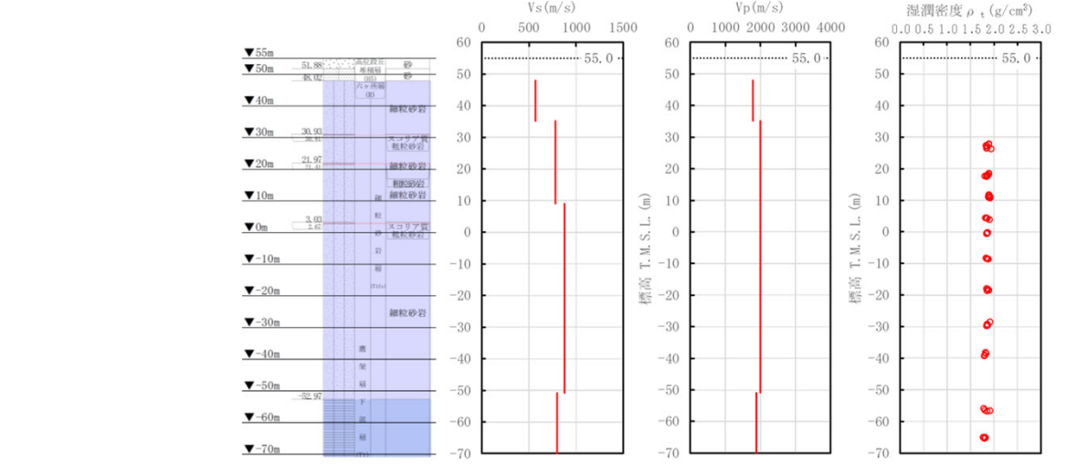
(a)地質柱状図 (b)S波速度 (c)P波速度 (d)単位体積重量 PS検層から得られたデータ (D-E5_孔)
