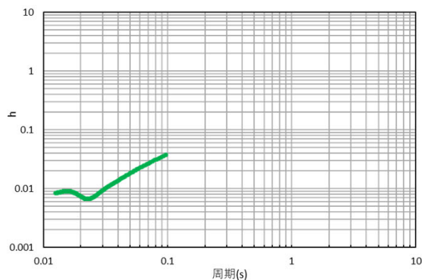
西側地盤
