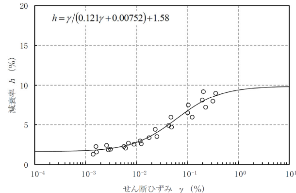
粗粒砂岩
