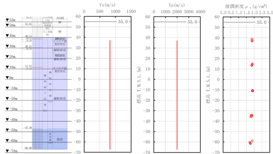
(a)地質柱状図 (b)S波速度 (c)P波速度 (d)単位体積重量 PS検層から得られたデータ (M-V孔)
