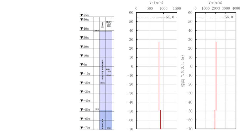
(a)地質柱状図 (b)S波速度 (c)P波速度 (d)単位体積重量 PS検層から得られたデータ (R5-Q10孔)
