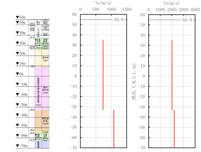
(a)地質柱状図 (b)S波速度 (c)P波速度 (d)単位体積重量 PS検層から得られたデータ（R5-Q12孔）
