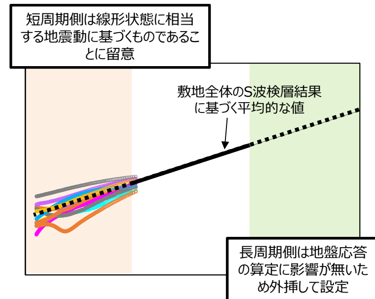
敷地の地盤の特徴を捉えた減衰定数の設定イメージ
