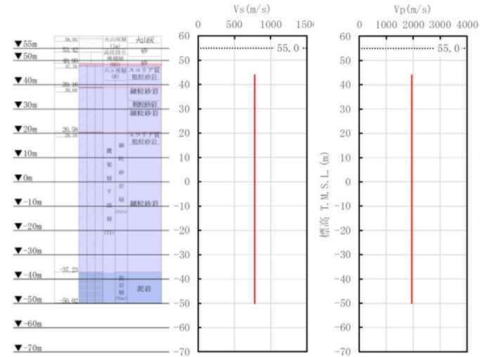
(a)地質柱状図 (b)S波速度 (c)P波速度 (d)単位体積重量 PS検層から得られたデータ (N3-E5_孔)
