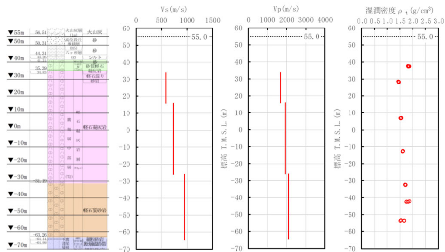
(a)地質柱状図 (b)S波速度 (c)P波速度 (d)単位体積重量 PS検層から得られたデータ (N6-V孔)
