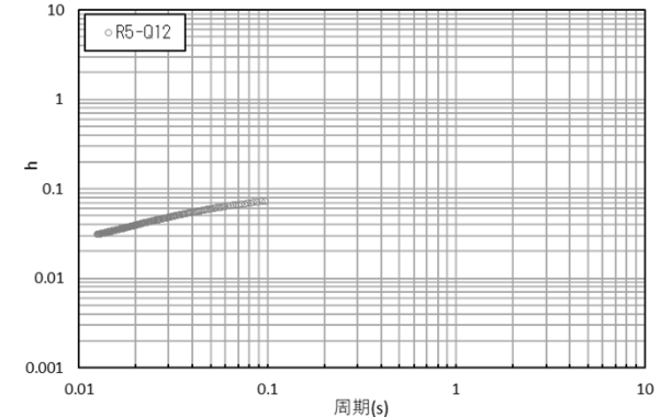
コリレーション波形と減衰定数(R5-Q12孔:観測深度GL-20m~-130m)
