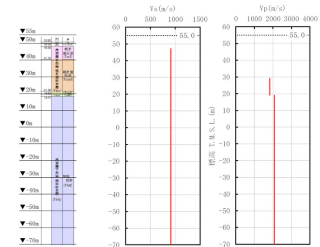
(a)地質柱状図 (b)S波速度 (c)P波速度 (d)単位体積重量 PS検層から得られたデータ (R5-Q9孔)
