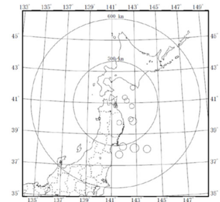
震央分布図
