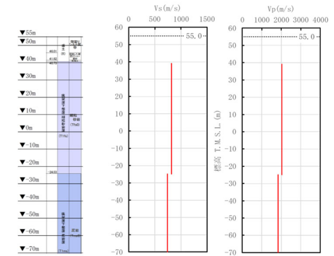
(a)地質柱状図 (b)S波速度 (c)P波速度 PS検層から得られたデータ（R5-Q11孔）
