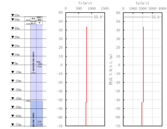
PS検層から得られたデータ (R5-Q2孔)
