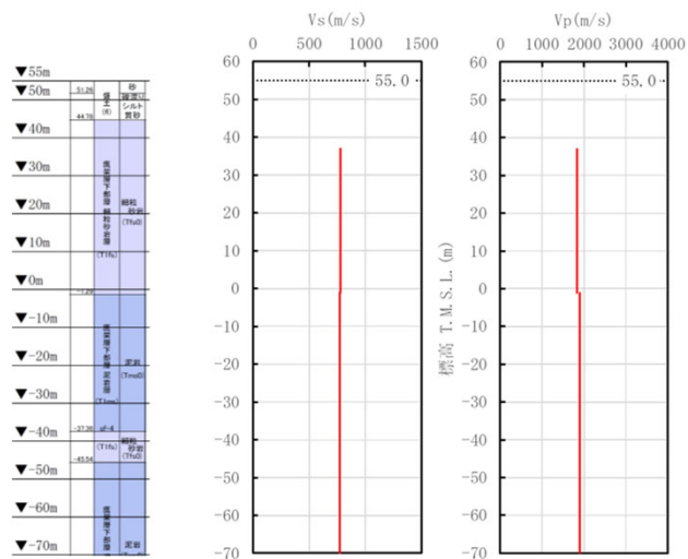
PS検層から得られたデータ (R5-Q1孔)
