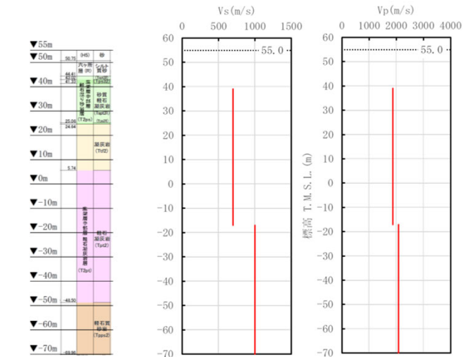
(a)地質柱状図 (b)S波速度 (c)P波速度 (d)単位体積重量 PS検層から得られたデータ (R5-Q7孔)
