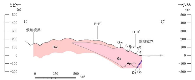
C-C' 断面図
