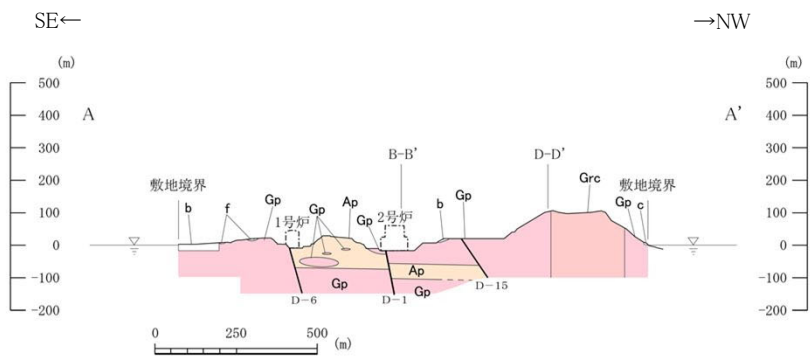
A-A' 断面図
