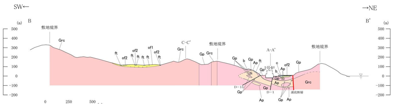
B-B' 断面図
