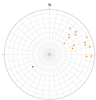
シュミットネット (下半球投影) ● せん断面 (K断層) : 16 ● 断層面 : 1
