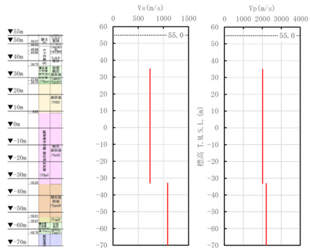
(a)地質柱状図 (b)S波速度 (c)P波速度 (d)単位体積重量 PS検層から得られたデータ (R5-Q12孔)
