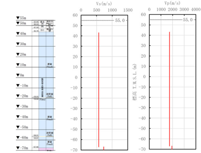
(a)地質柱状図 (b)S波速度 (c)P波速度 PS検層から得られたデータ (R5-Q5孔)
