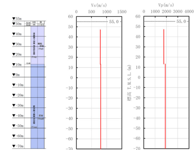
(a)地質柱状図 (b)S波速度 (c)P波速度 PS検層から得られたデータ (R5-Q6孔)
