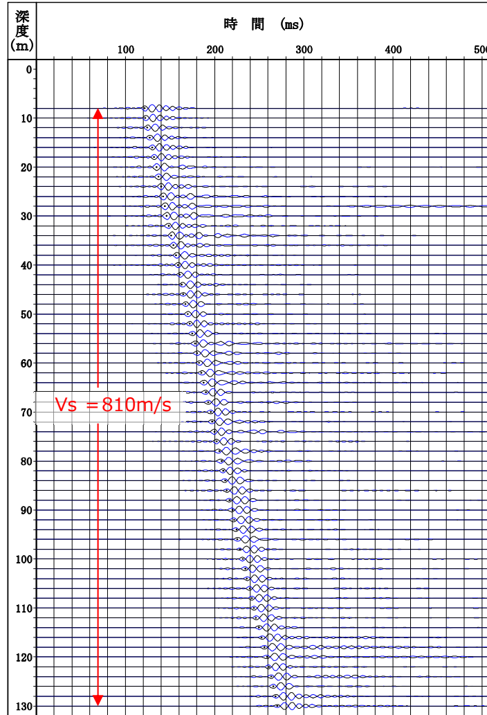
相対振幅と観測波形(コリレーション処理後：R5-Q6孔の例)
