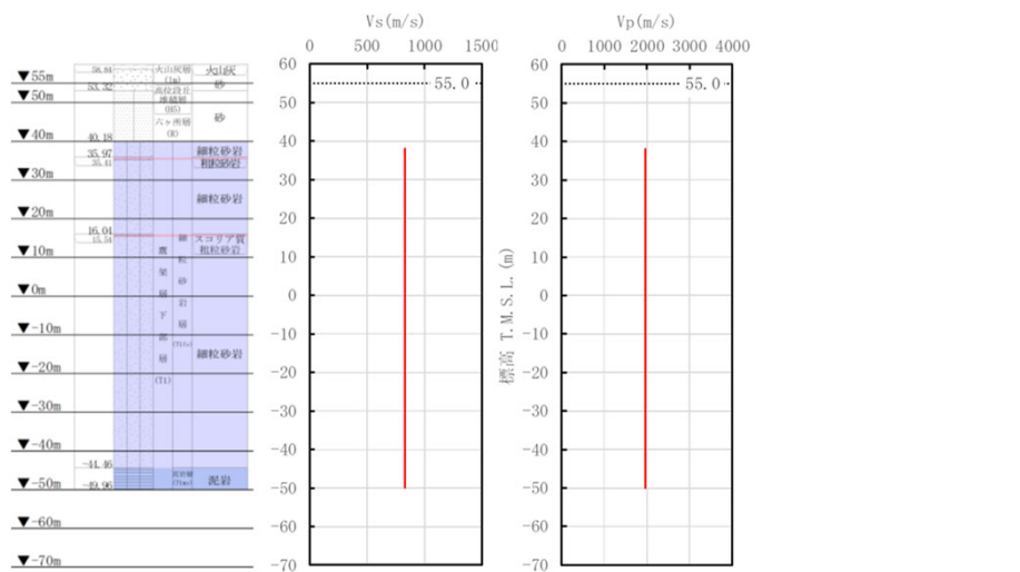
(a)地質柱状図 (b)S波速度 (c)P波速度 PS検層から得られたデータ (N3-E5_孔)
