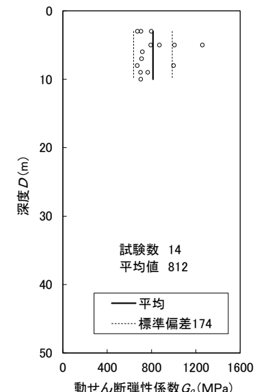
第2グループ ( q_u \geq 0.6\text{MPa} )
