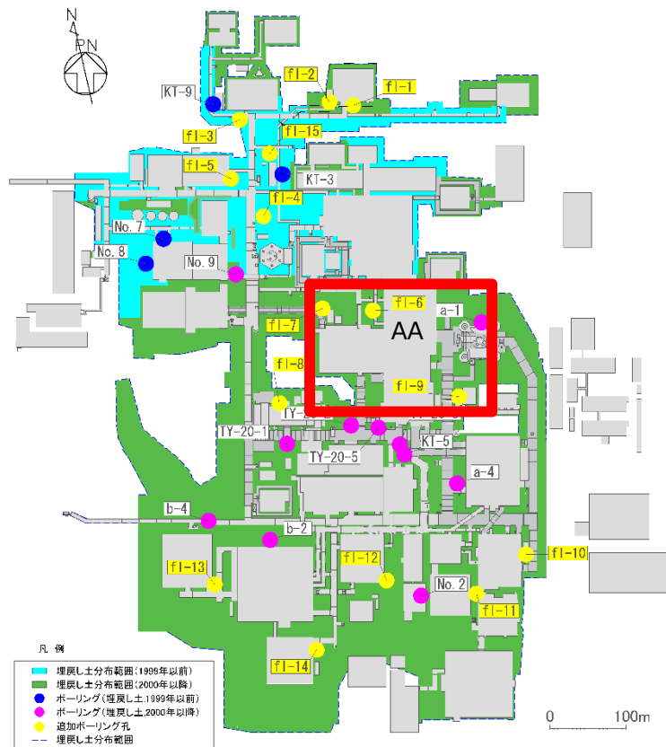
AA周辺の埋戻し土分布位置図
