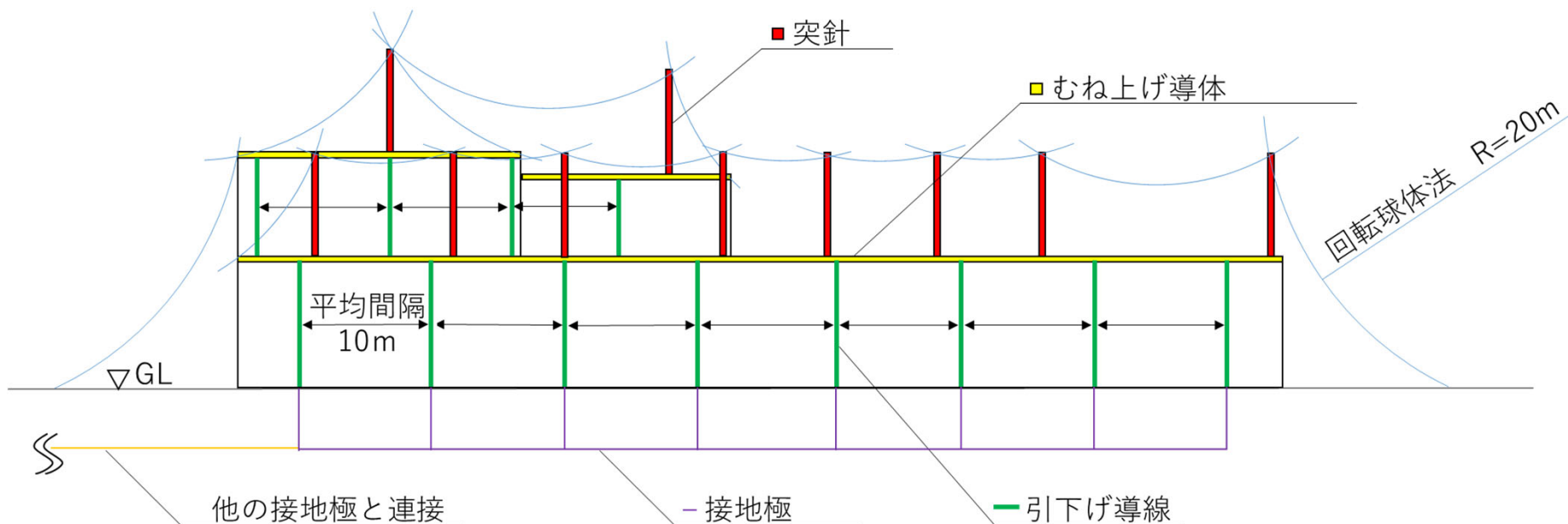
<緊急時対策建屋 避雷設備 概要図>
