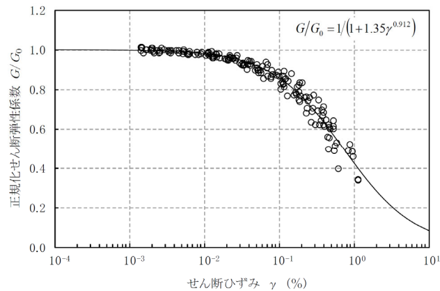
泥岩 (上部層)
