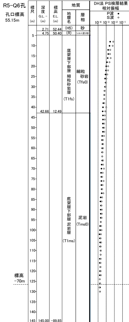
相対振幅と観測波形(コリレーション処理後：R5-Q6孔の例)
