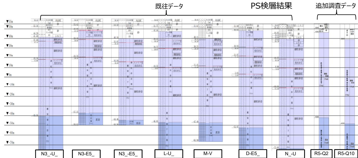
地質柱状図の比較
