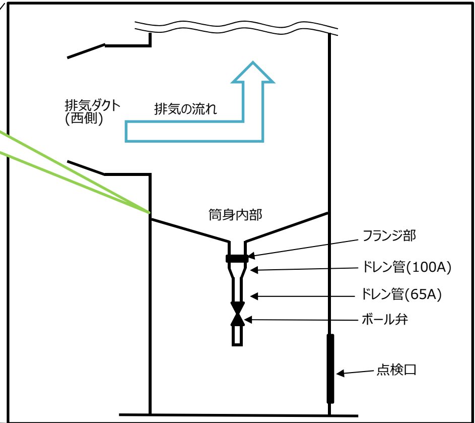
主排気筒の底部の拡大図
