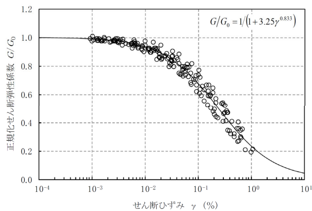
礫混り砂岩
