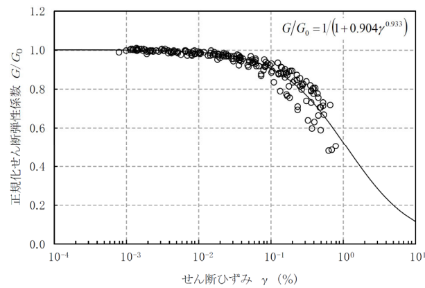
泥岩 (下部層)
