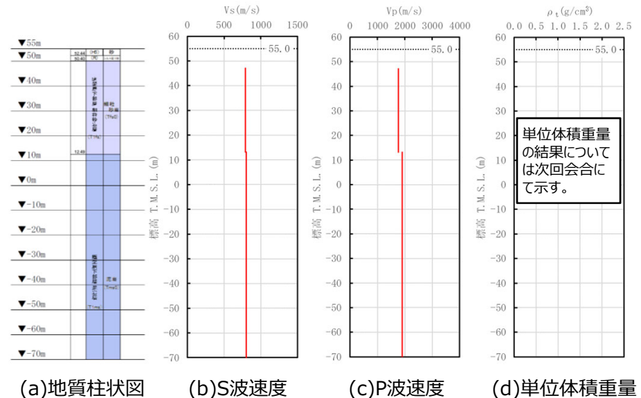
(a)地質柱状図 (b)S波速度 (c)P波速度 (d)単位体積重量 PS検層から得られたデータ（R5-Q6孔の例）
