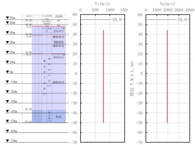
(a)地質柱状図 (b)S波速度 (c)P波速度 PS検層から得られたデータ (N3-E5_孔)
