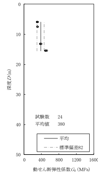
第1グループ ( q_u \geq 0.2 \sim 0.3\text{MPa} )
