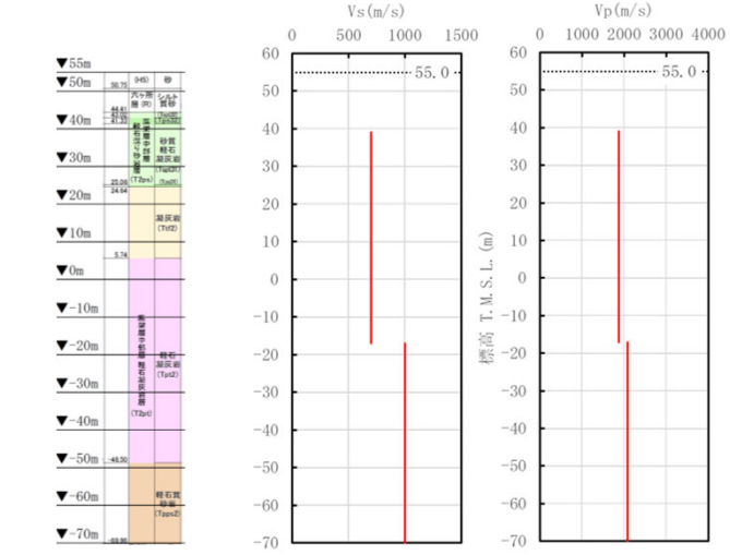
(a)地質柱状図 (b)S波速度 (c)P波速度 PS検層から得られたデータ (R5-Q7孔)
