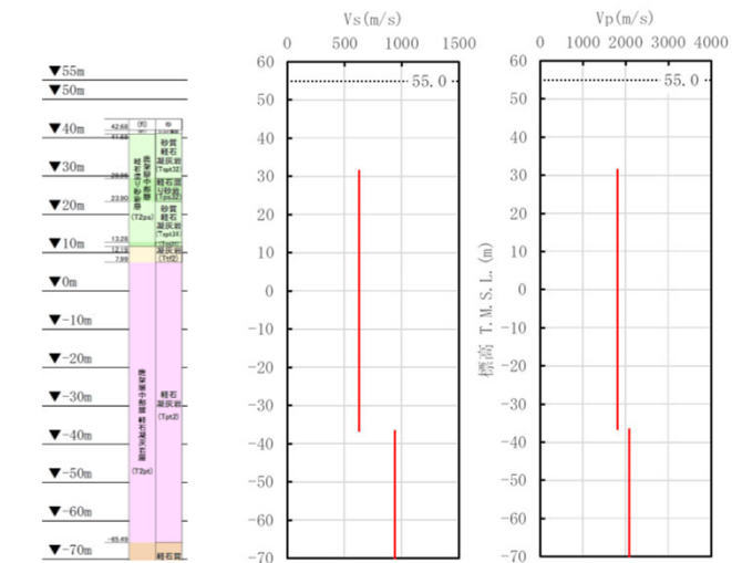
(a)地質柱状図 (b)S波速度 (c)P波速度 PS検層から得られたデータ (R5-Q4孔)
