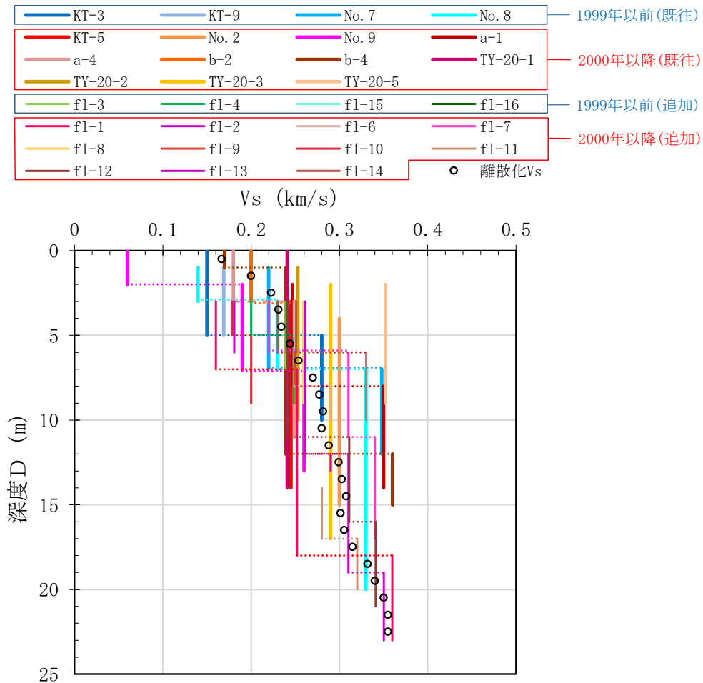
第 3.4-3 図 ボーリング柱状図による V_s と離散化 V_s (全 30 孔)
