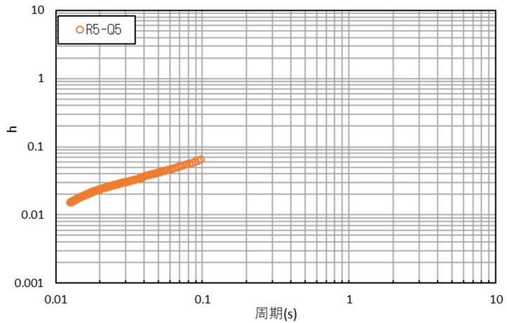
参考 1-3-20 図 コリレーション波形と減衰定数 (R5-Q5 孔: 観測深度 GL-18m~-130m)
