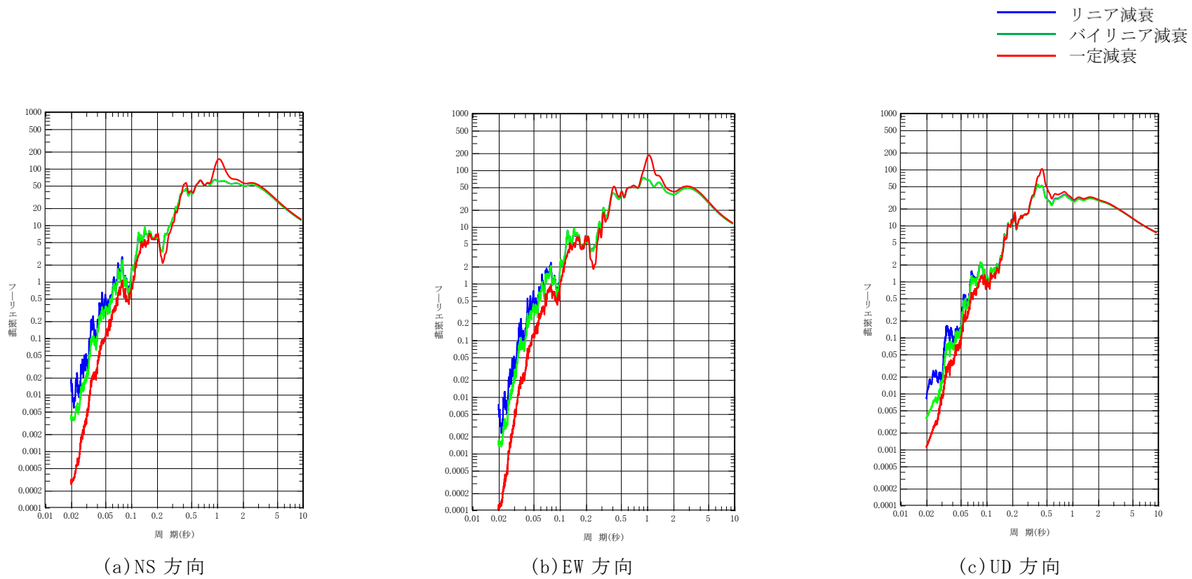
参考 3-3.2 図 地震観測記録のシミュレーション解析結果のフーリエスペクトル (西側地盤)
