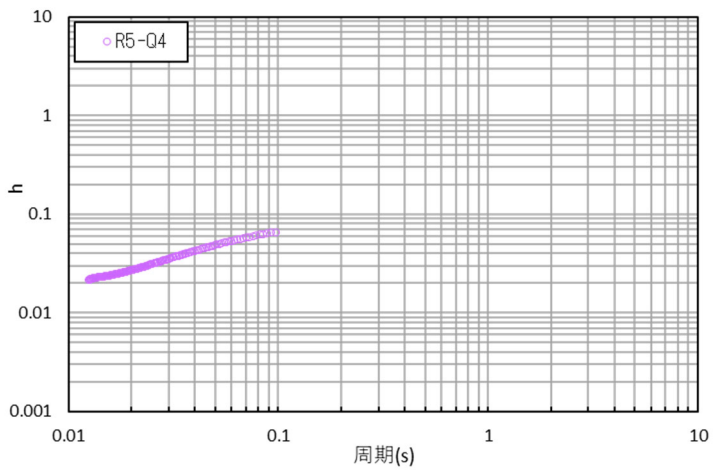
参考 1-3-19 図 コリレーション波形と減衰定数 (R5-Q4 孔: 観測深度 GL-18m~-130m)
