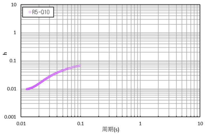
参考 1-3-25 図 コリレーション波形と減衰定数 (R5-Q10 孔: 観測深度 GL-18m~-130m)
