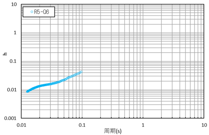
参考 1-3-21 図 コリレーション波形と減衰定数 (R5-Q6 孔: 観測深度 GL-18m~-130m)
