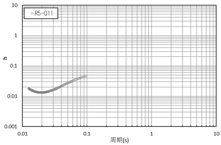
参考 1-3-26 図 コリレーション波形と減衰定数 (R5-Q11 孔: 観測深度 GL-18m~-130m)
