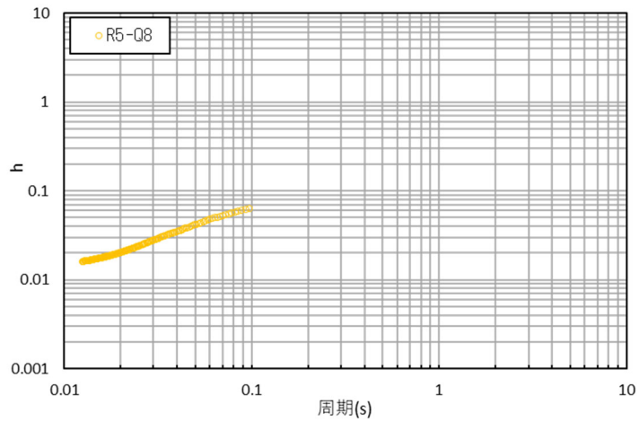
参考 1-3-23 図 コリレーション波形と減衰定数 (R5-Q8 孔: 観測深度 GL-18m~-130m)
