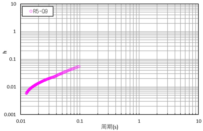
参考 1-3-24 図 コリレーション波形と減衰定数
