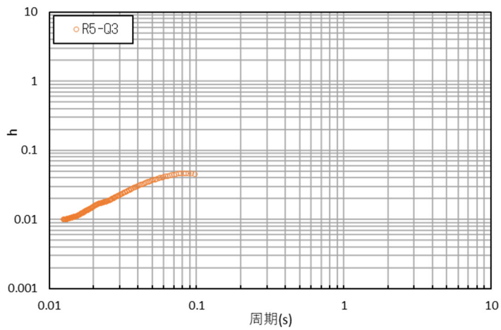
参考 1-3-18 図 コリレーション波形と減衰定数 (R5-Q3 孔: 観測深度 GL-18m~-130m)
