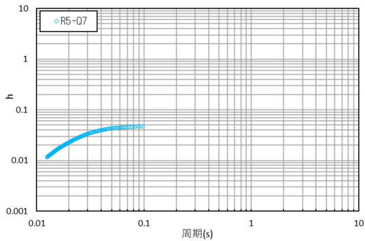
参考 1-3-22 図 コリレーション波形と減衰定数 (R5-Q7 孔: 観測深度 GL-18m~-130m)
