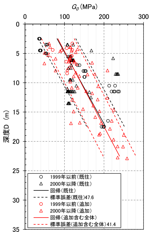
第 3.4-2 図 G_0 分布(全 30 孔)
